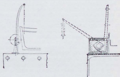
Шлюпбалки поворотные и сист. Welin.
