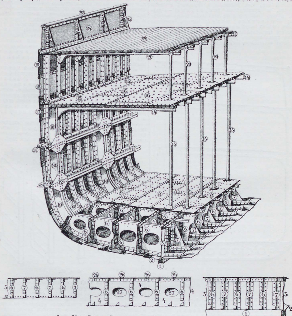
Фиг. 38а. Стальной корпус с двойным дном.
