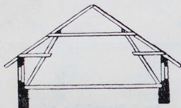
Рис. 9. Пролет 10,5 м.
