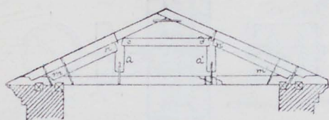
Рис. 4. Пролет от 13 до 15 м.
