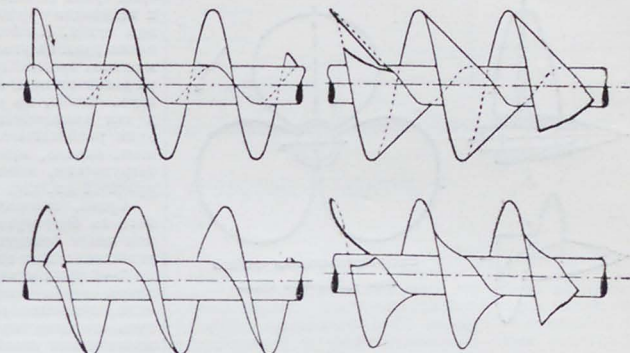
ВИНТОВЫЕ ПОВЕРХНОСТИ РАЗЛИЧНОГО ВИДА.
