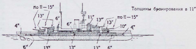
Линейный корабль „Royal Sovereign“
