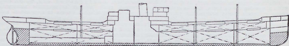
РАСПОЛОЖЕНИЕ ГРУЗОВЫХ ТРЮМОВ.
