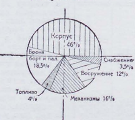
4. Большой легкий крейсер «Courageous» 1916 г.
