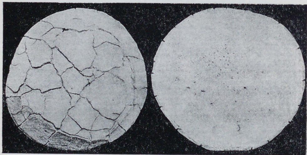
Лепешка, обнаруживающая так называемое «непостоянство объема» цемента. На рис. видны характерные трещины. Лепешка же вполне доброткацементного цемента — совершенно гладкая и прочная.
