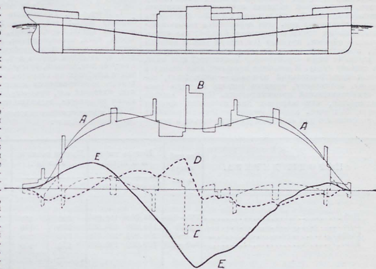
ПРОДОЛЬНАЯ КРЕПОСТЬ НА ПОДШВЕ ВАРНЫ.
