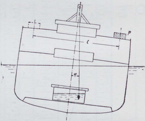
Определение центра тяжести судна путем наклонения
