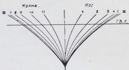
Масштаб Бонжана.
