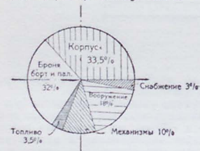
1. Лин. кор. «Royal Sovereign» 1915 г.
