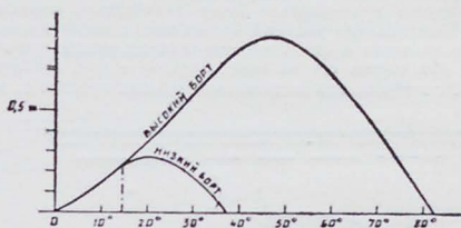
Зависимость остойчивости от высоты борта.
