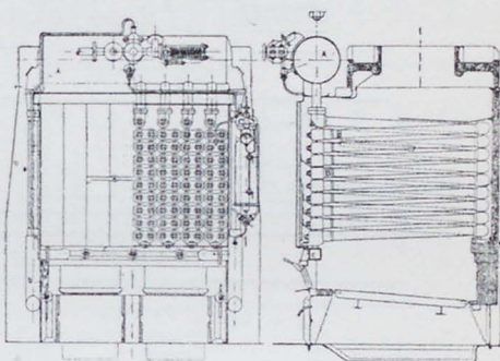
Судовой водотрубный котел Бельвиля.
