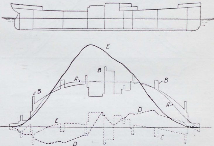
ПРОДОЛЬНАЯ КРЕПОСТЬ НА ТИХОЙ ВОДЕ.
