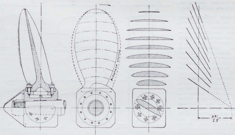
ГРЕБНОЙ ВИНТ ТОВАРО-ПАССАЖИРСКОГО ПАРОХОДА.
