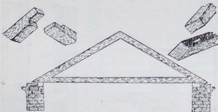
Рис. 1. Пролет до 6,5 м.
