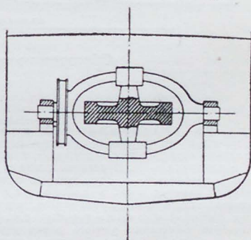
Жироскоп Шлика.
