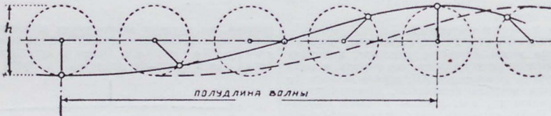
Образование профиля волны по трохоиде.
