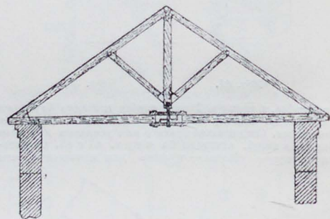
Рис. 3. Пролет от 8,5 до 10,5 м.
