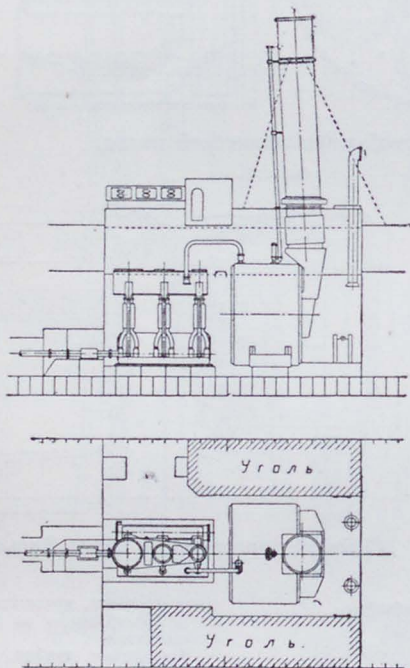
Расположение главных механизмов
