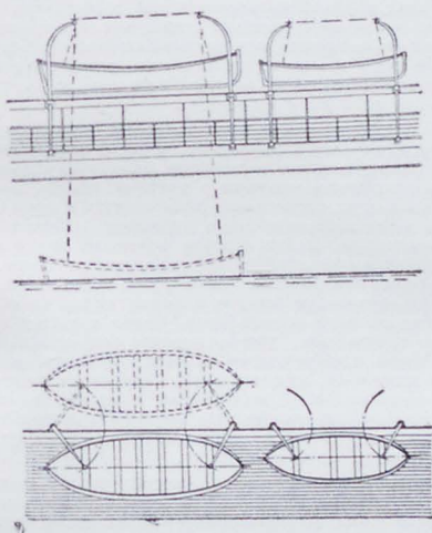
Шлюпбалки поворотные и сист. Welin.
