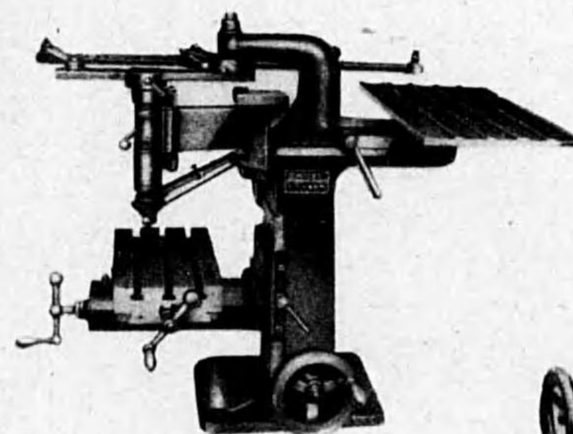
DO型彫刻機
