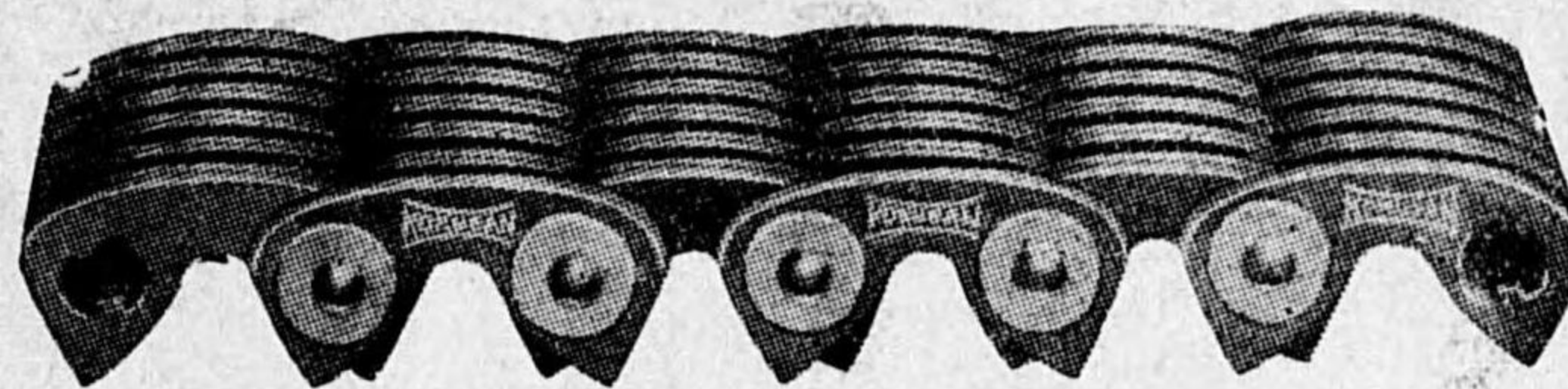
高速度サイレントライナーチェーン
