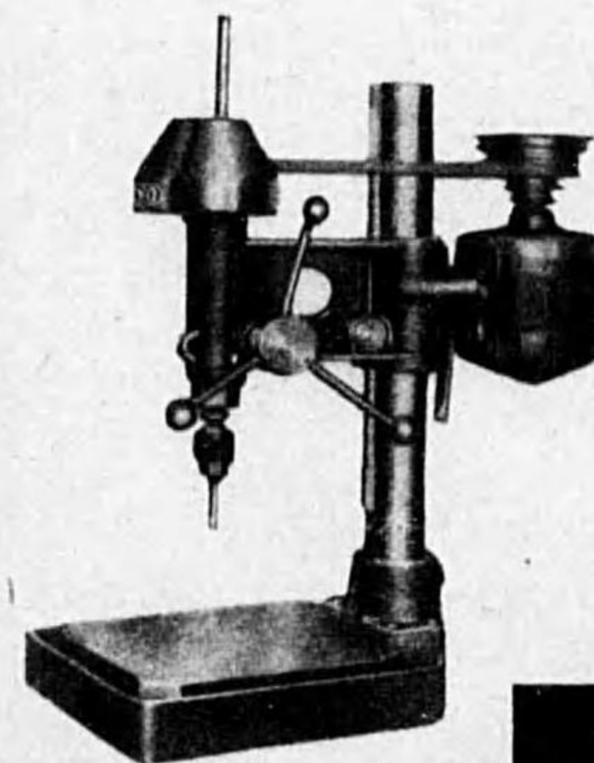
M.D.型高速電動 卓上鑽孔機
