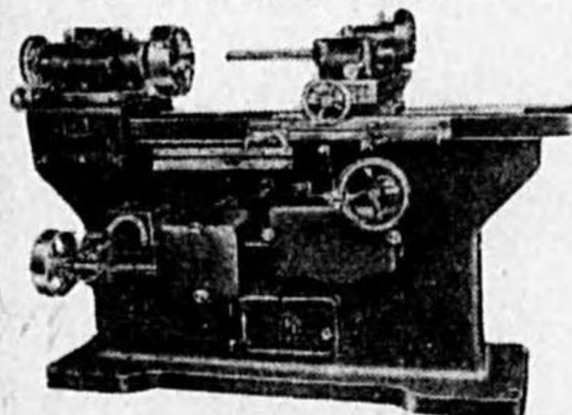
3H型内面研磨機
