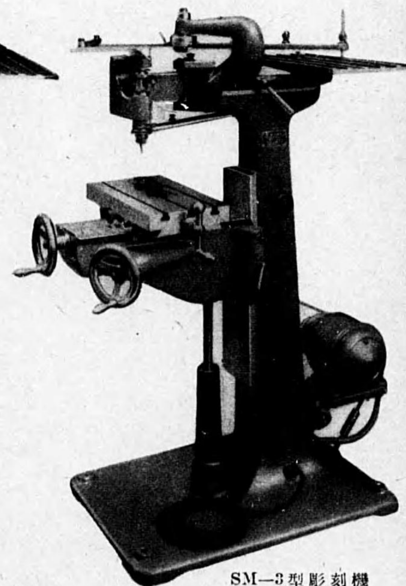
SM-3型彫刻機
