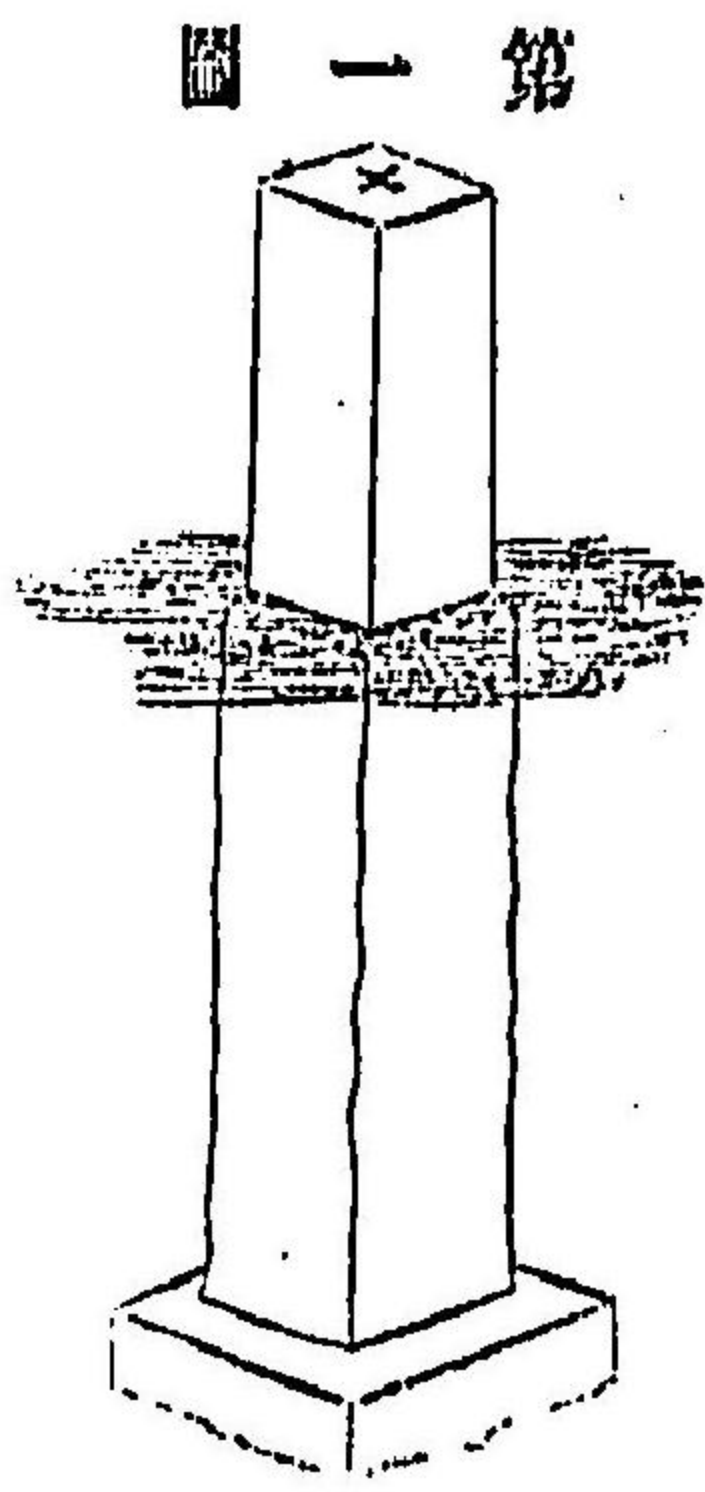
第一圖 標材ハ堅實ノ石ヲ用ユ方柱ニシテ幅約五六寸 標面上ニ顯ナルコト約一尺五寸餘ハ土中ニ 埋ム表面ニ經度或ハ緯度測點點面ニハ水路 部標面ニハ年月日ヲ刻ス
