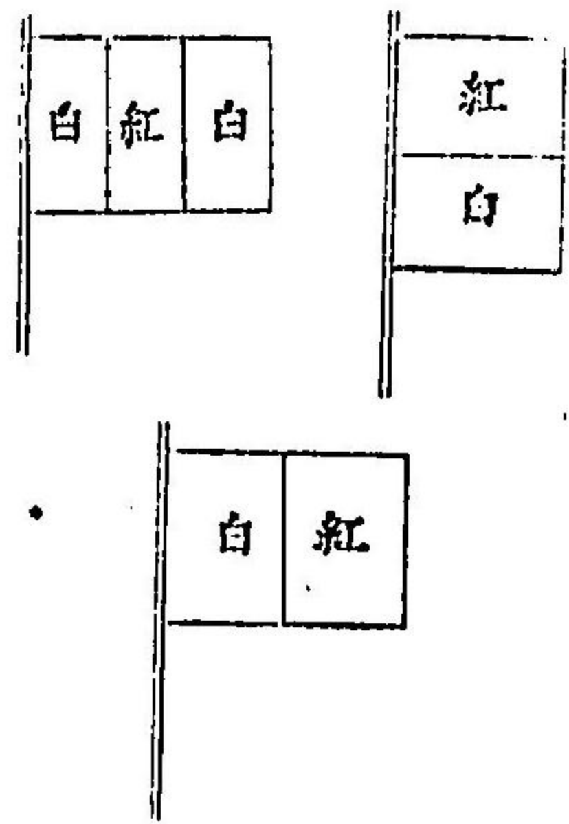
第二圖 紅白二色ノ金印ヲ用ユ其大サハ測量ノ難易ニ照シテ各大小アリ竿ハ竹杭ハ木片片面ニ水路測點ト書ス或ハ傍側ニ木標ヲ 添設シテ之レニ書スルコトアルヘシ 張綱ハ標樁ヲ用ユ場合ニヨリ麻若クハ鐵繩ヲ用ユルコトアルヘシ
