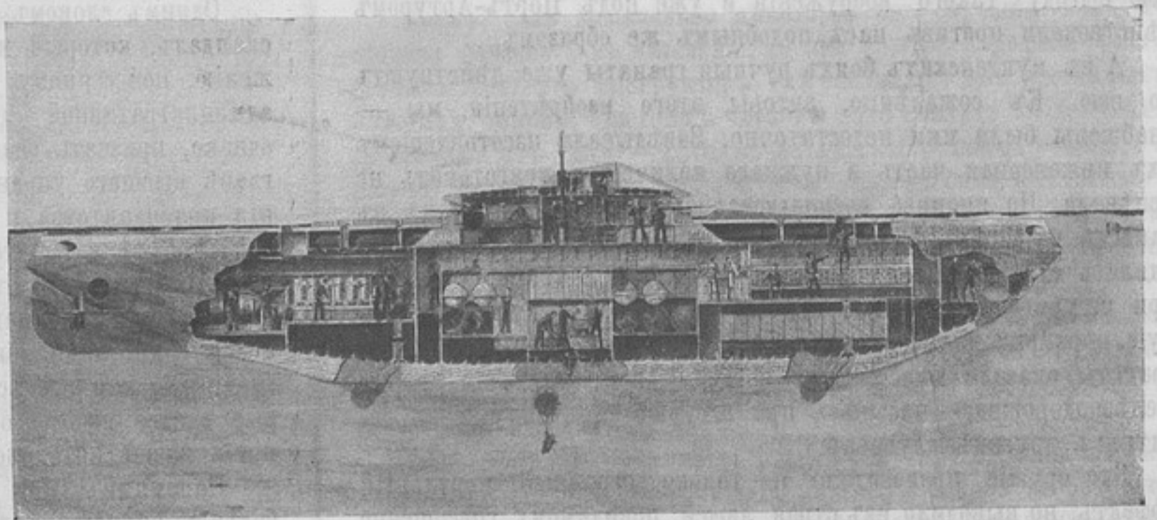
Лодка типа Лэка, въ разрѣзѣ. Въ средней части показано, какъ лодка ставитъ мины загражденія (Изъ книги «Нуженъ ли намъ флотъ и значеніе его въ исторіи Россіи»).
