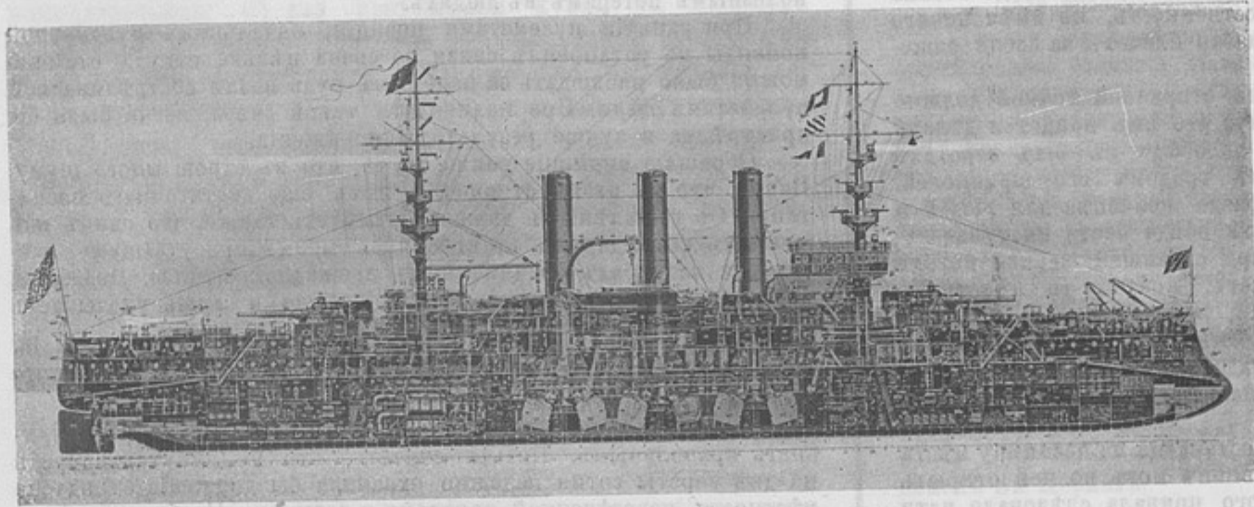
Внутреннее расположеніе современнаго броненосца. (Изъ книги «Нуженъ ли намъ флотъ и значеніе его въ исторіи Россіи»).
