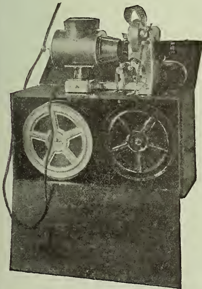
Fig. 4. Proyector portátil.
