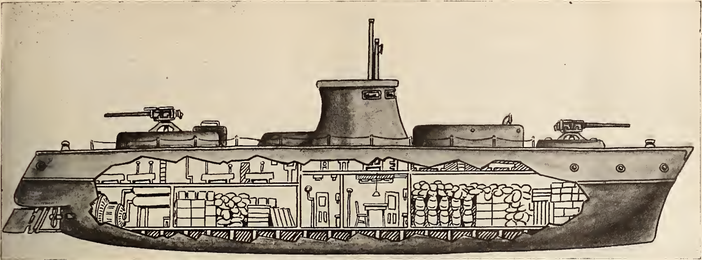
Buque de muy poco calado, de 1000 toneladas, destinado a burlar submarinos. Dibujo GAUMONT.
