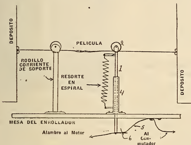
Un Interruptor de Motor.
