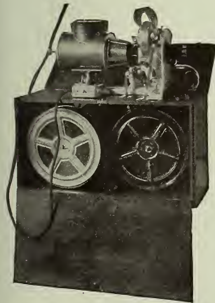
Fig. 4. Proyector portátil.
