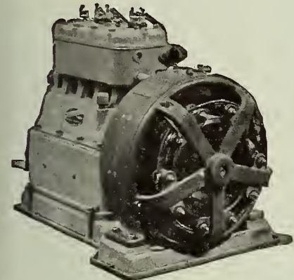
Fig. 1. Planta eléctrica a gasolina "Hallberg," 4 1/2 kilovatios.
