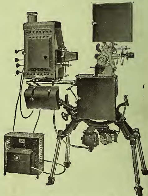
Camarógrafo de Power No. 6B
