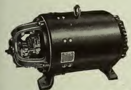
Fig. 2. Motor-generador "Hallberg 20th Century," para corriente alterna y continua.
