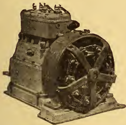
Fig. 1. Planta eléctrica a gasolina "Hallberg," 4 1/2 kilovatios.
