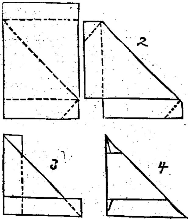
三 角 袋 摺 疊 順 序 (虛 線 為 摺 疊 處)
