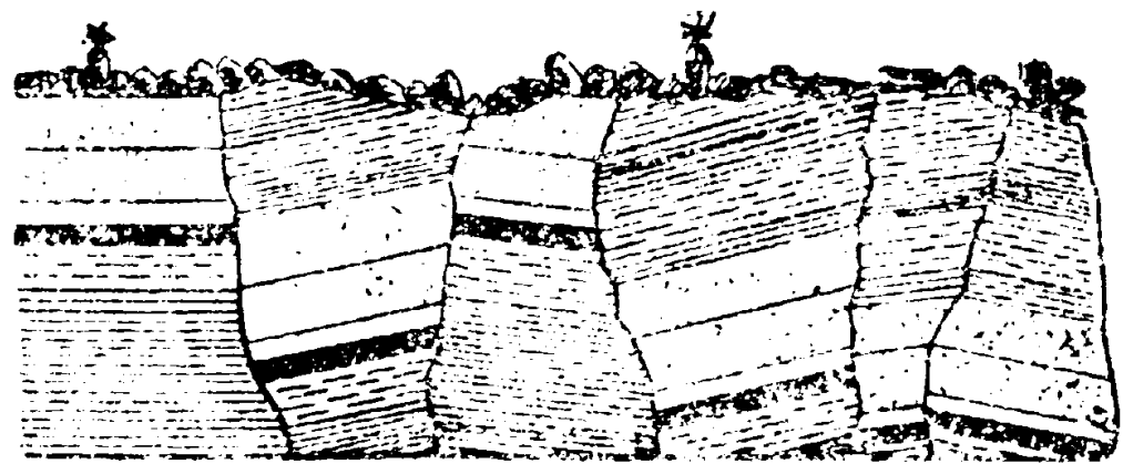
第72圖——斷層
