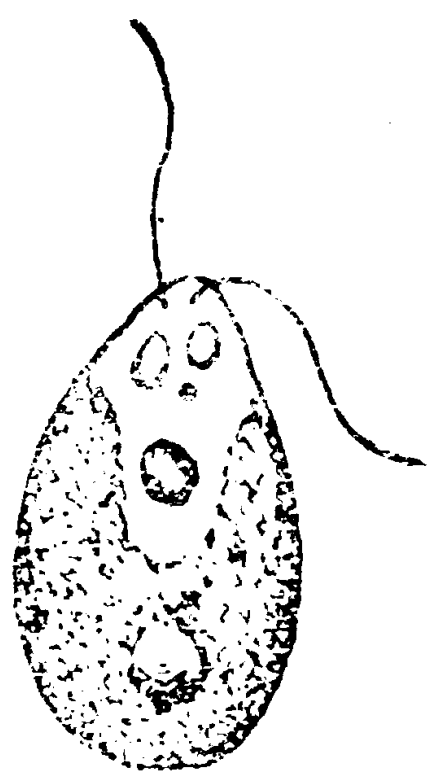
第25圖——單胞藻
