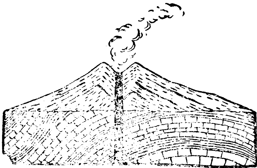
第73圖——火山
