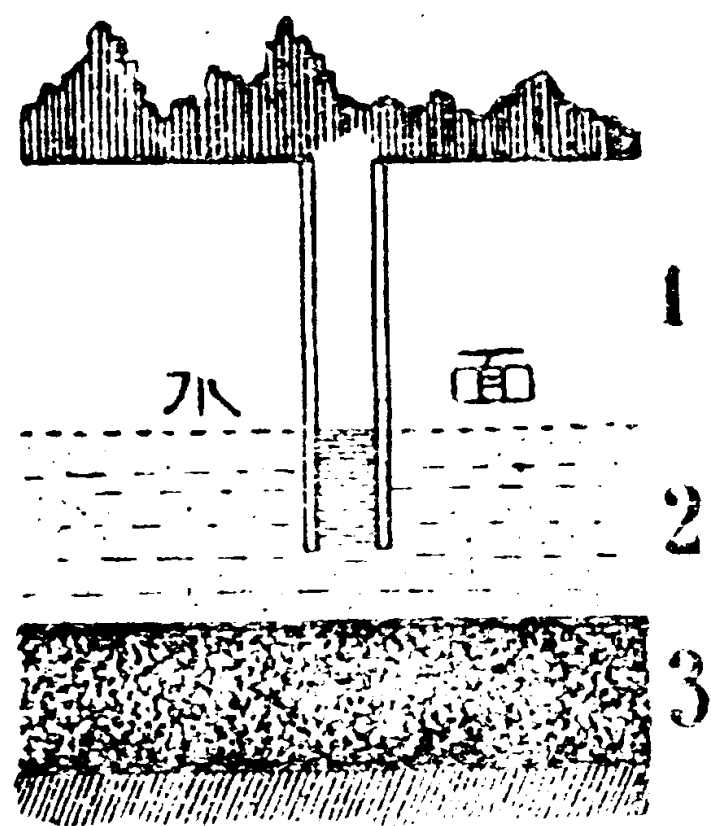
第64圖——井的發生 1,透水層；2,留水層；3,不透水層。
