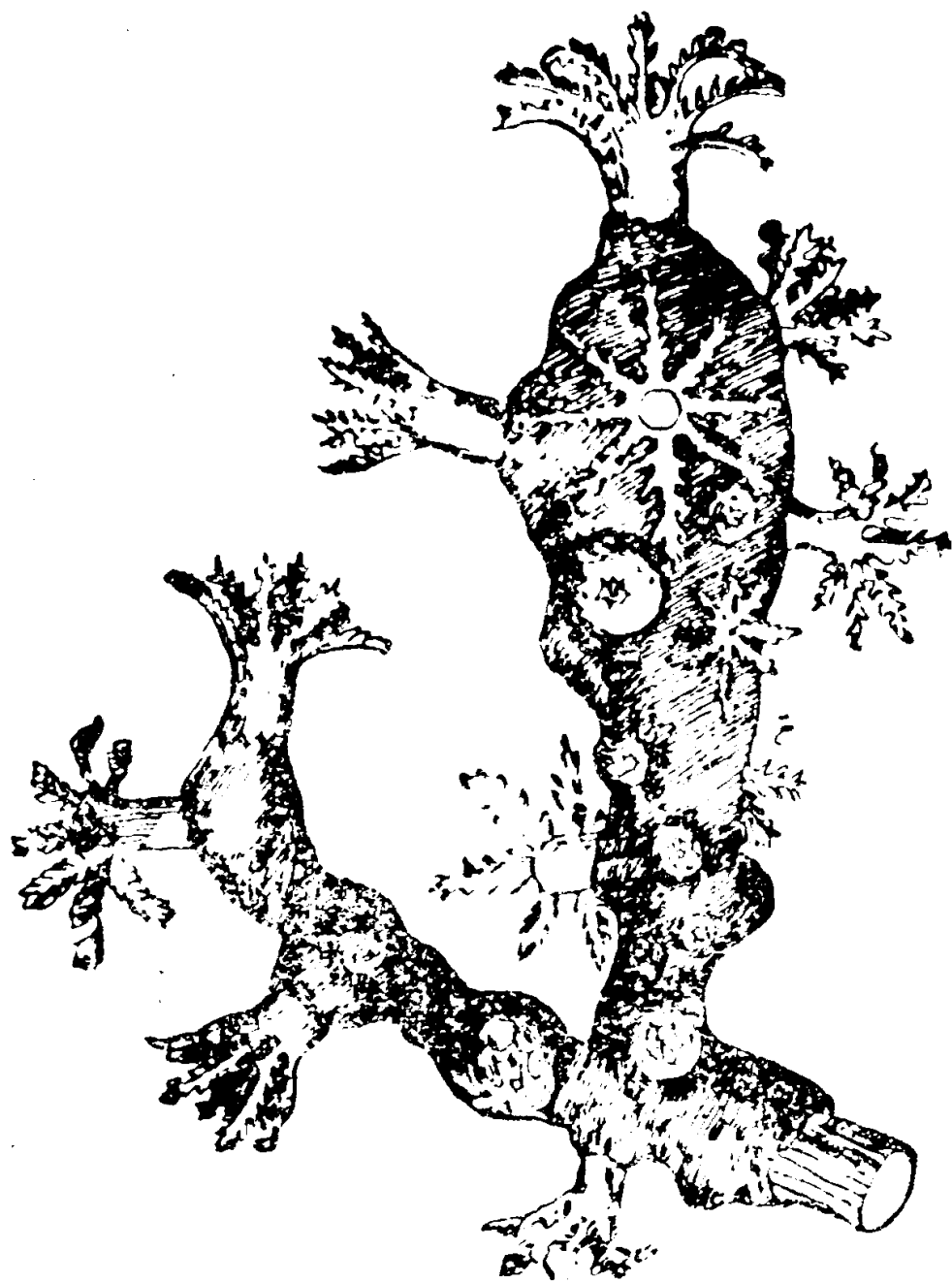
第30圖——珊瑚蟲
