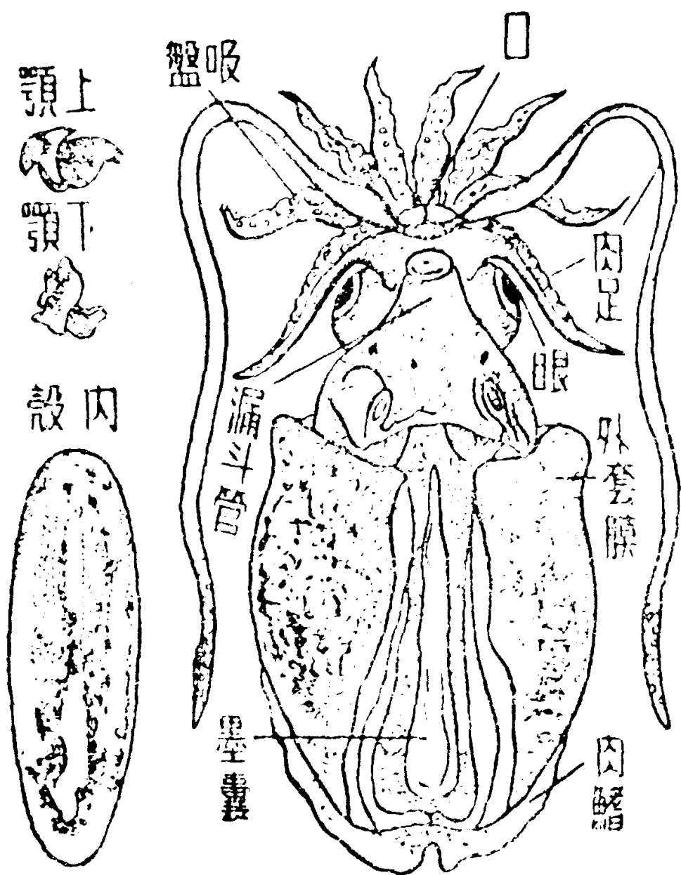
第40圖——烏賊
