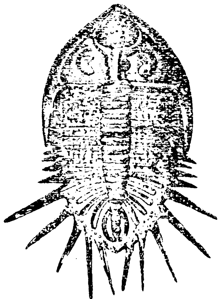
第77圖——三葉蟲
