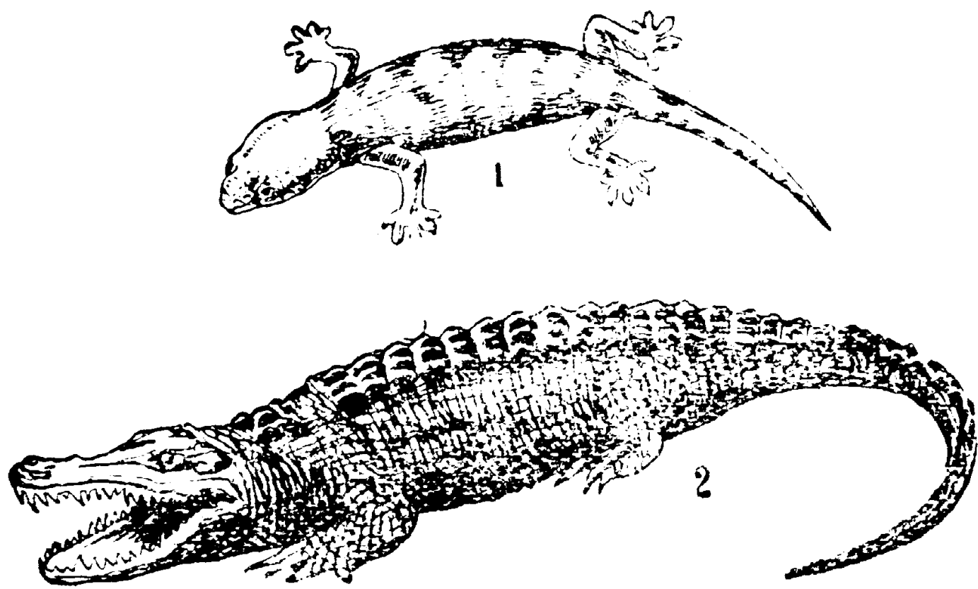
第53圖——1, 守宮；2, 鱷
