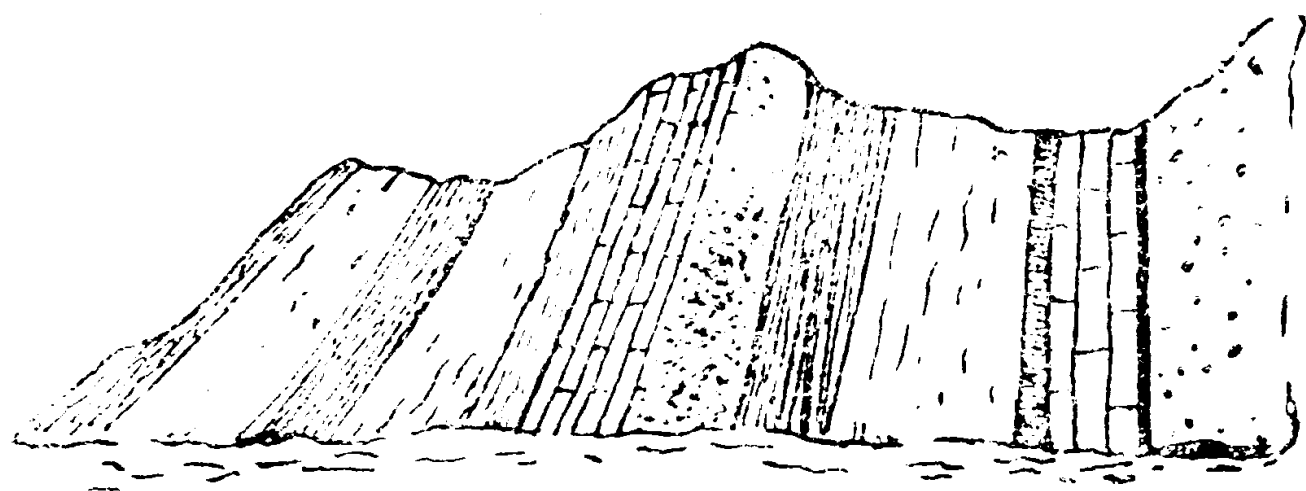
第74圖——直立層
