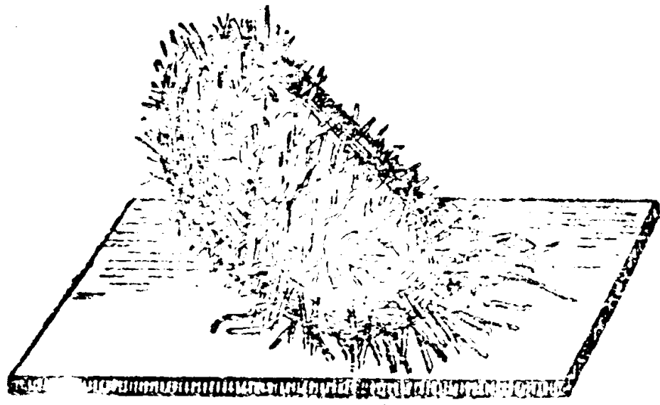
第33圖 一海 蜆
