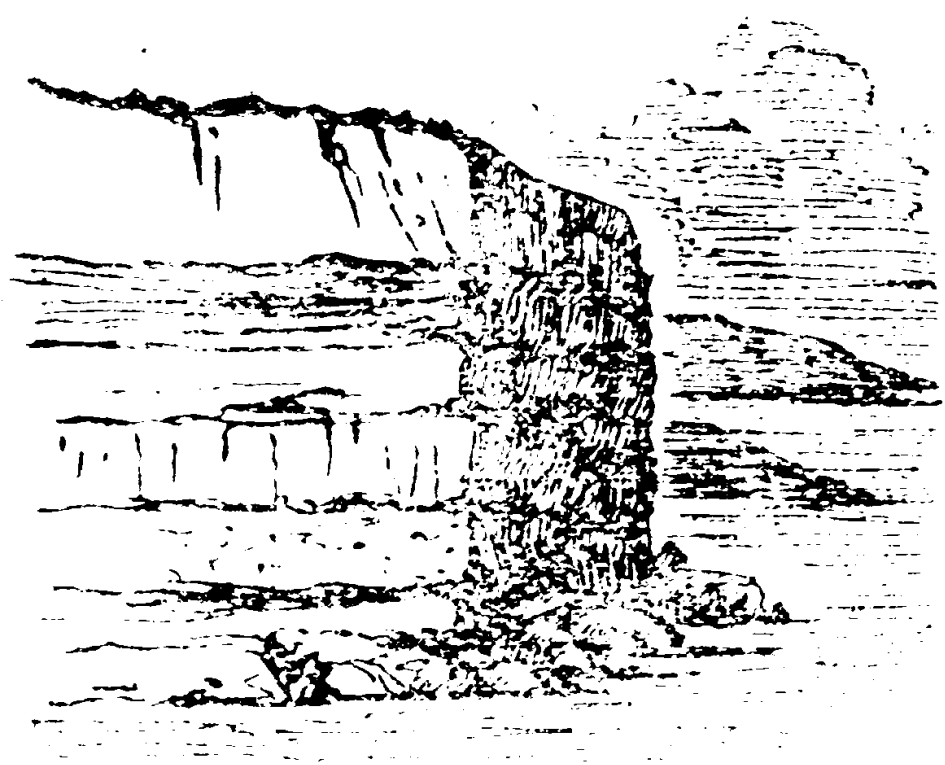
第71圖——水成岩層
