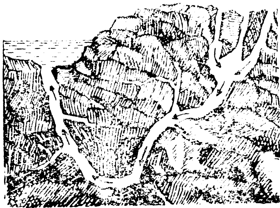
第66圖——溫泉
