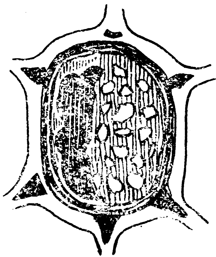
第13圖——篩管
