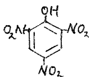
苦味酸
