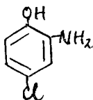
4-氯-2-氨基苯酚
