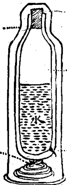
↑ 熱水瓶內部構造縱剖面略圖
