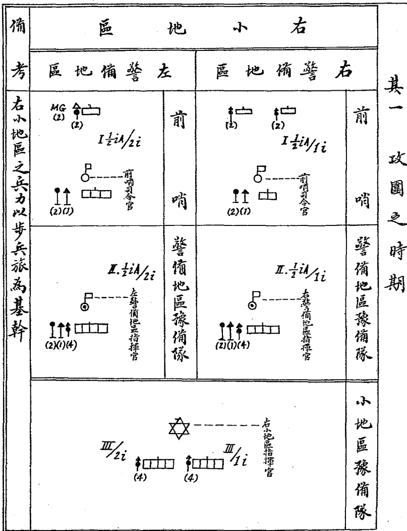
例圖之分區隊軍區地小內區地之師間業作擊攻並間圍攻時擊攻塞要於
