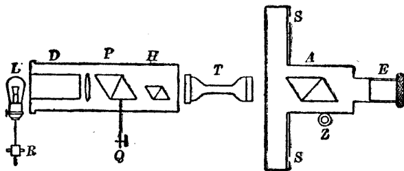
第 8 圖 偏極計之概略圖表(縱截面)
