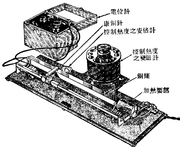
第 4 圖 丹諾斯之測熔點儀器
