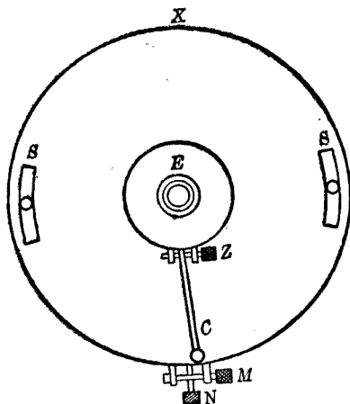
第 9 圖 偏極計(頂視圖)
