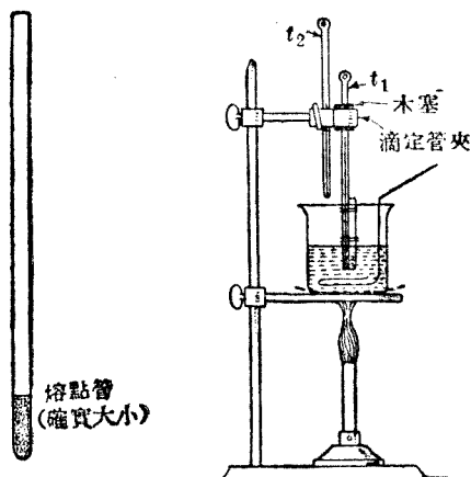
第 2 圖 測熔點儀器
