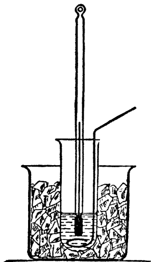
第 5 圖 簡單之測凝固點儀器
