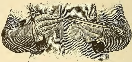
FIG. 20.—Diluting cultures.
