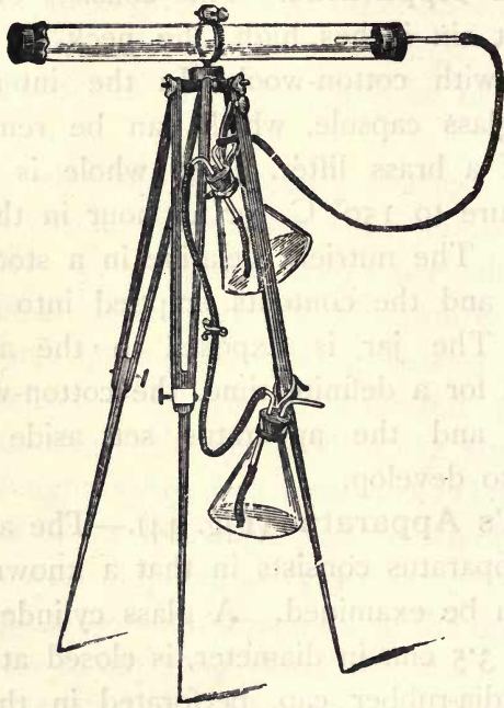
FIG. 44.—HESSE'S APPARATUS.
