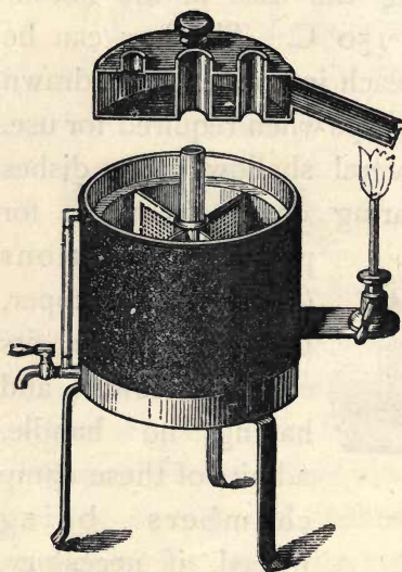
FIG. 14.—SERUM STERILISER.
