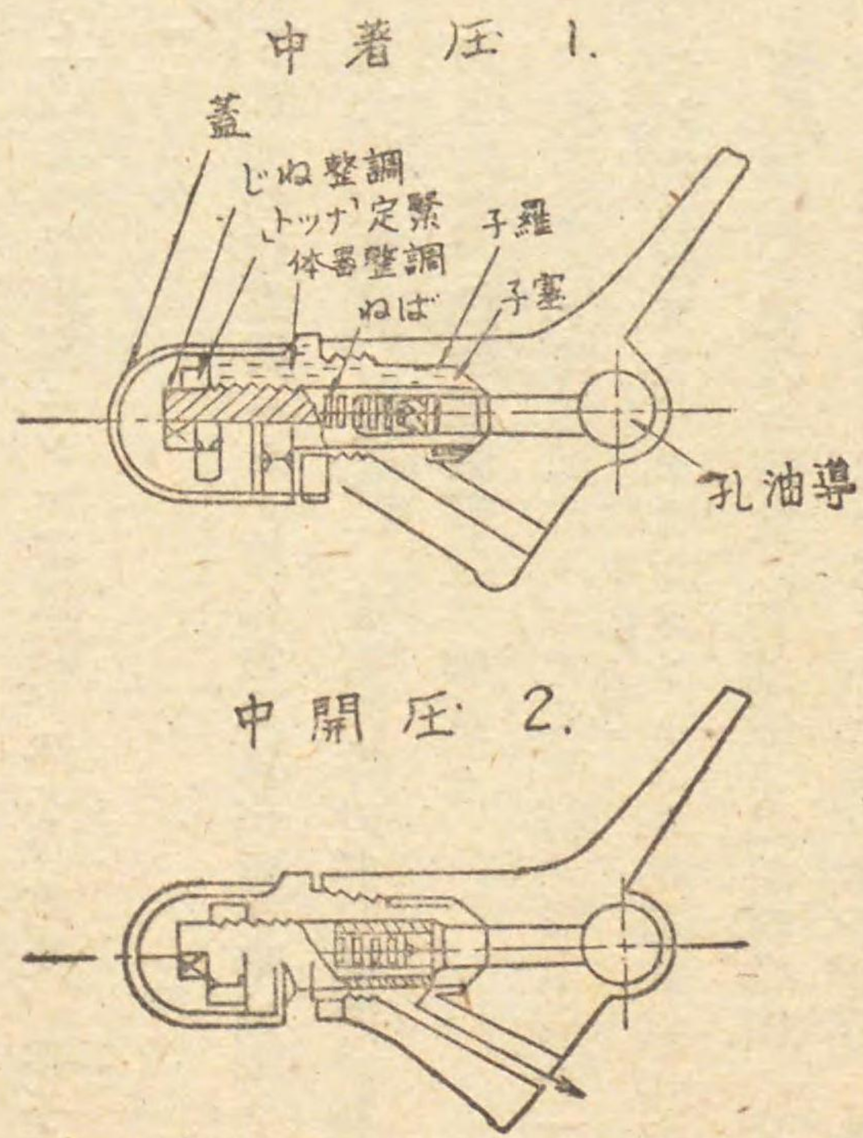
第百七十圖 油壓調整器
