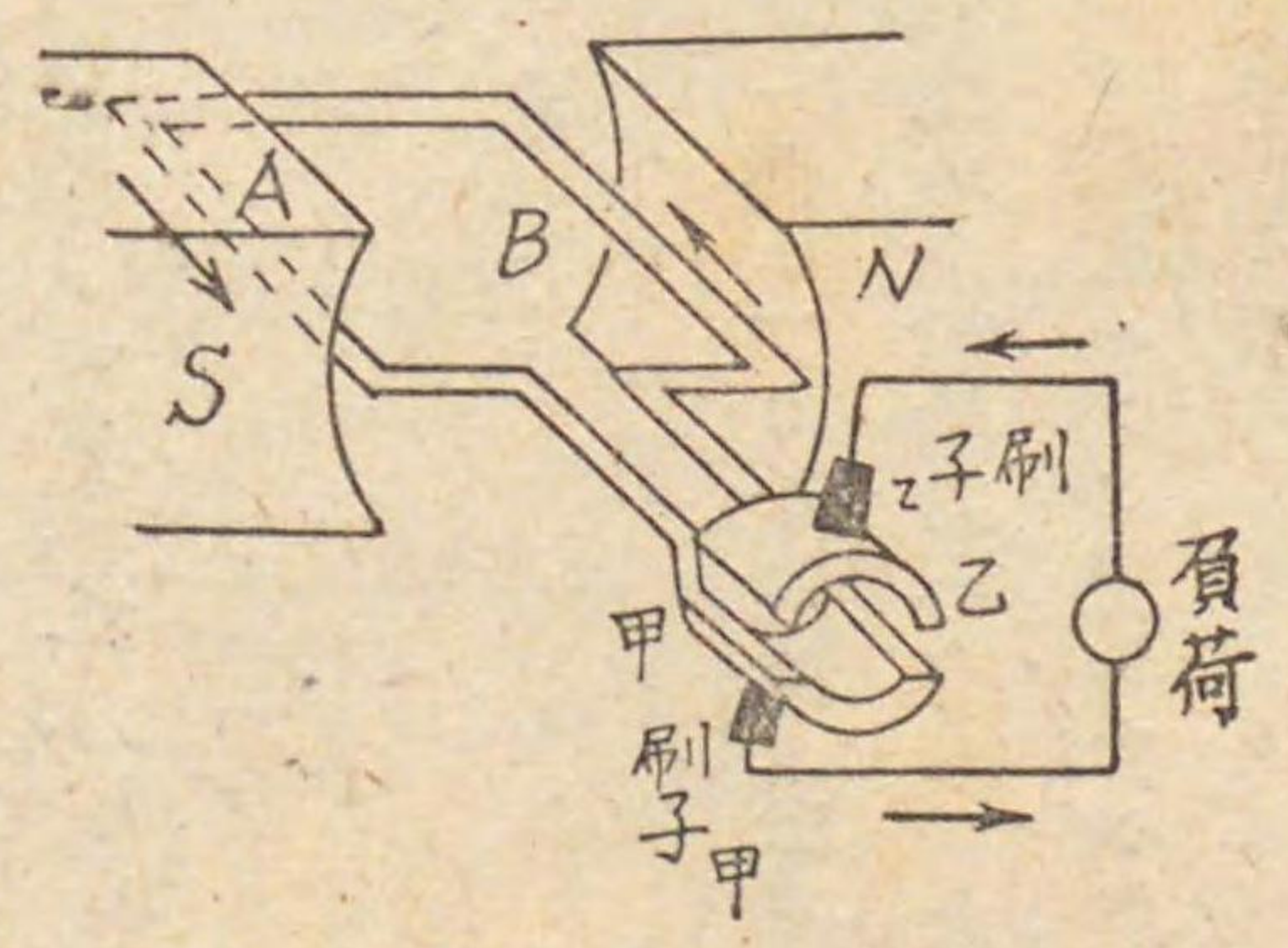
機電發流直 圖十九第
