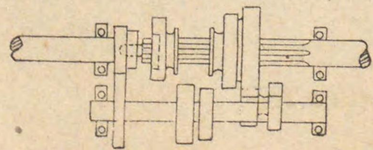
第一副齒車ト後退齒車大 後退齒車ト第一主齒車啞合
