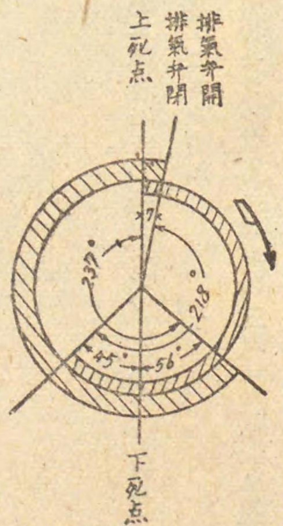
圖三十百第 弁調圖
