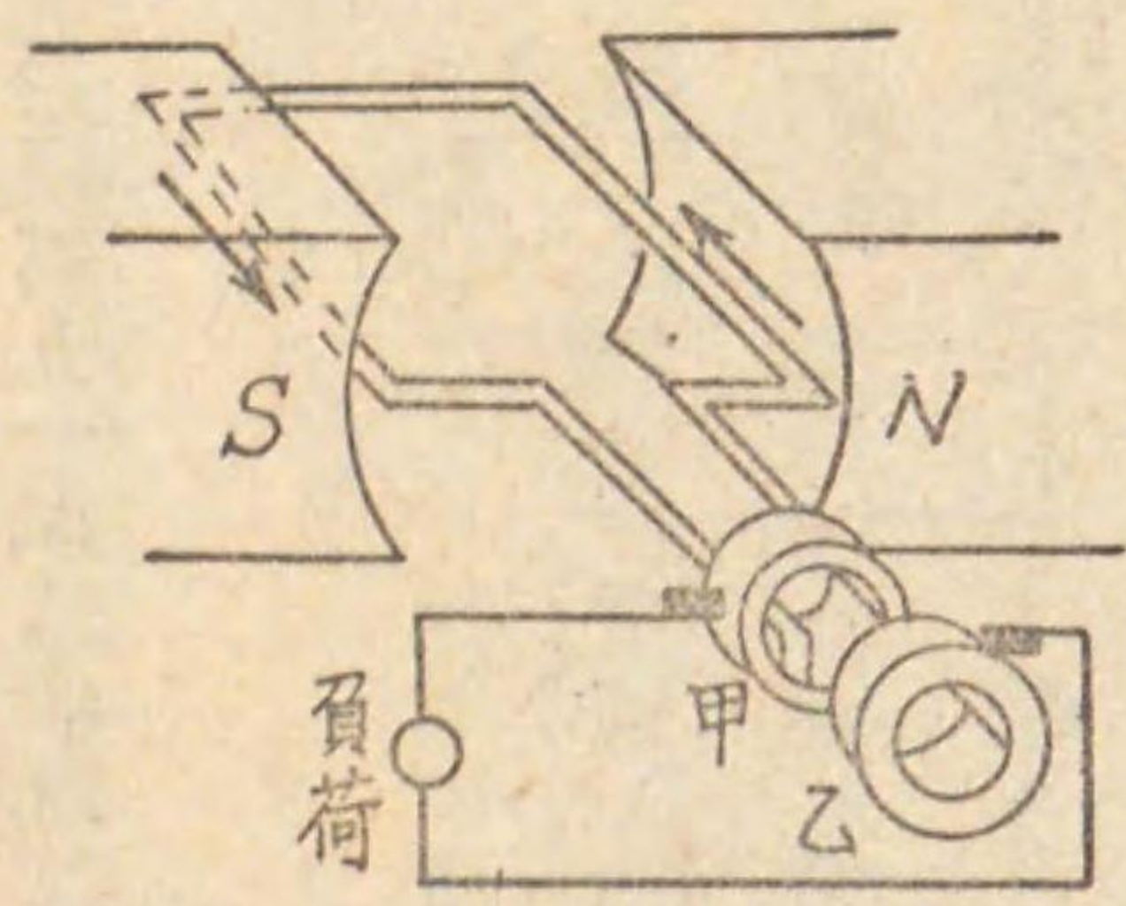
機電發卷直甲 圖二十九第
