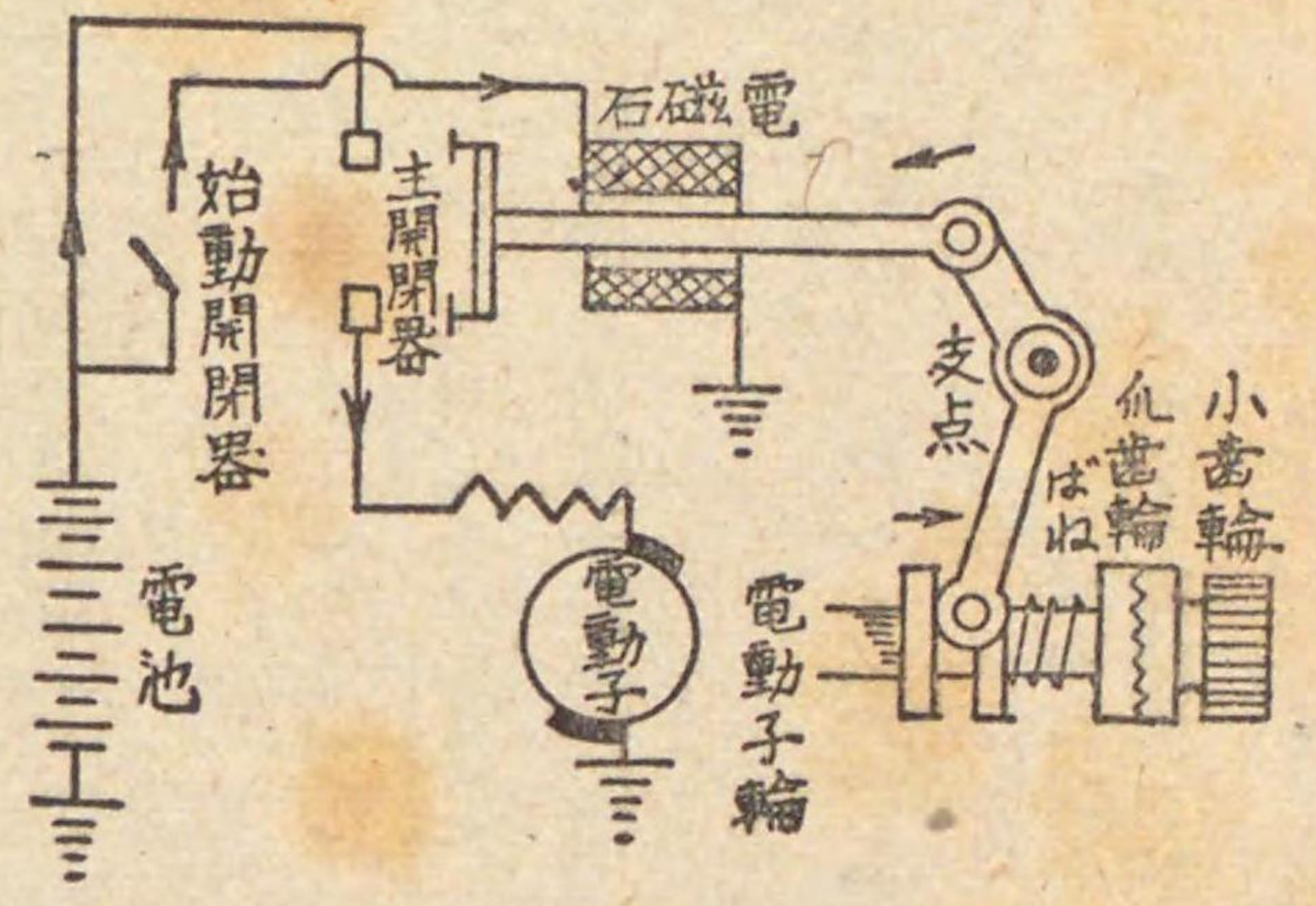
機動電動始式動自 圖五百第
