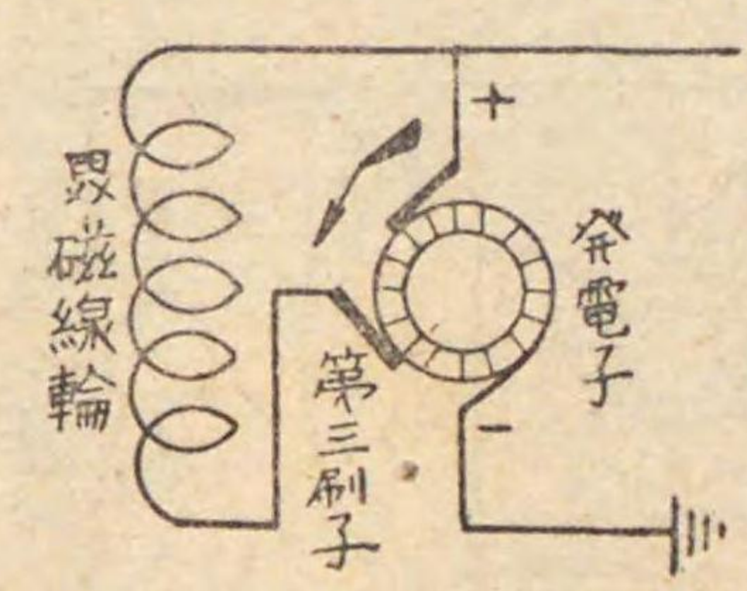
圖七十九第 機電發型子刷三第
