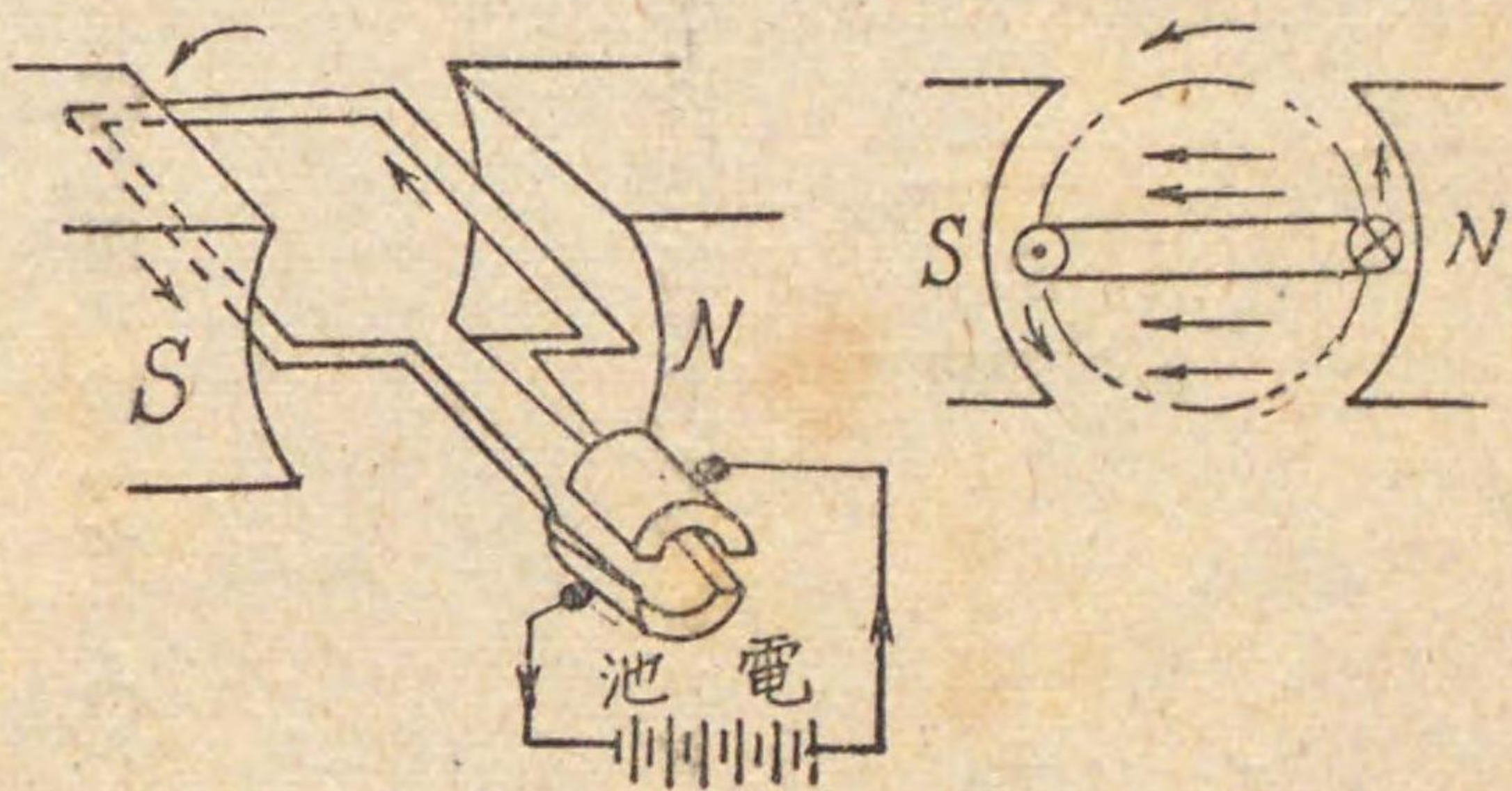
機動電流直 圖九十九第
