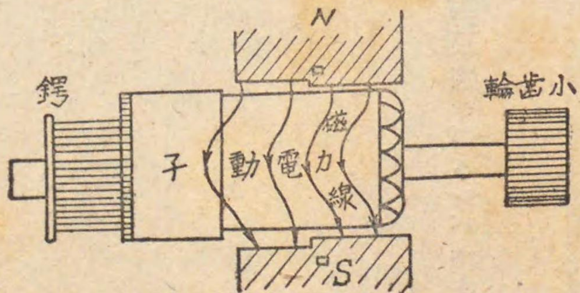
領要動移ノ子動電 圖三百第
