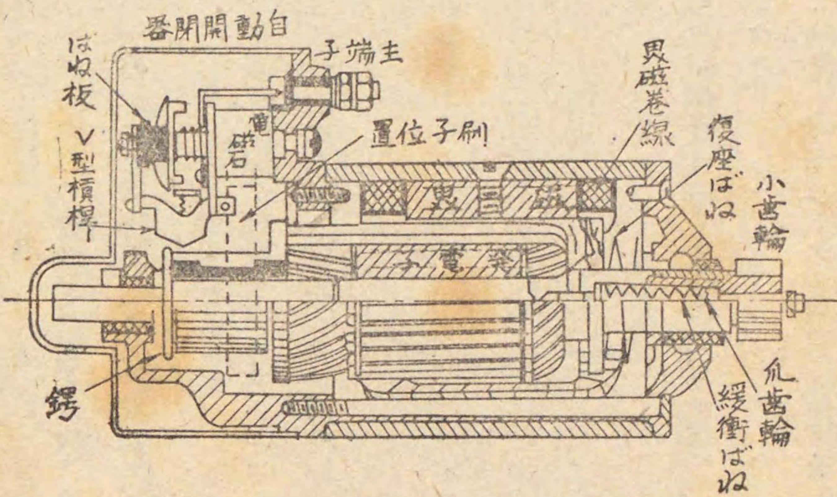
機動電動始型磁電 圖二百第
