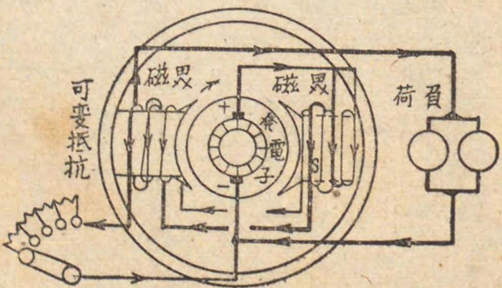
圖五十九第 複卷發電機
