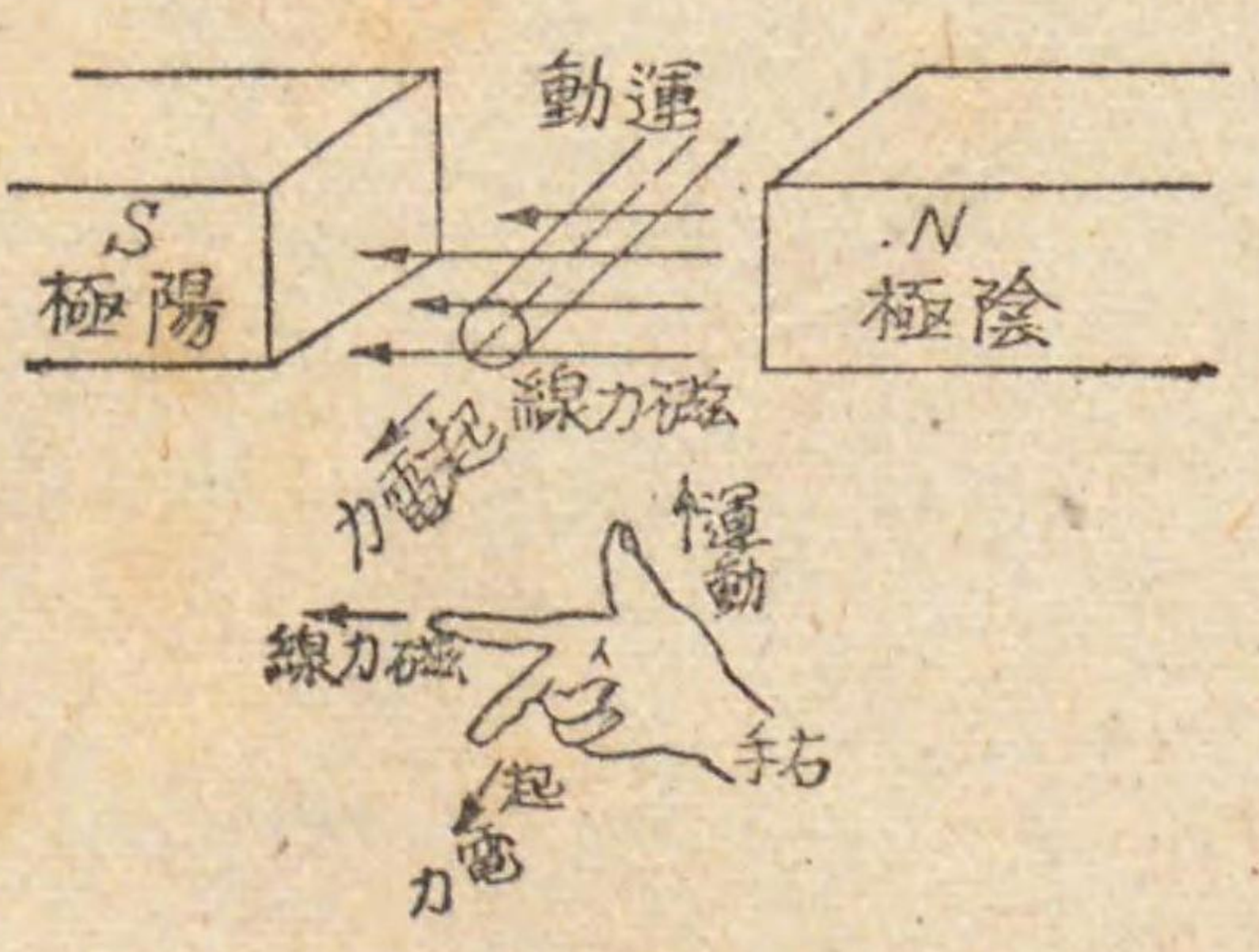
圖六十八第 則法ノ〔電發〕手右
