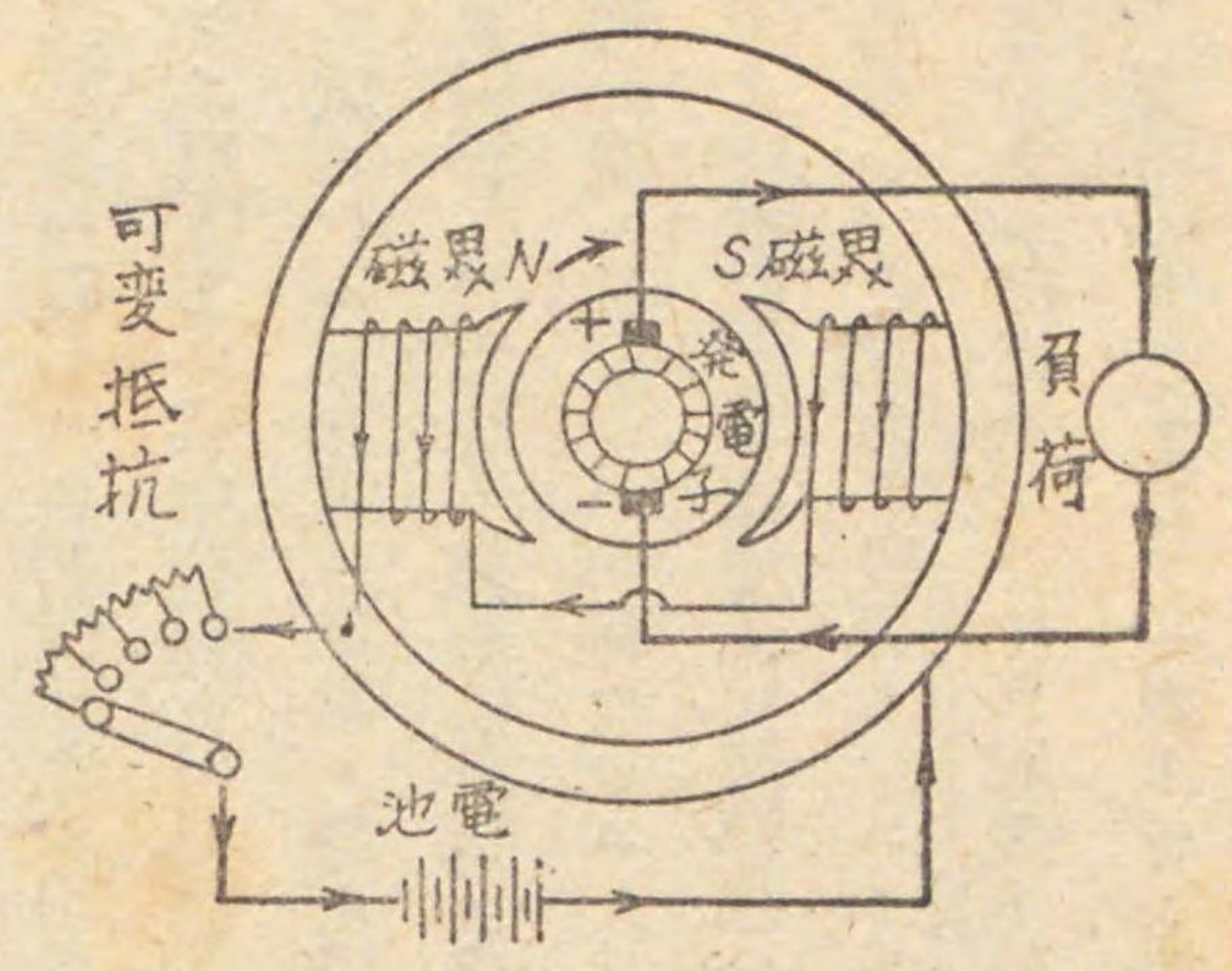
機電發磁動他極二 圖七十八第
