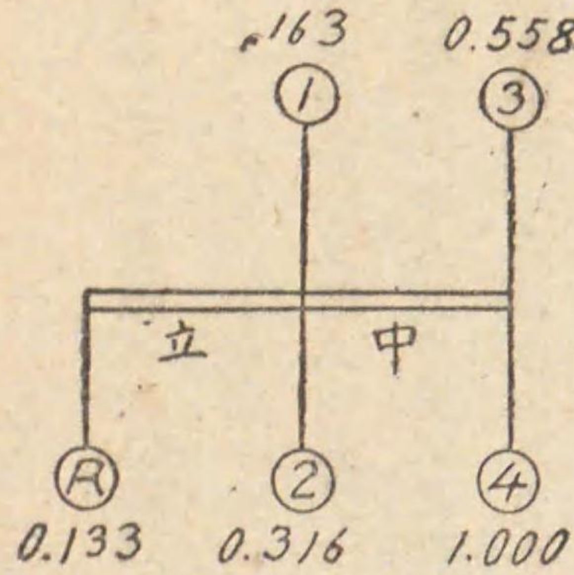
第一副齒車ト第一主齒車啞合
