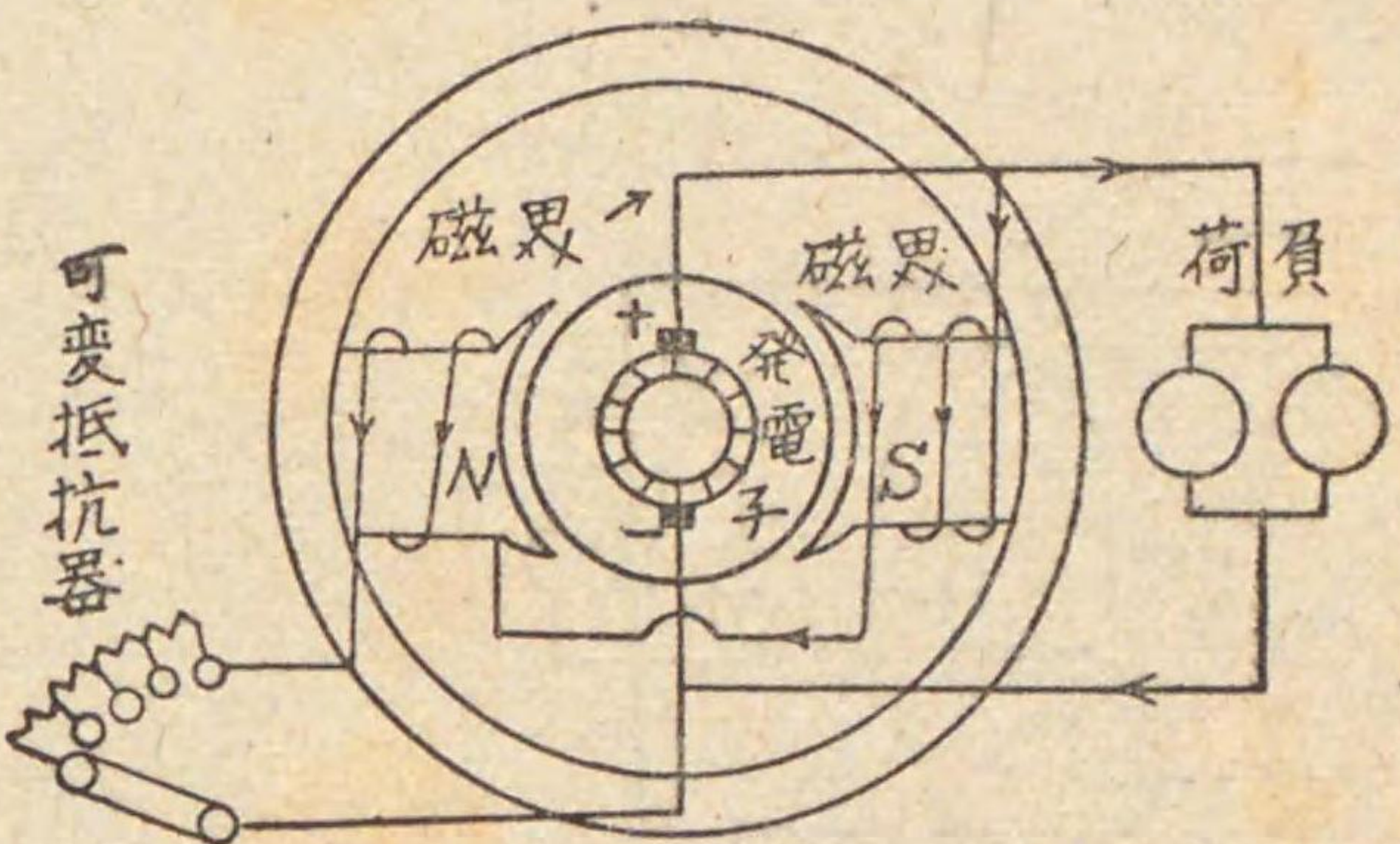
圖四十九第 分卷發電機
