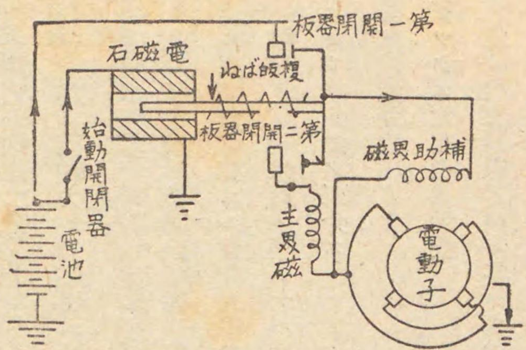
線配機動電動始 圖一百第
