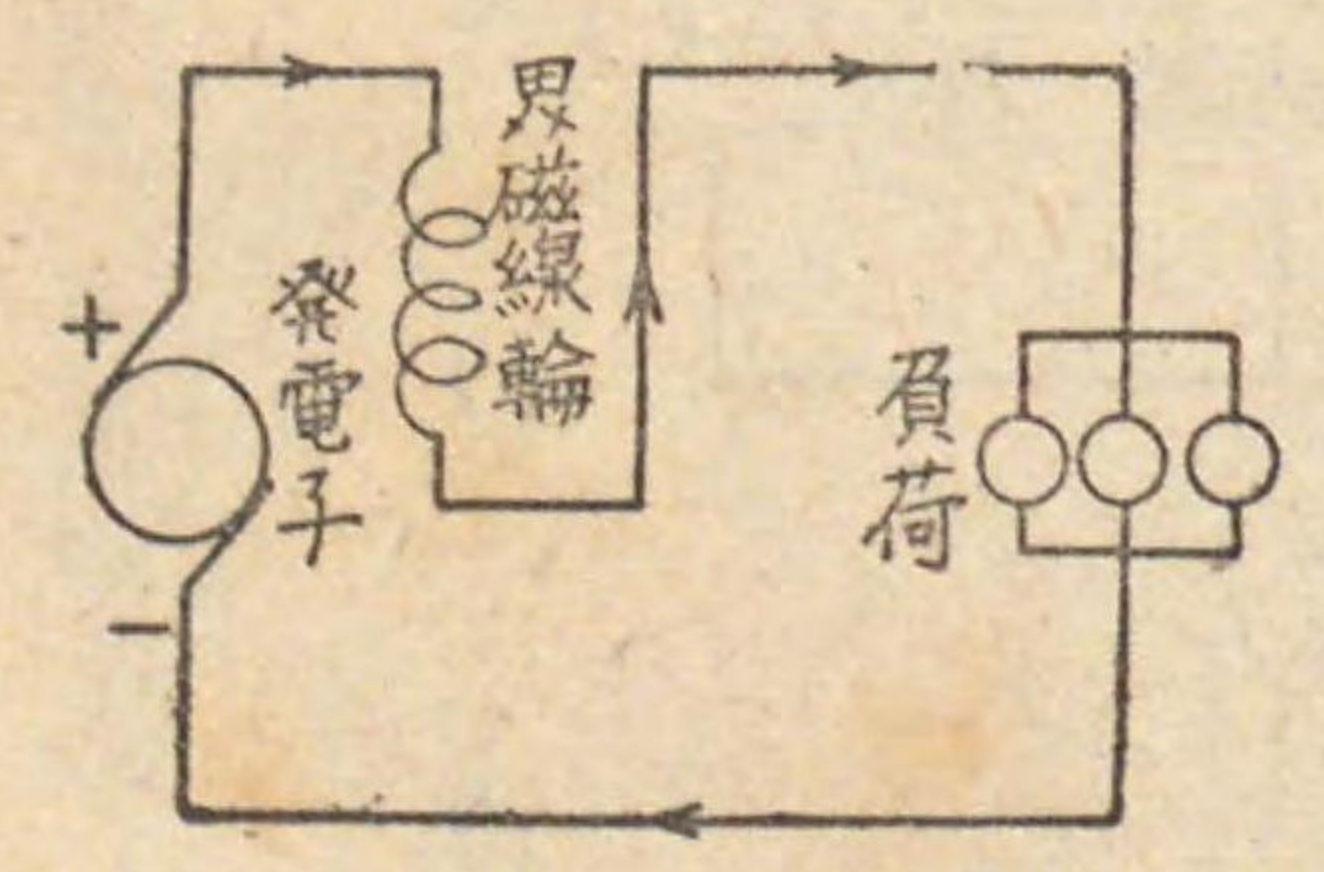
機電發卷直乙 圖二十九第
