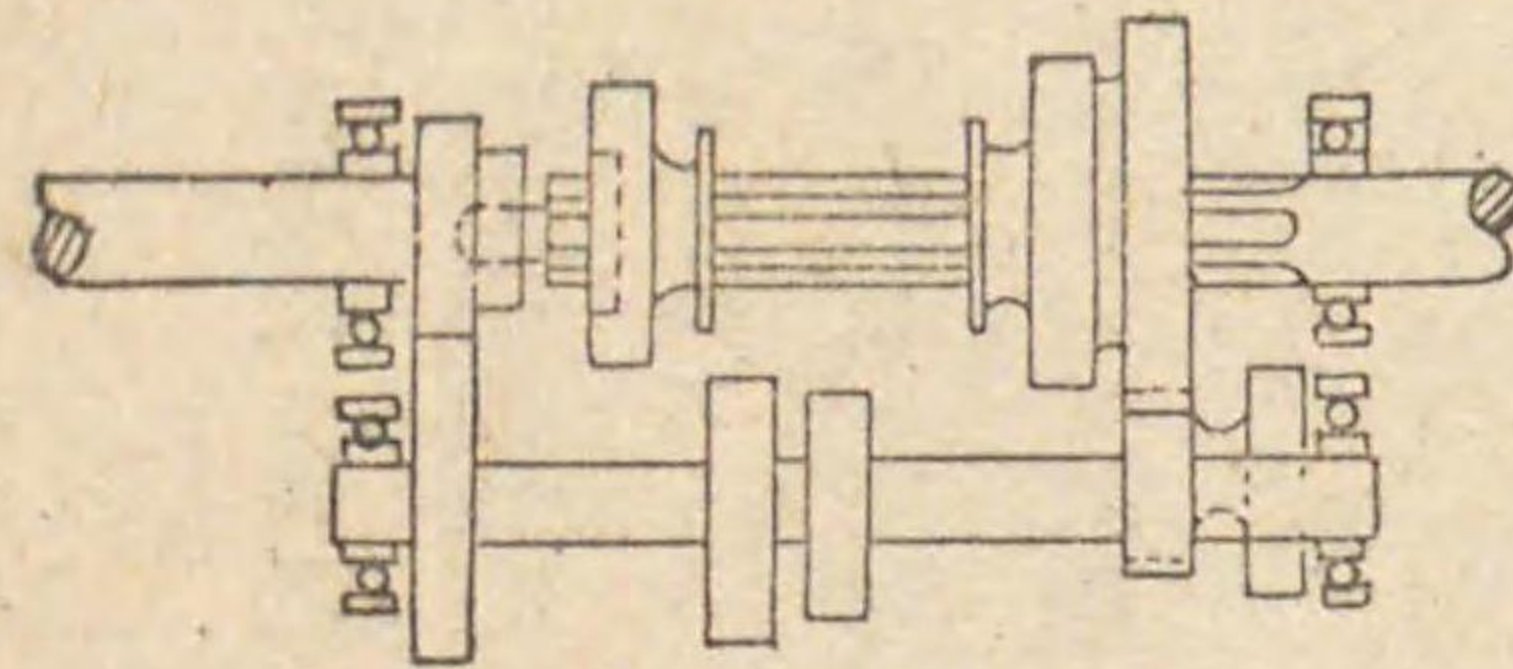
第三副齒車ト第三主齒車啞合
