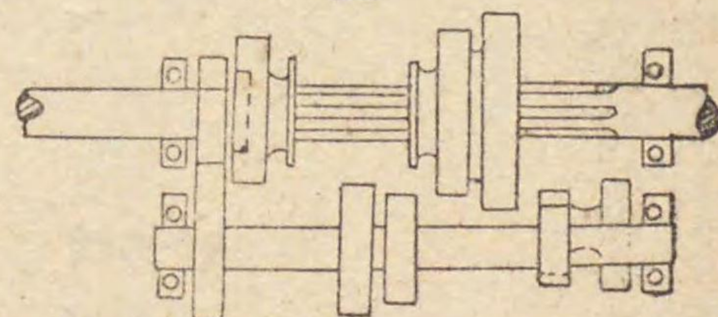
常啞主齒車ト直結
