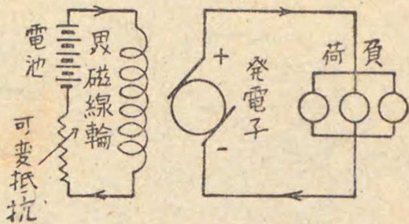
圖三十九第 他勵磁發電機
