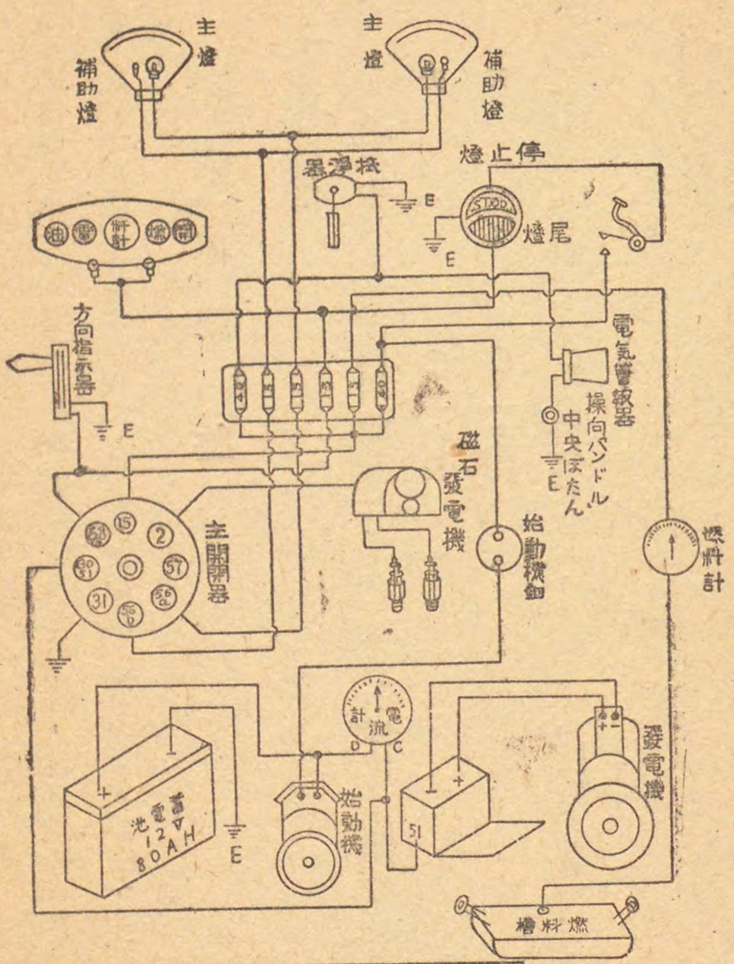
圖 線 配 圖 四 十 八 百 第
