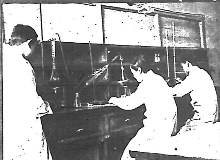
有機分析
