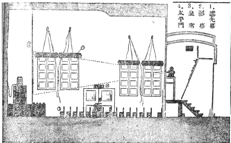
教育電影場之縱剖面圖 第十圖
