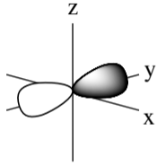
Orbitale p y
