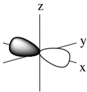
Orbitale p x
