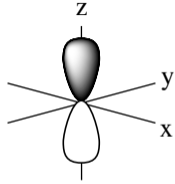
Orbitale p z
