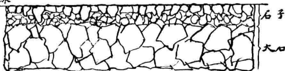
(23) 圖 碎石路剖面
