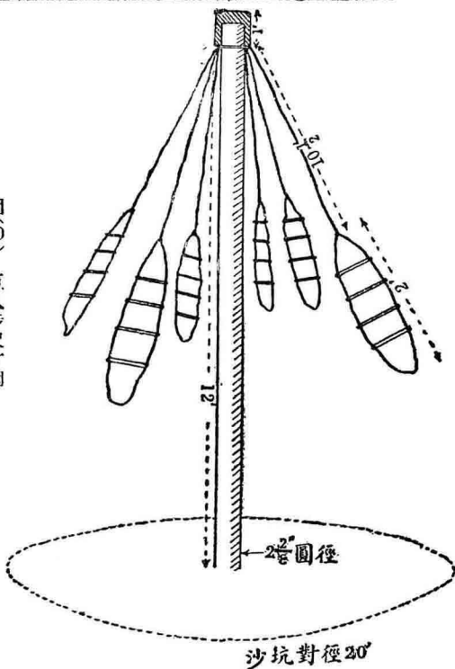
圖(40) 巨人步尺寸圖
