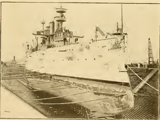
CRUISER "NEW YORK" IN DRY-DOCK. DER KREUZER "NEW YORK" IM TROCKENDOCK.
