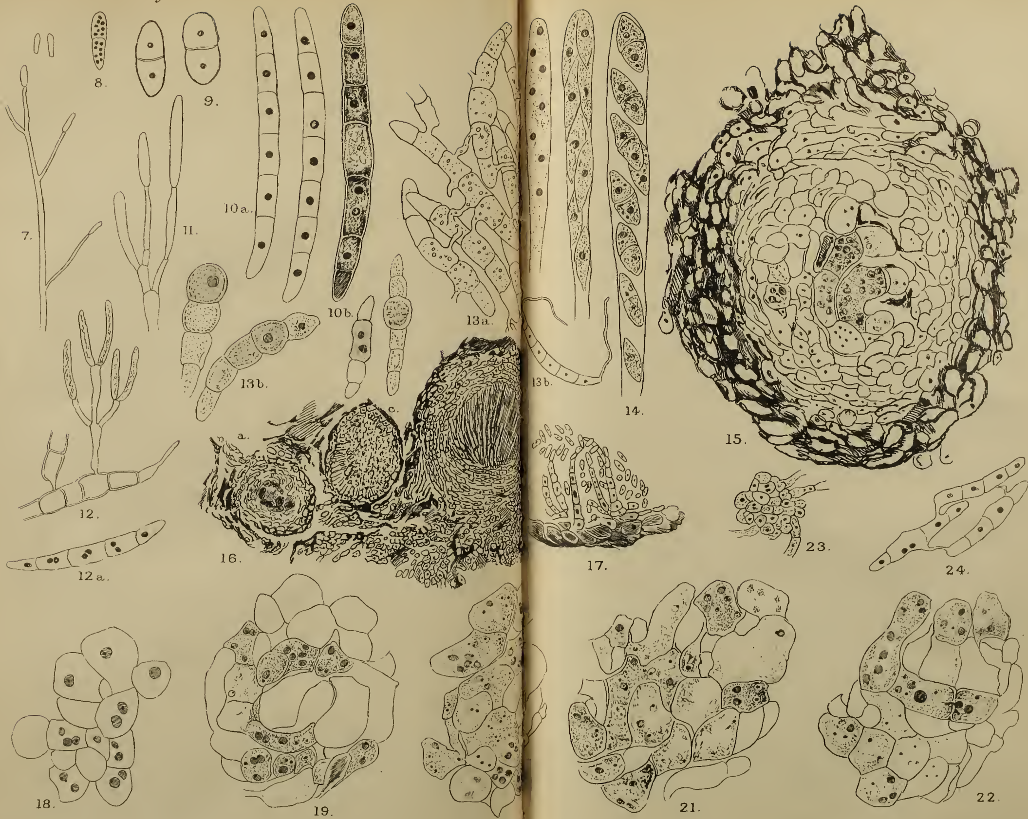
CAYLEY - NECTRIA GALLIGENA.
