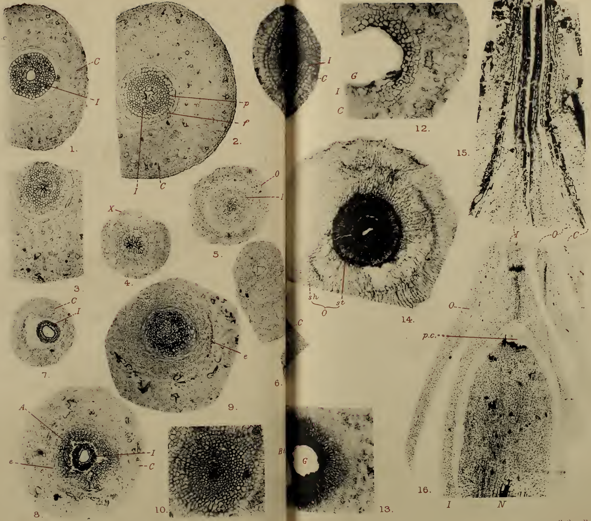
M. G. THODAY - GNETUM.
