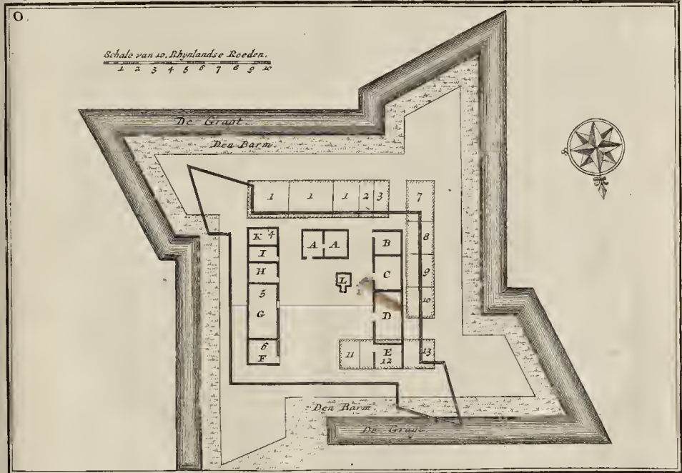
O. KAARTE VAN DE VESTING OP REMBANG, Gemeeten den 6. April 1708, door G. v. Broekhuysen.
