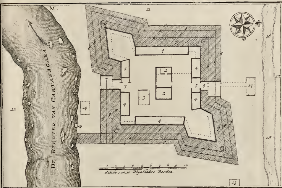
A. BEELDINGE VAN DE SCHANS GEMAAKT DOOR DEN E. CAPITEIN BINTANG, Tot CARTANAGARA, in de Land-streek van BANJOE-MAAS, Achter de Berg van TAGAL. na dat hy de laatste Slag tegen den Landlooper, Radin Parwata Sari, int Jaar 1706, heeft gedaan etc.
