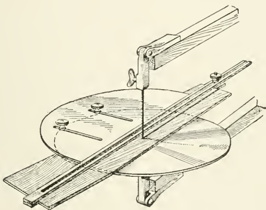
Fig. 54—Scroll-saw guide
