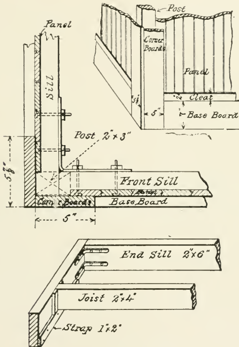
Fig. 312—Corner details
