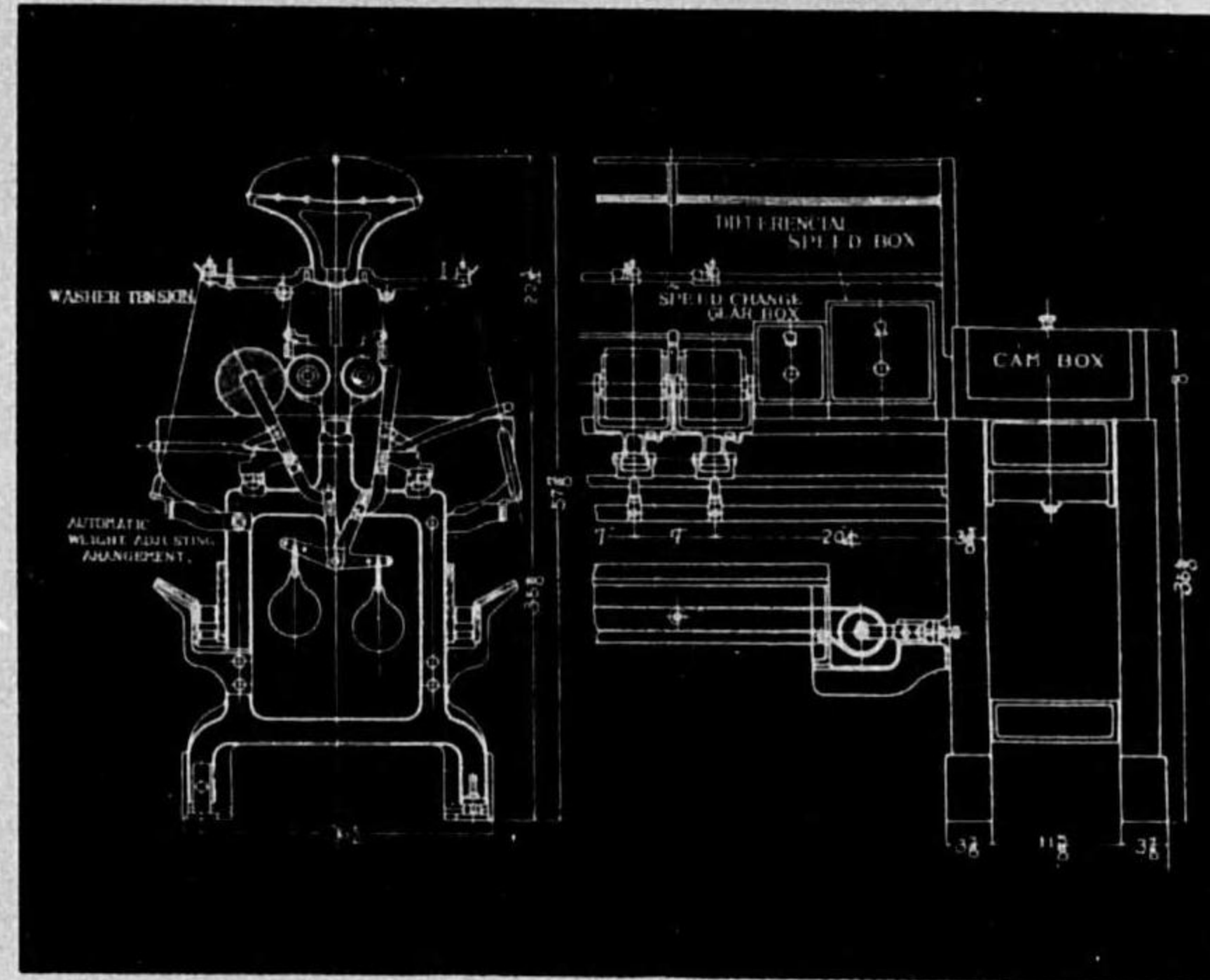
クイツク・トラバース・ワインダー セミハイスピード (特許出願中)
