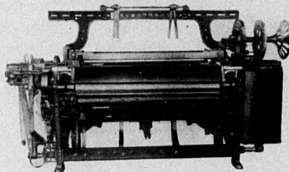
專賣特許阪本式自動織機
