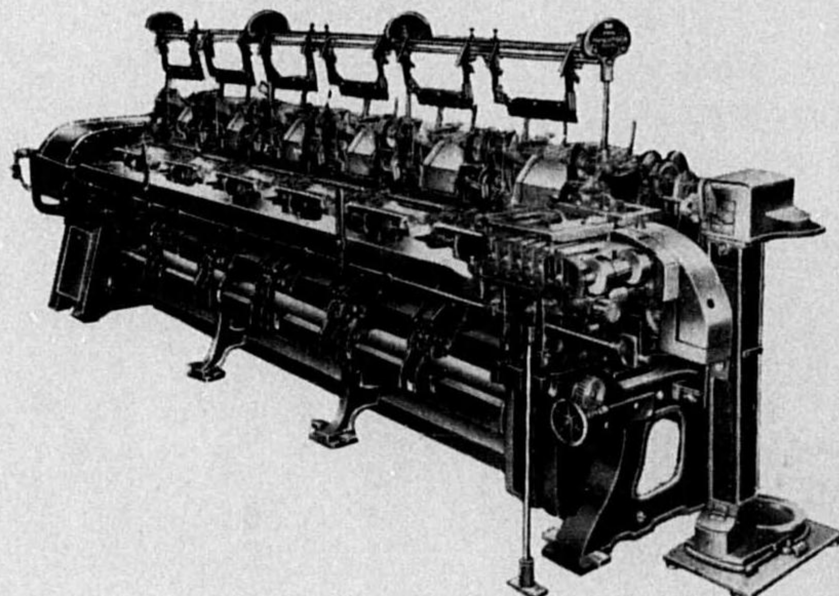
綿紡用コーマー
