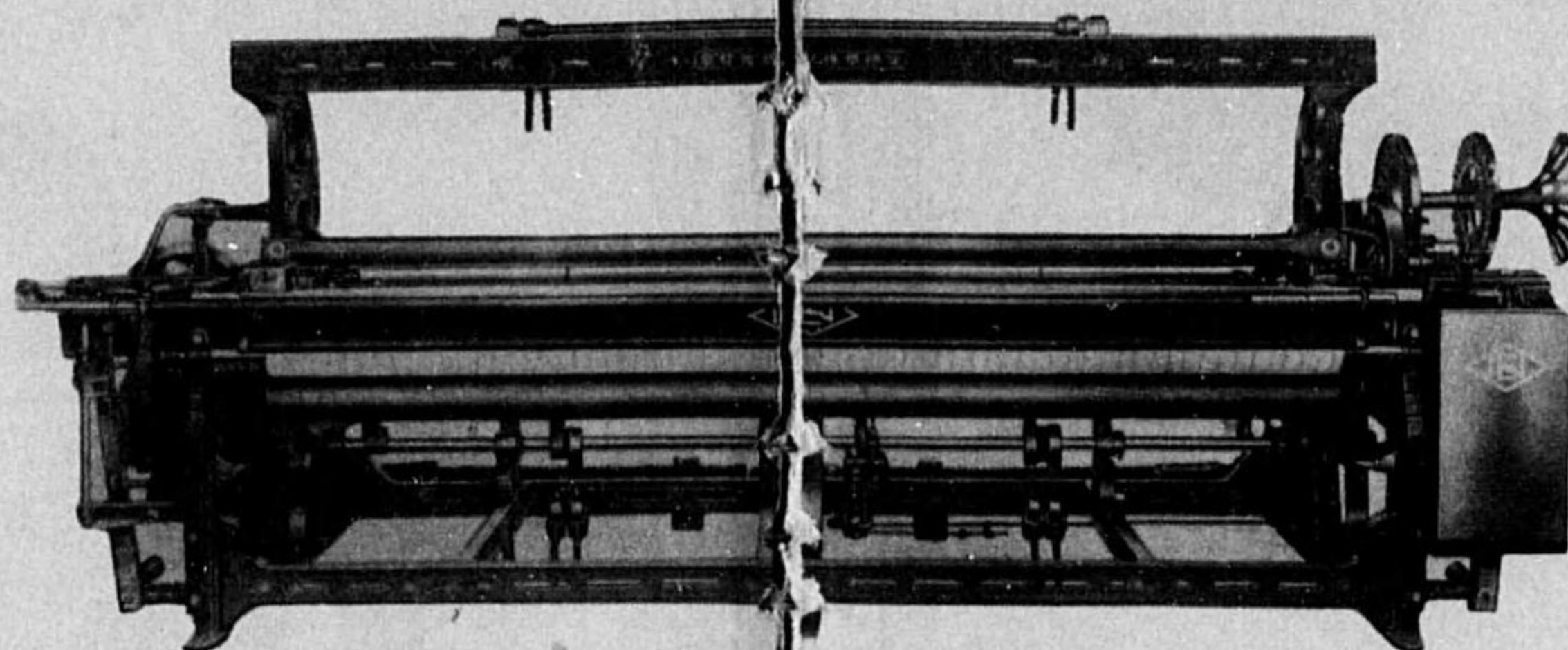
專賣特許 阪本式 超廣幅自動織機 (筵巾98吋)
