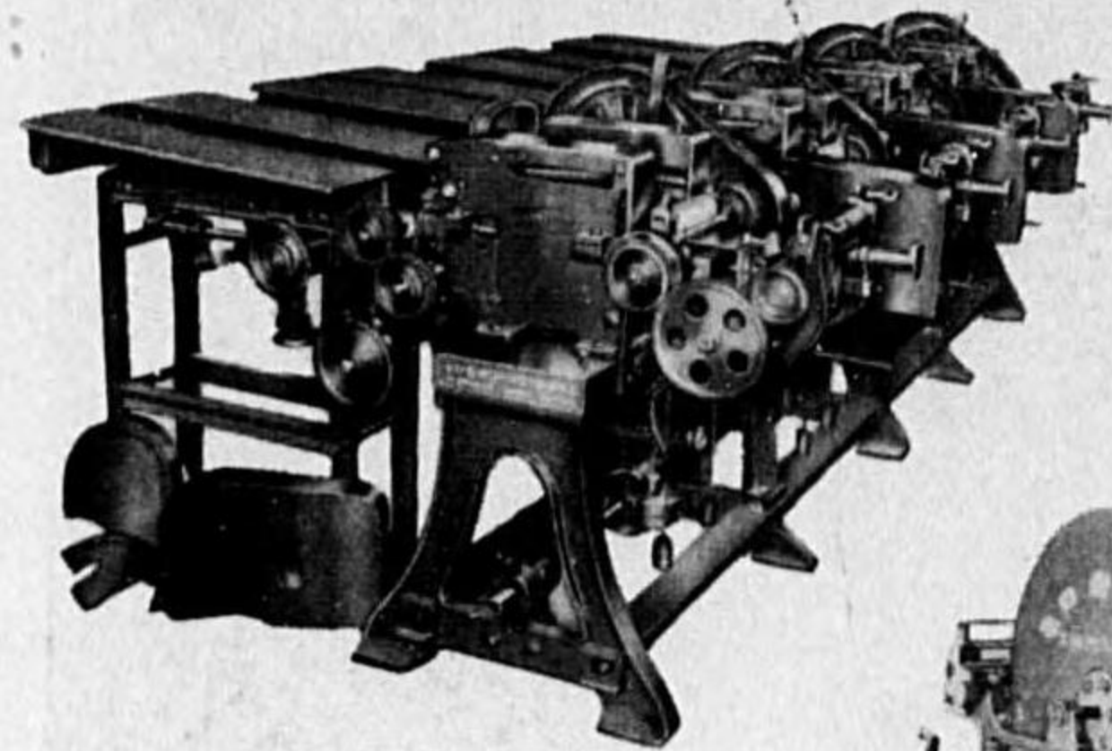
米式製襪機
