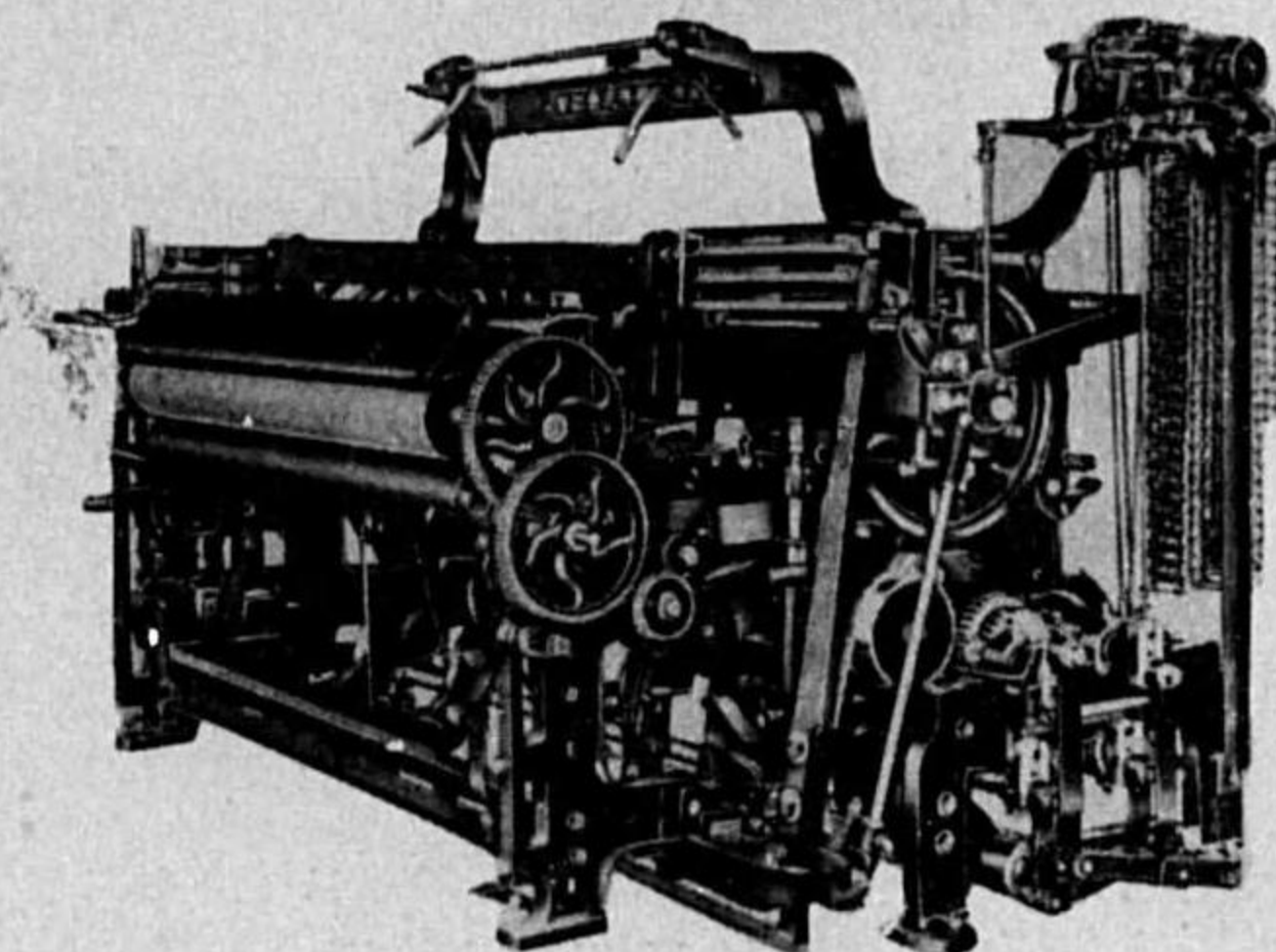
專賣特許阪本式力織機
