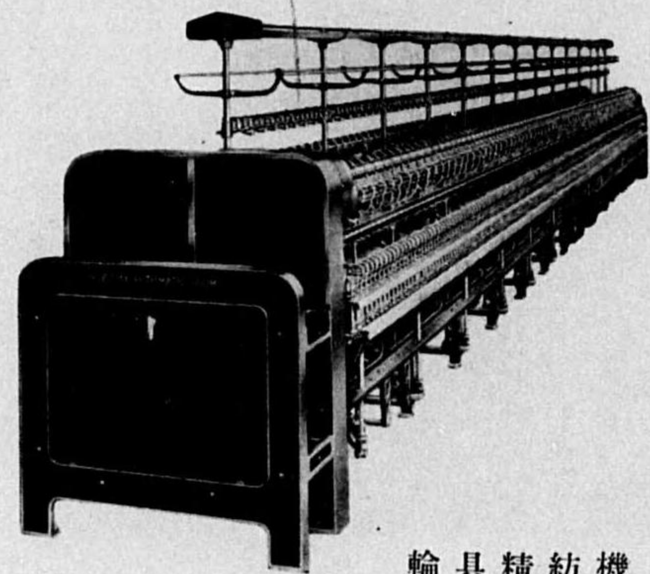
輪具精紡機
