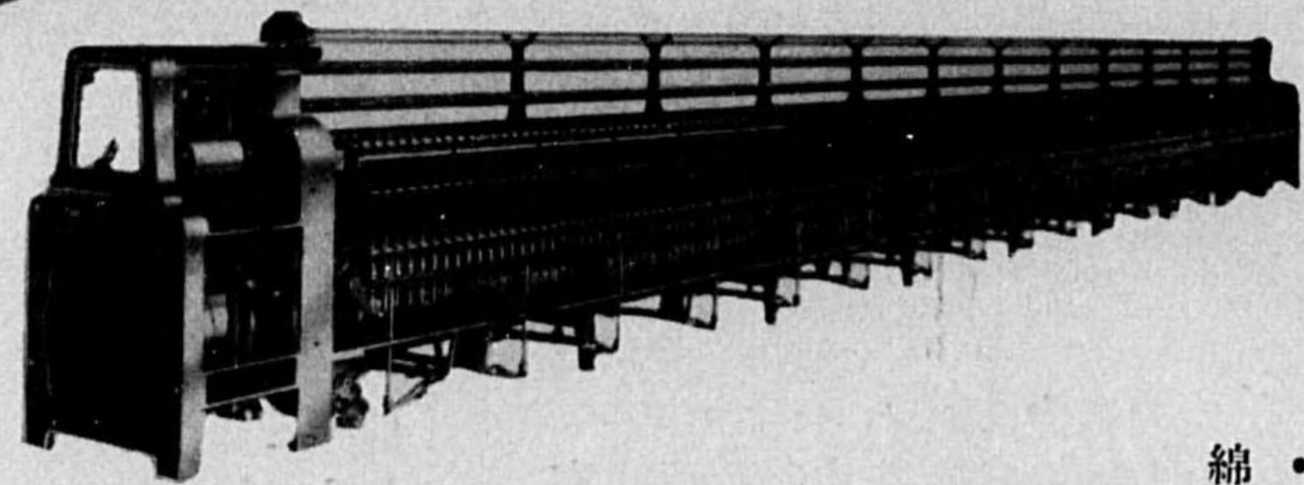
輪具撚糸機
