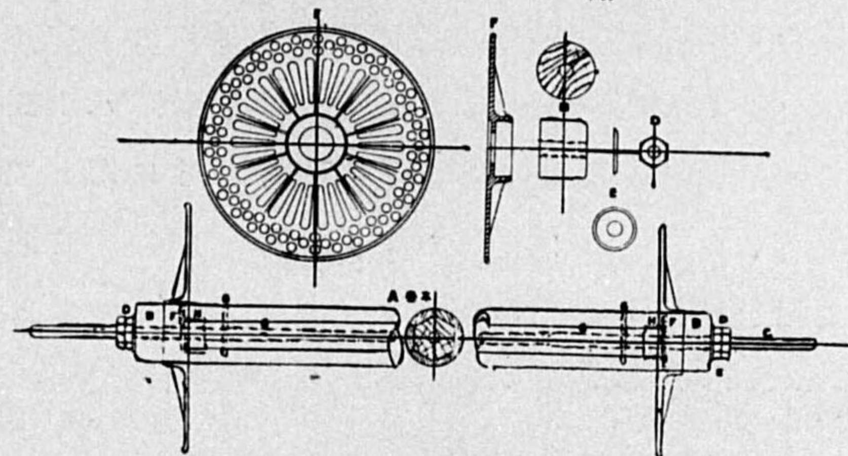
三ツワ式特製新型荒卷ビーム
