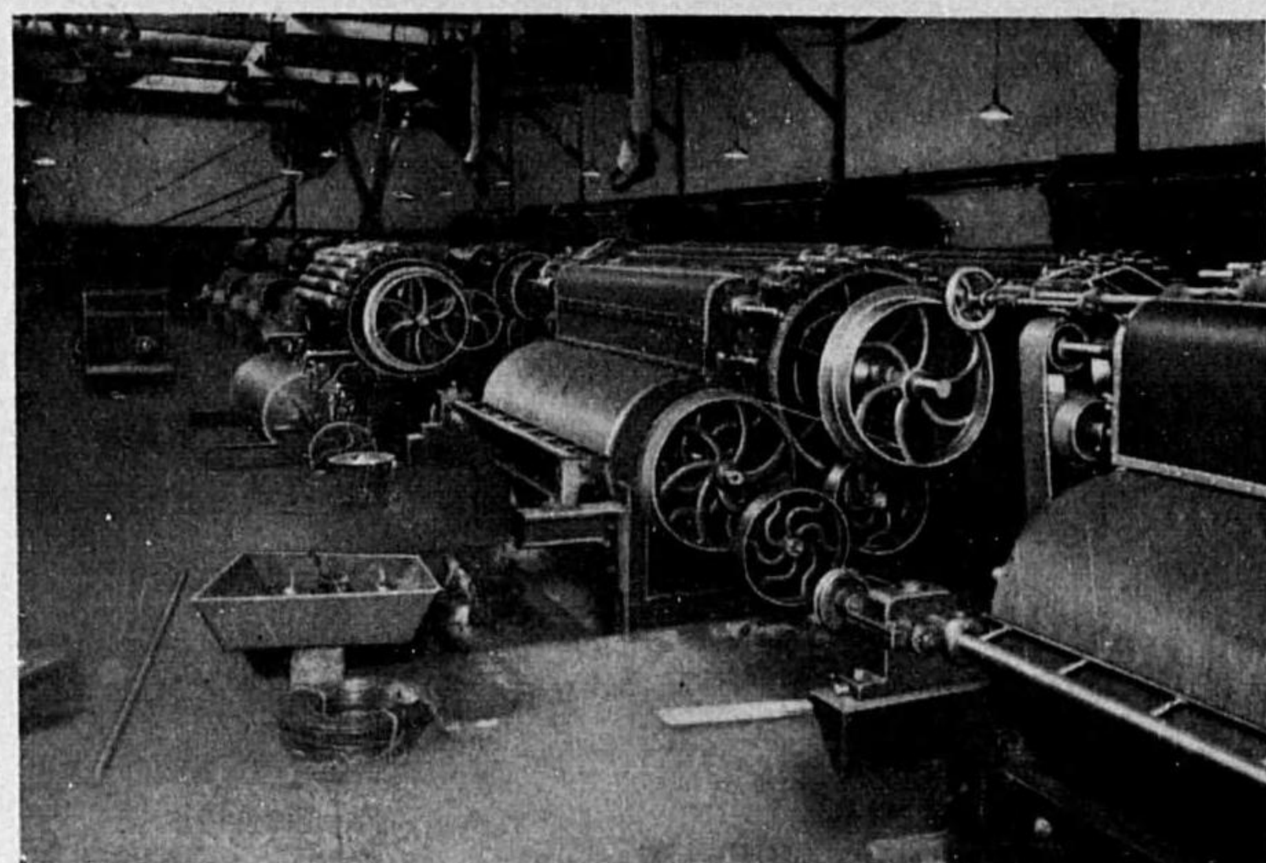
山室式ガーネットマシン
