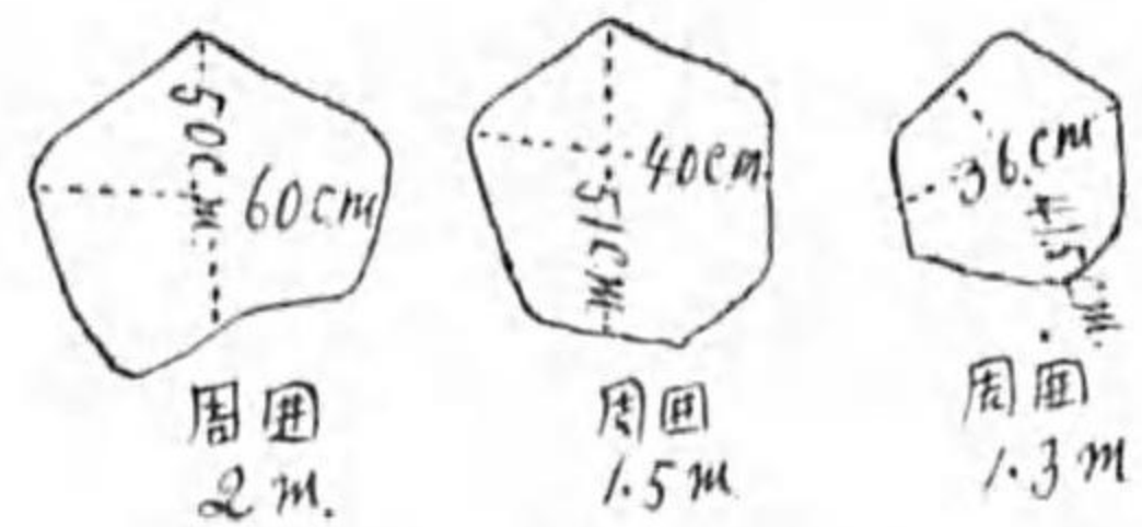
大島ノ粗面岩柱ノ斷面圖 第三十圖
