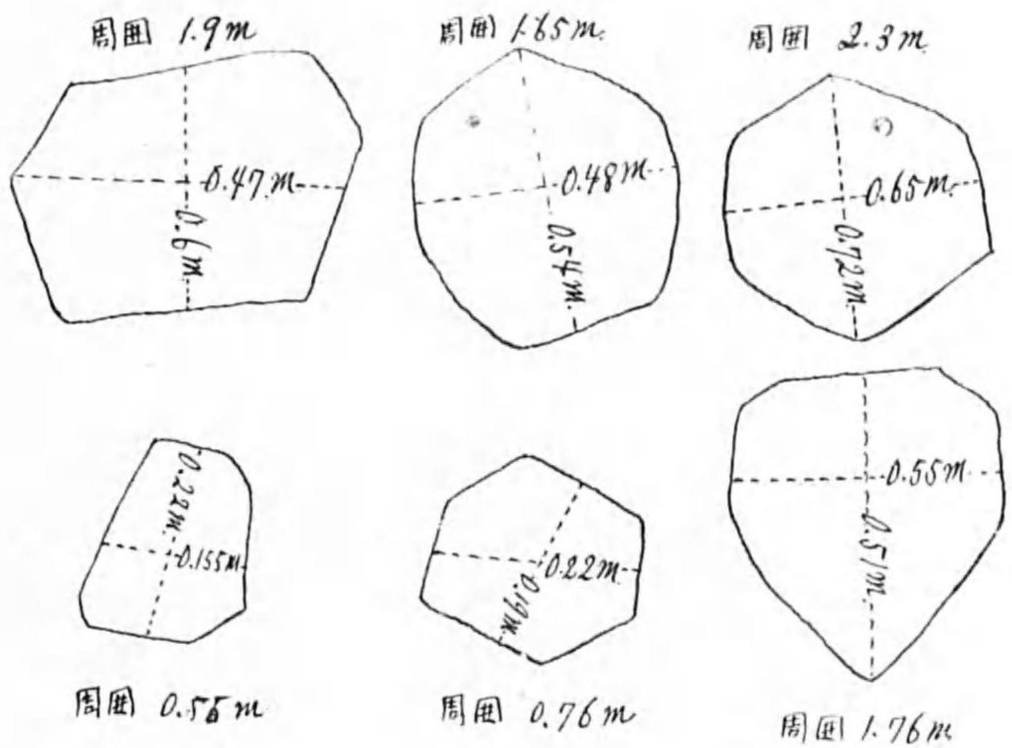
第九圖 青龍洞ノ玄武岩ノ大サ
