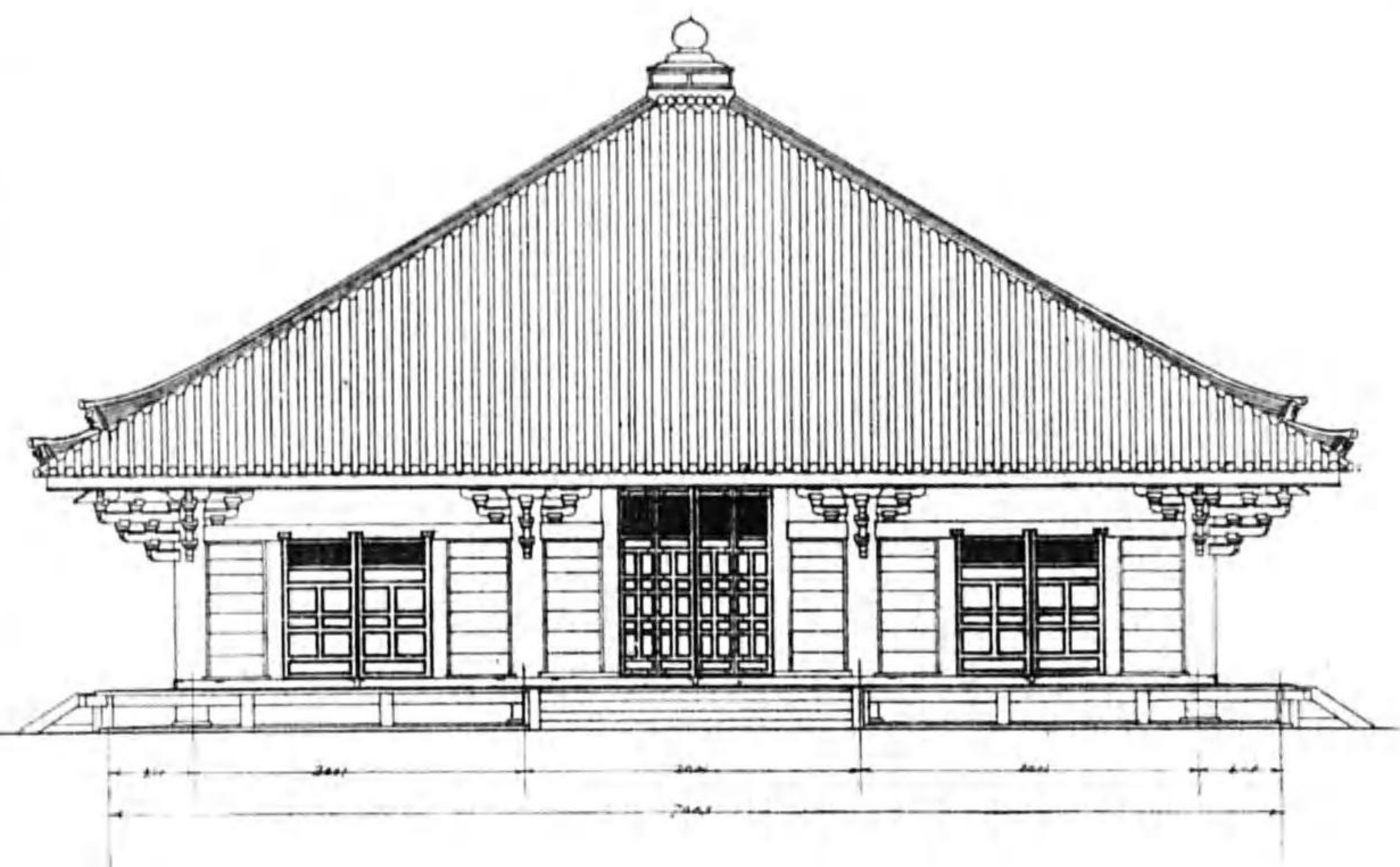
圖版 第三五 (追加) 淨土寺淨土堂正面圖及天井見上圖
