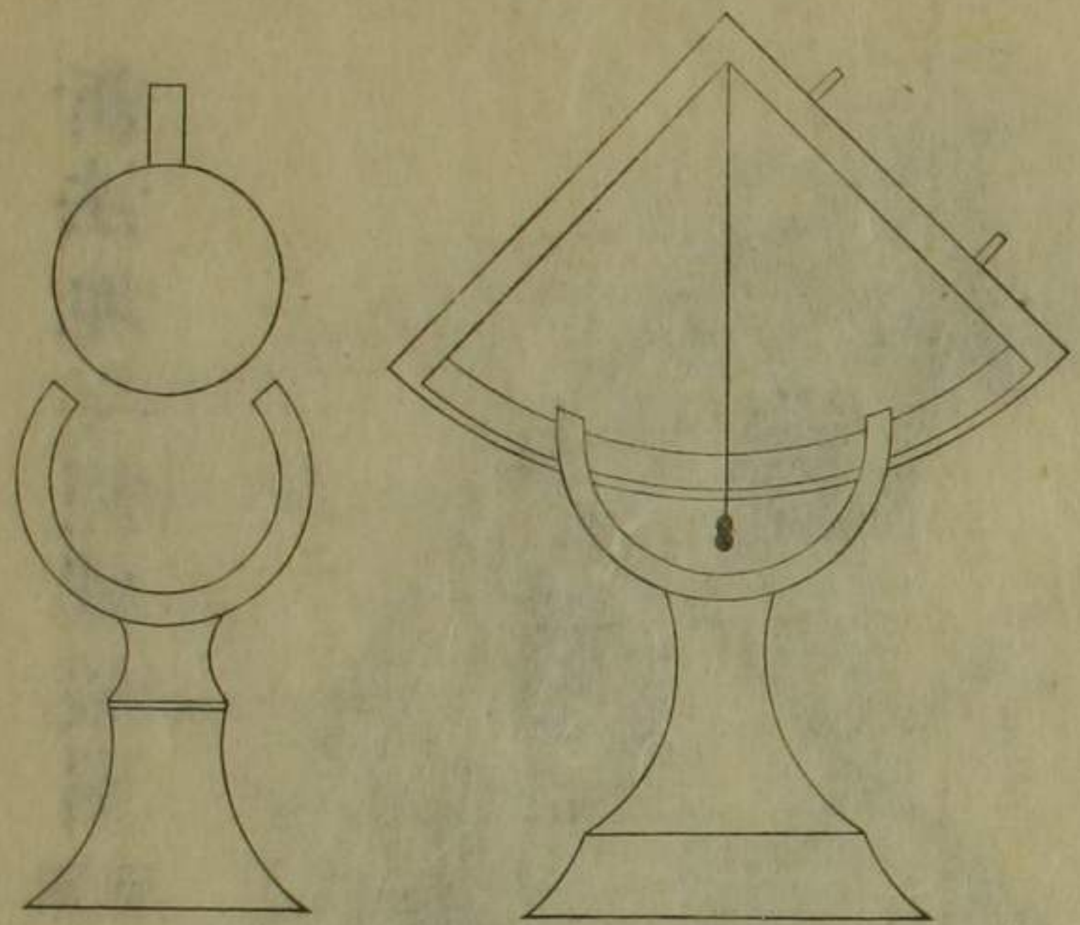
弩儀圖
