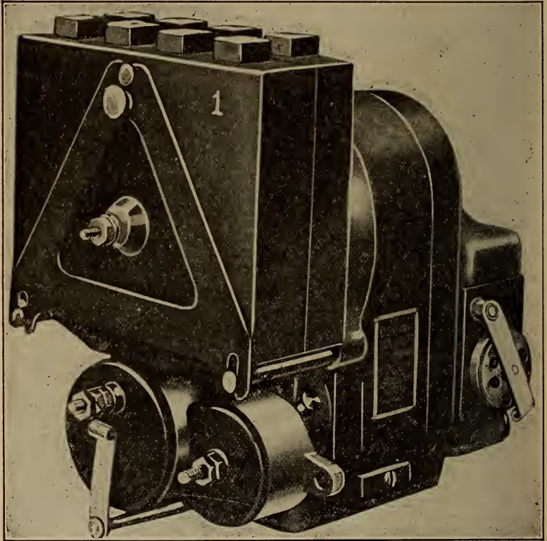
Fig. 63.—Type DD Berling High Tension Magneto.
