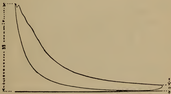
Fig. 14.—Diesel Motor Card.
