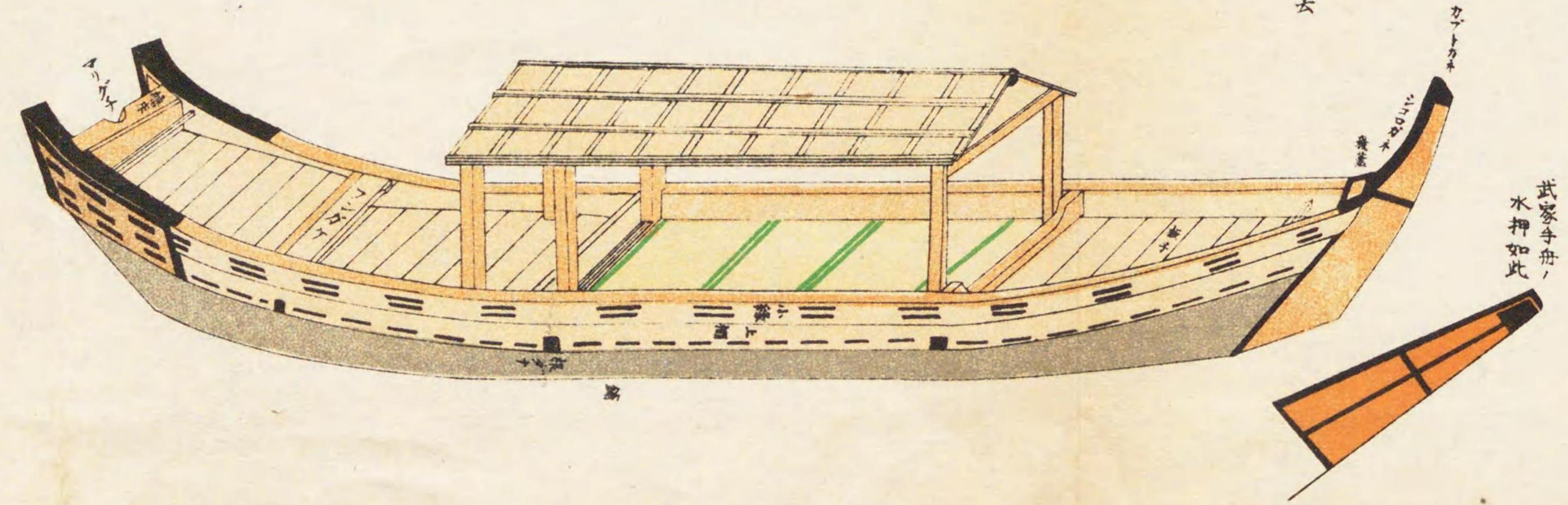
日除船 俗ニ屋根船ト云 但四挺立三挺立二挺立 上口九尺 長二丈五六尺 横六尺
