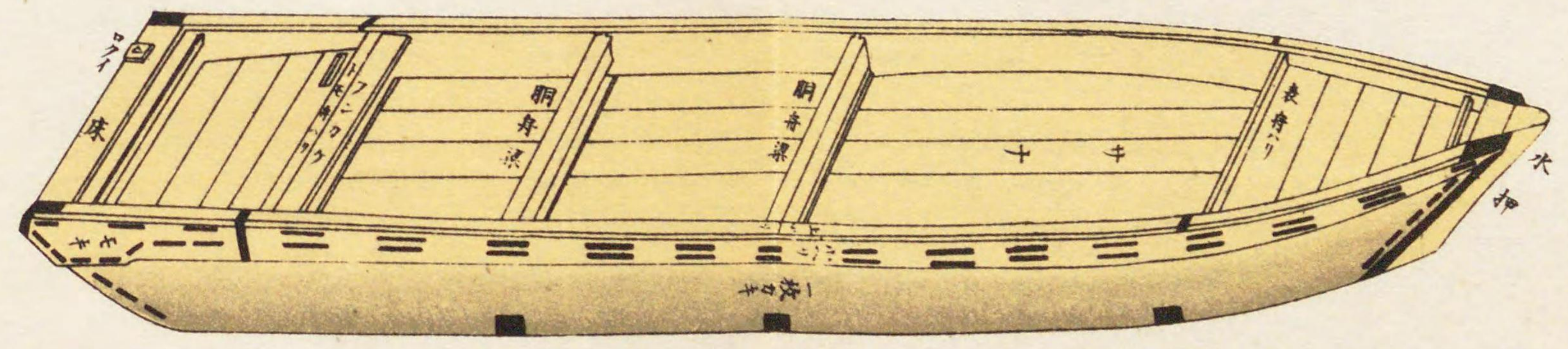
上口九 長二丈四五尺 横六尺位ヨリ七八尺位迄
