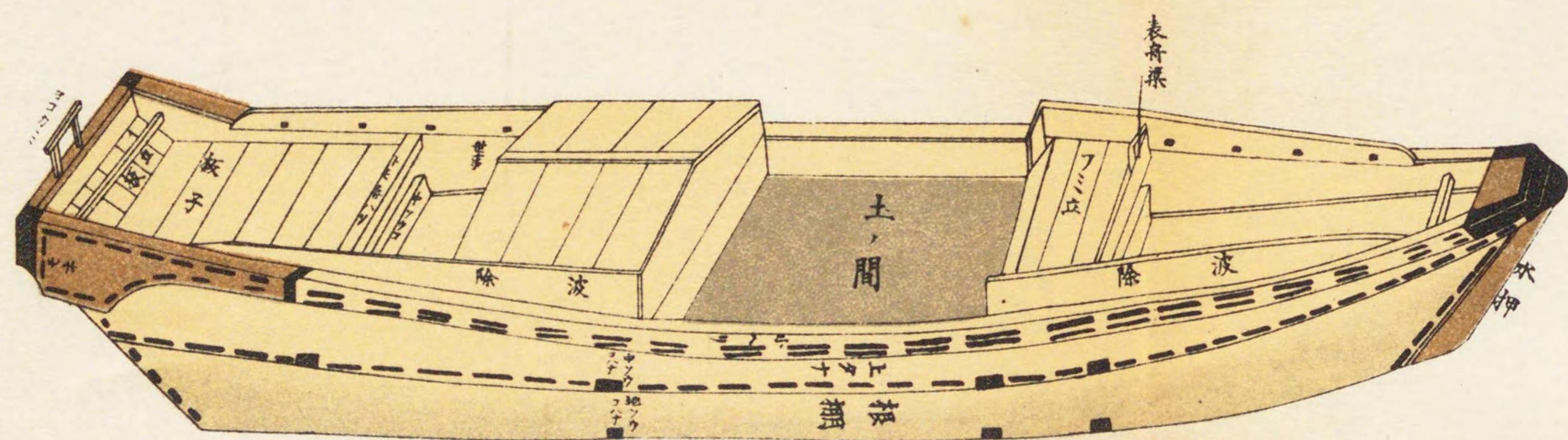
土船 俗ニ土舟ト云 上口九 長二丈八九尺 横八尺位
