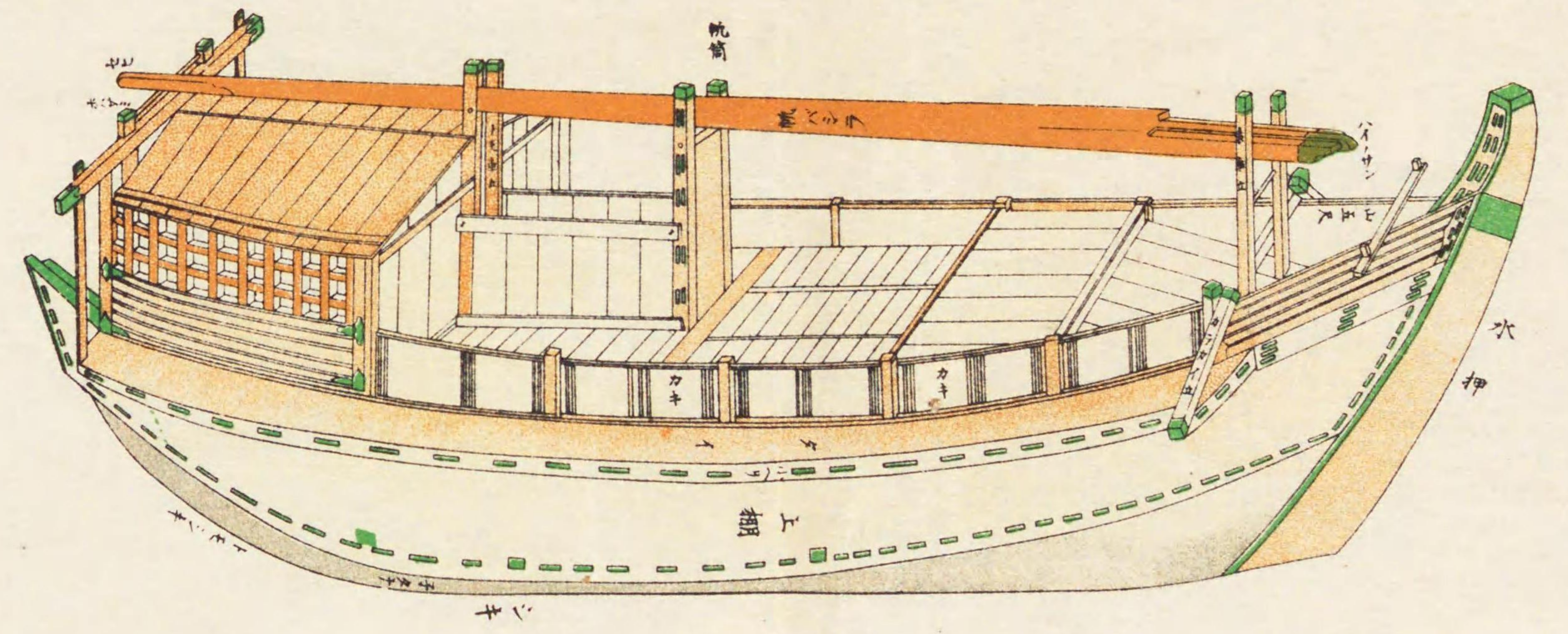
五太力船 櫓付 所ニヨリ 小廻り舟トモ云 武藏 伊豆 相模 安房 上總 辺海付ニ 有之 上口九尺 長同前
