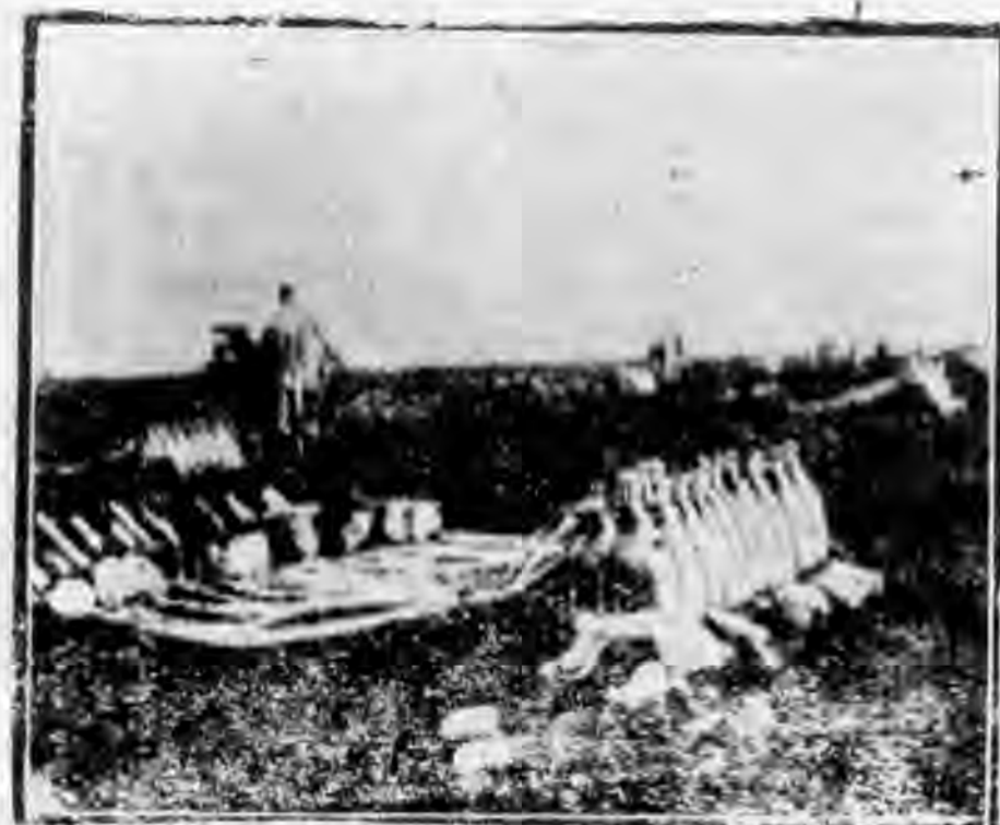
圖七 埋好待放的吹毒鋼瓶，(已與導氣管接好)
