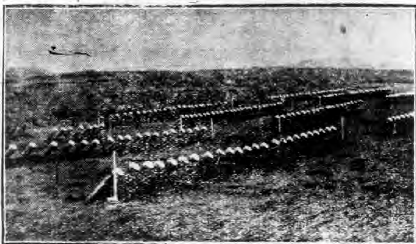
圖八 安好待放的德國式18厘米地射砲。
