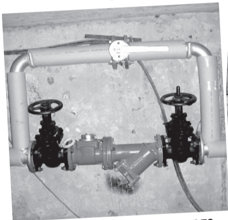
Установка водомерного узла в подвале дома № 2 на ул. Плещеевской
