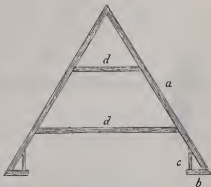
Fig. 1. Takstol.
