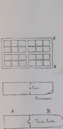
Fig. 45. Båge och karm från Viborgs slott.
