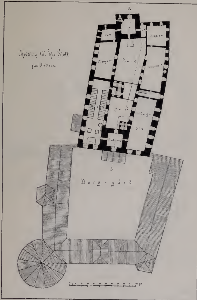
Fig. 4. Åbo slott. Plan af fjärde våningen.
