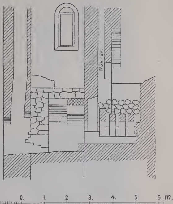
Fig. 40 a. Genomskärning af den gamla ugnen. Betäckningshvalfvet bortlämnadt.
