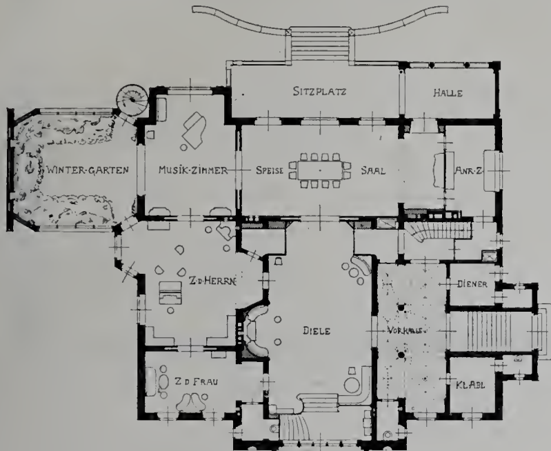
—ERDGESCHOSS—
