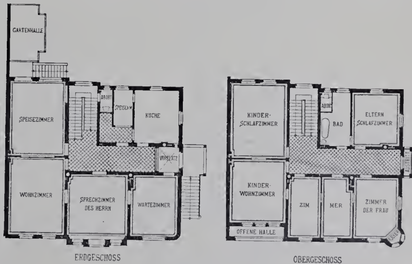
Wohnhaus in Halle, Friedrichstr. 49.
