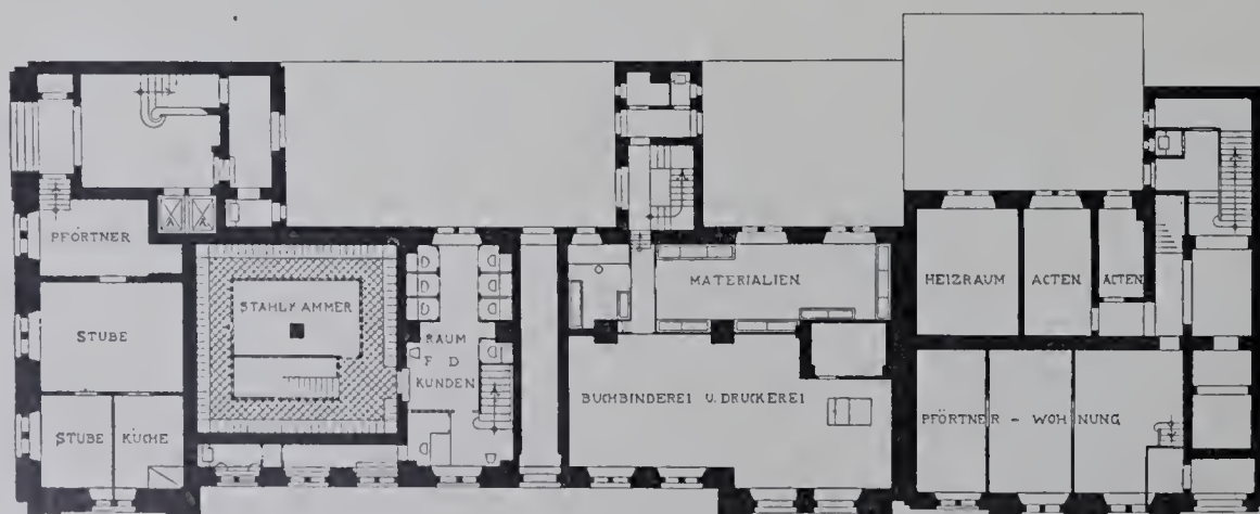
Untergeschoss.
