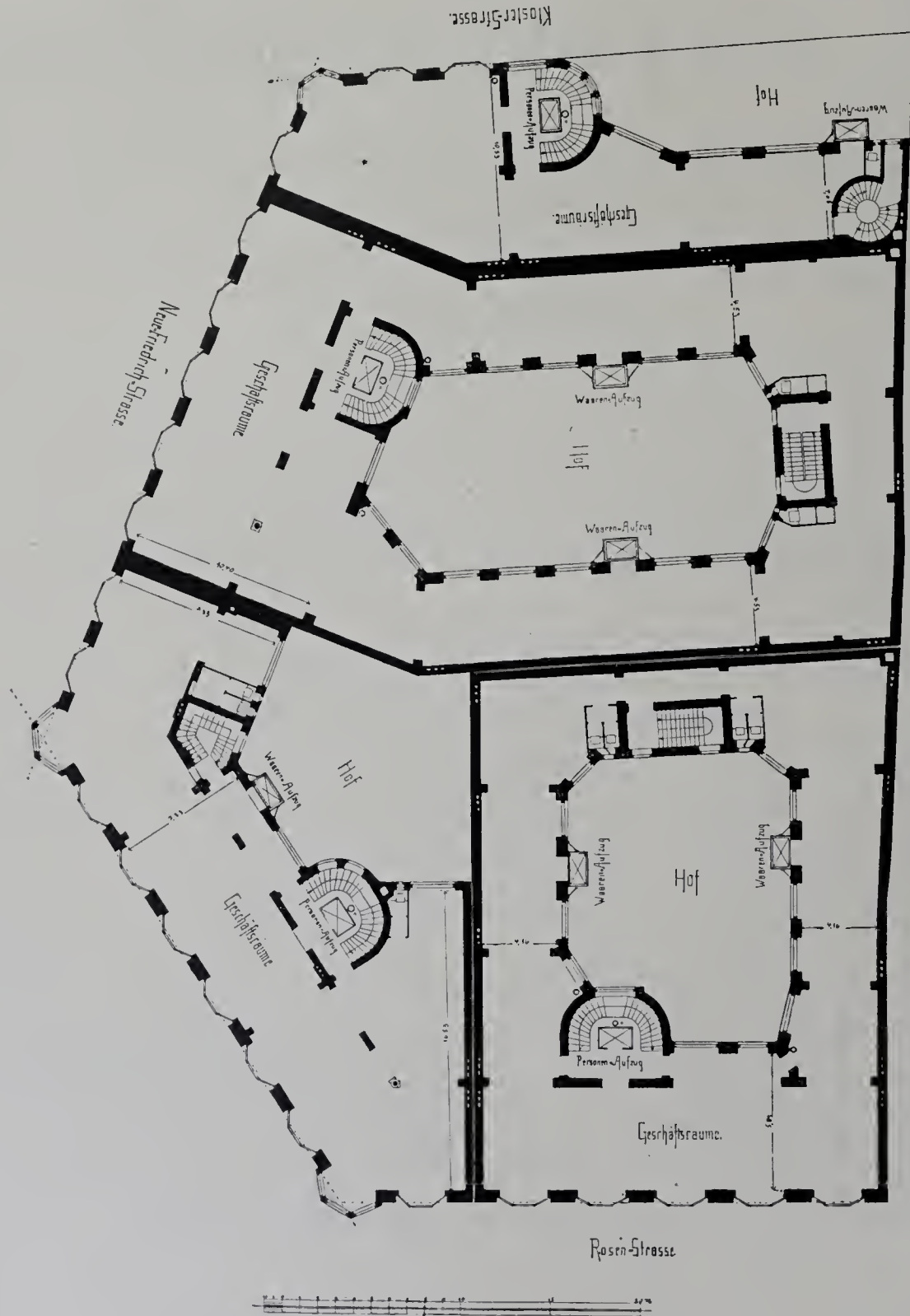
I. Obergeschoss.
