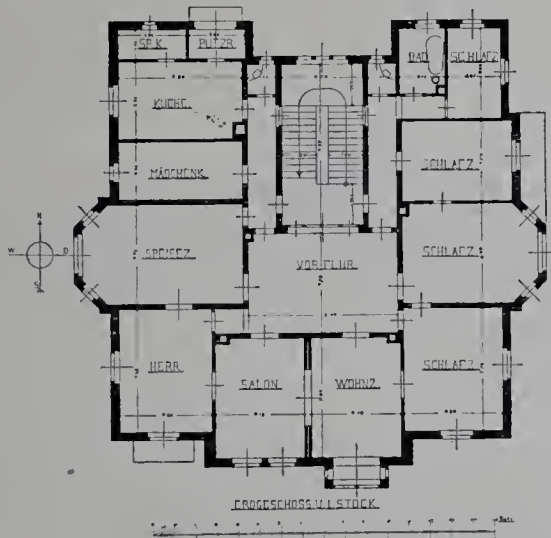
Wohnhaus in Dresden, Comeniusstr. 3.
