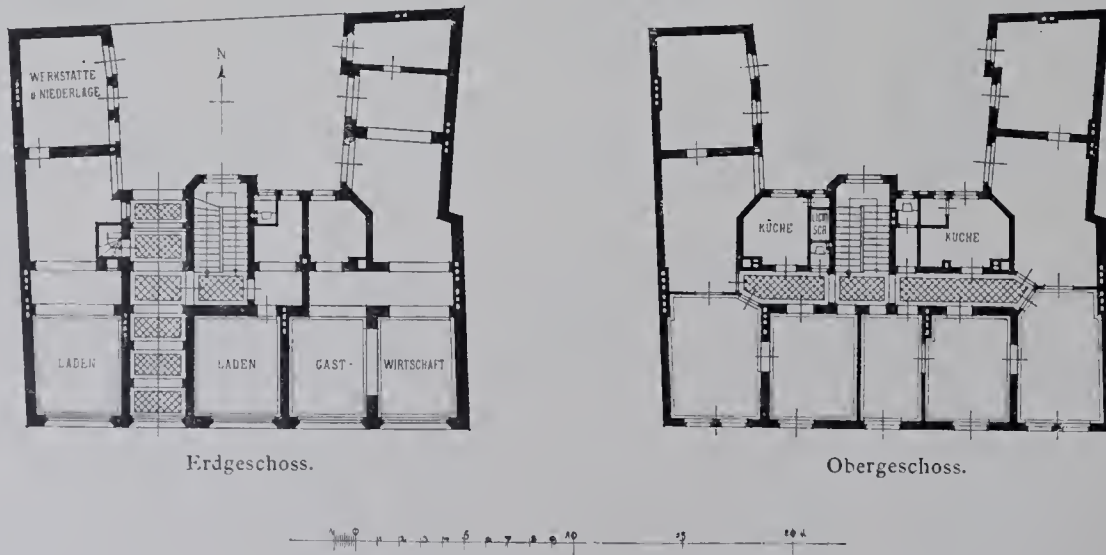
Kauf- und Wohnhaus in Halle, Brüderstr. 2.
