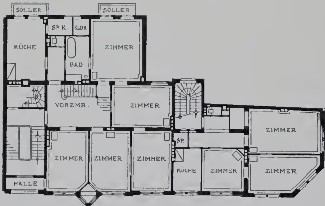
II. Stockwerk.
