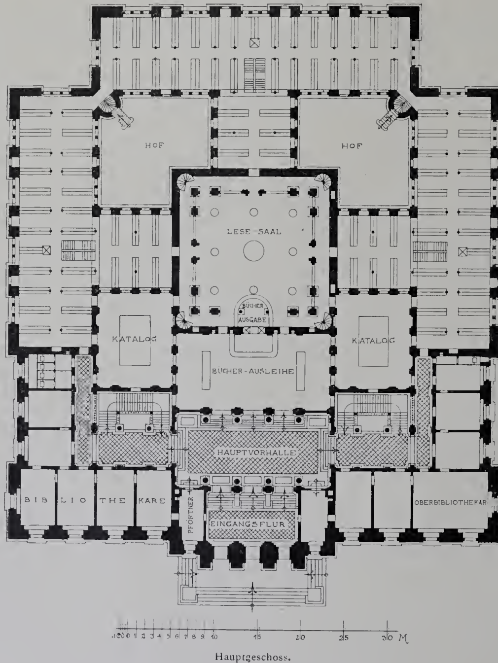
Die Universitäts- und Landesbibliothek in Straßburg i. E.
