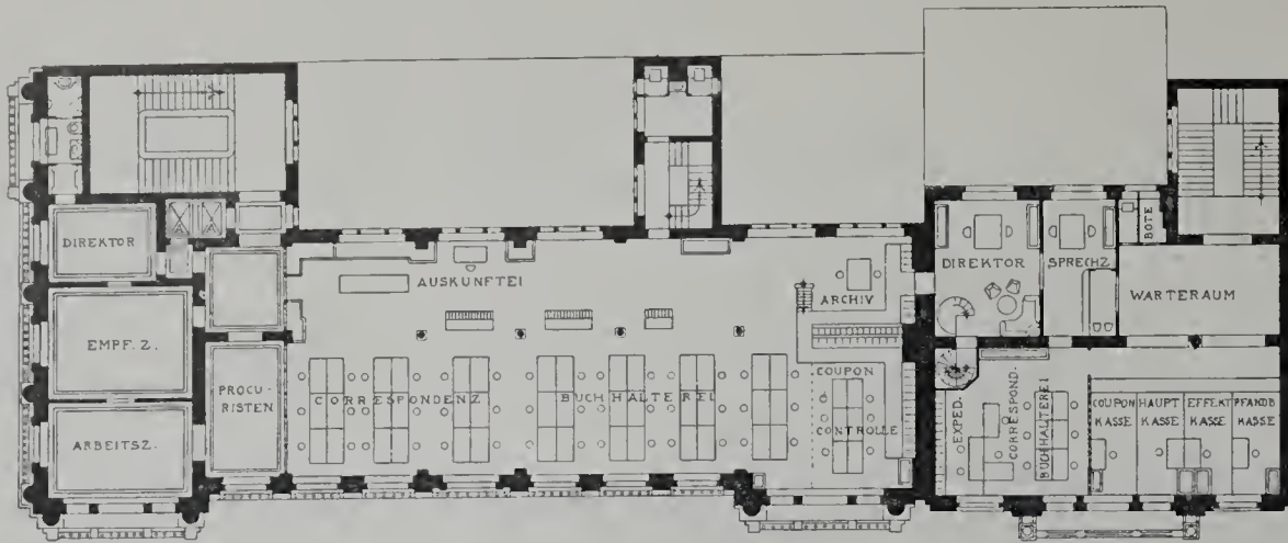
II. Stockwerk.
