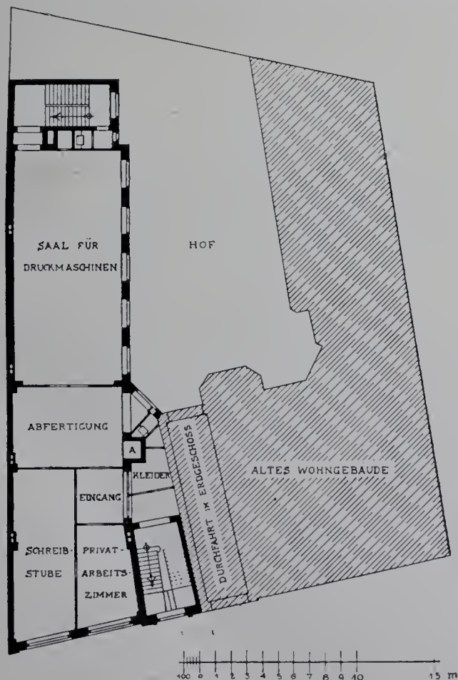
Haus Ullstein in Berlin, Charlottenstr. 10.
