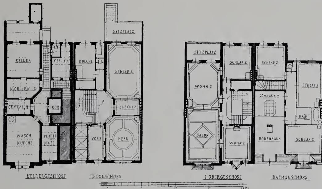
Zwei Wohnhäuser in Halle, Luisenstr. 2 u. 3.
