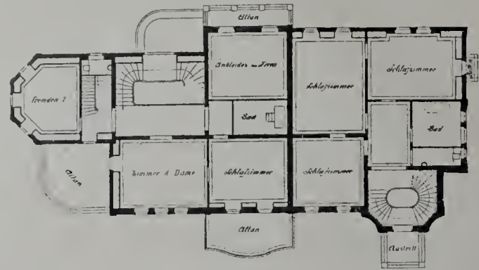
Obergeschoss.
