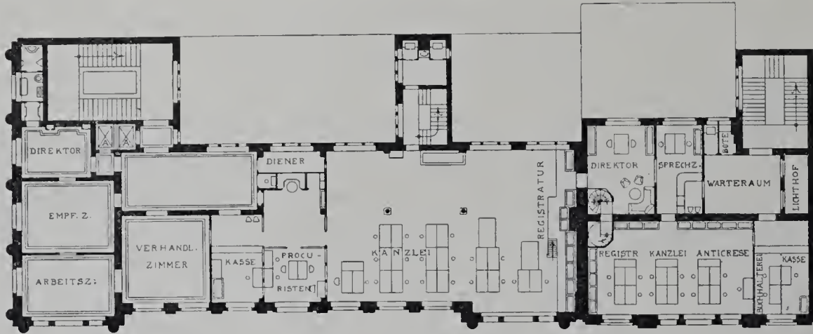
I. Stockwerk.
