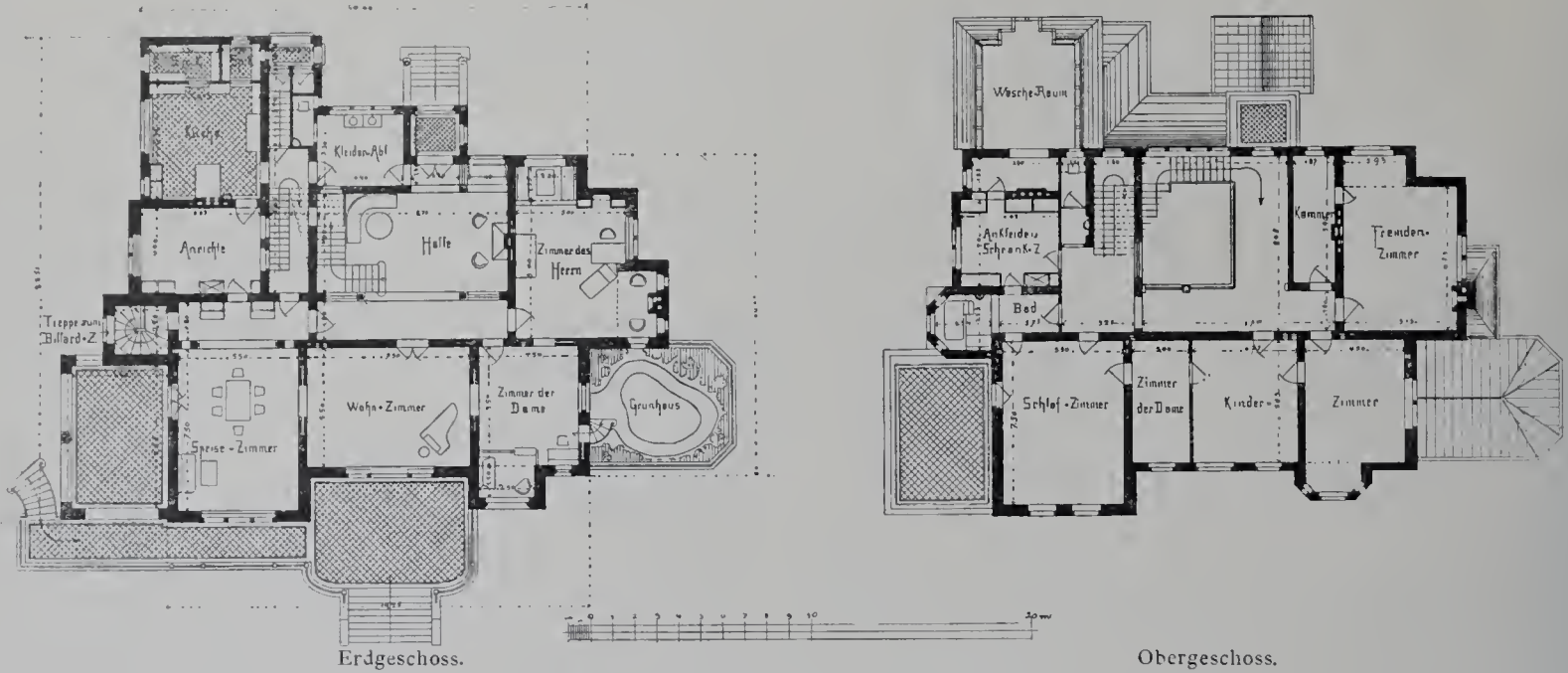
Landhaus Kolbe in Radebeul bei Dresden.
