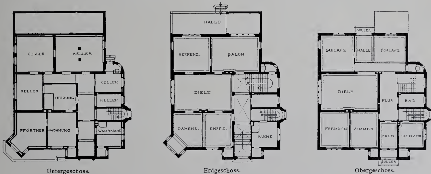
Landhaus in Halle, Händelstr. 16.
