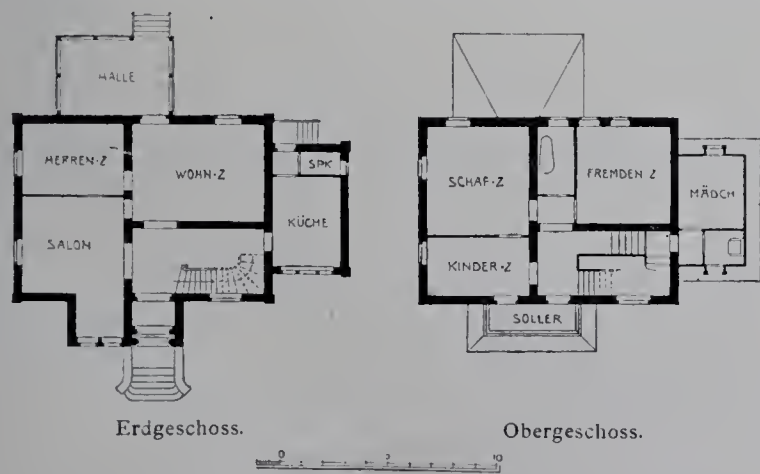
Landhaus in Gr. Lichterfelde, Marthastr. 2.
