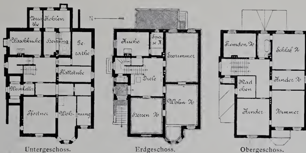
Landhaus K. Reimer in Grotto-Lichterfelde, Grabenstr. 35.
