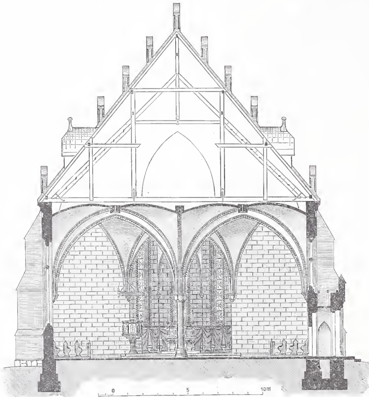
Abb. 2. Querschnitt.
