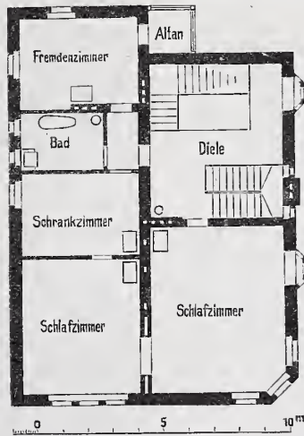
Abb. 3. Obergeschoss.
