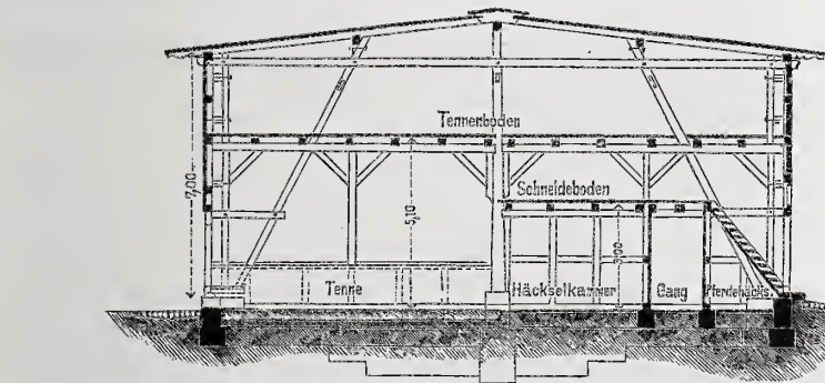
Abb. 5. Querschnitt.
