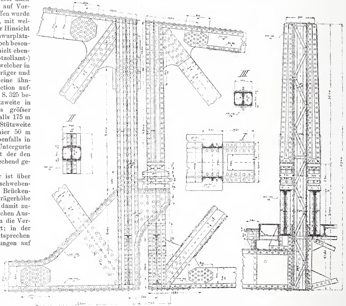
Seitenansicht. Abb. 15. Anordnung der freischwebenden Stützpunkte.
