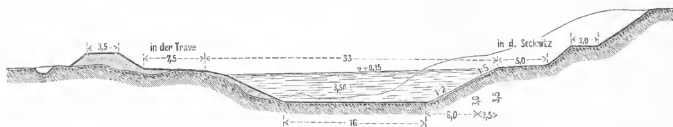
Abb. 3. Querschnitt in der Trave und unteren Stecknitz.
