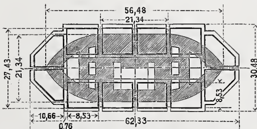
Abb. 8. Aufsicht auf die Kasten und Schnitt A-A durch einen Strompfeiler.
