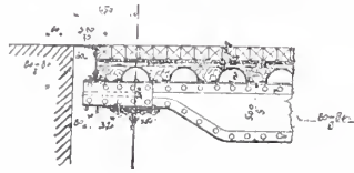
Abb. 17. Anschluß der Fahrbahn an die Widerlager.
