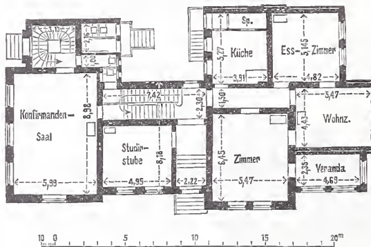
Abb. 4. Erdgeschoss.
