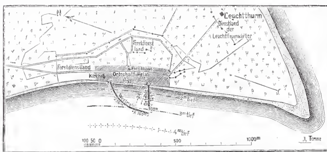
Abb. 1. Lageplan.
