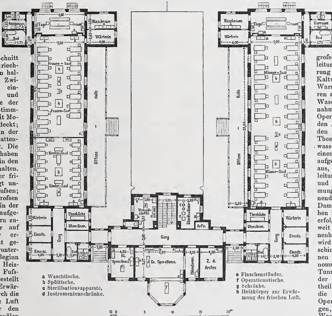
Abb. 1. Erdgeschoss.
