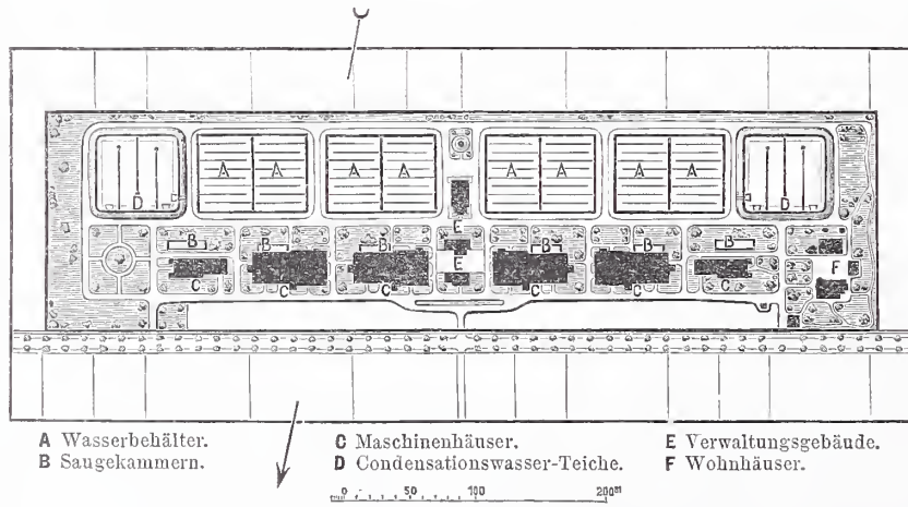
Abb. 2. Lageplan des Werkes Lichtenberg.
