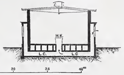
Abb. 3. Querschnitt X Y.
