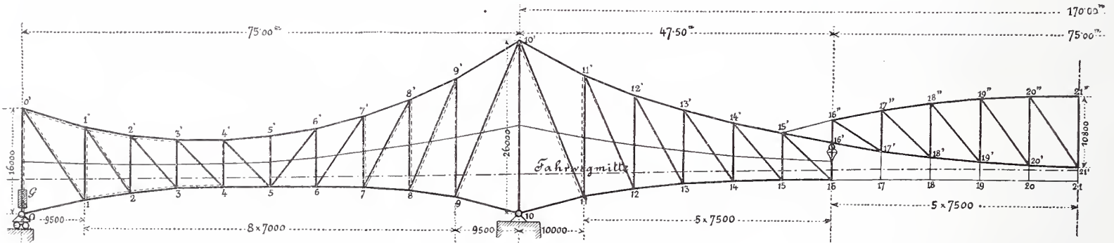
Abb. 35. Hauptträgersystem.
