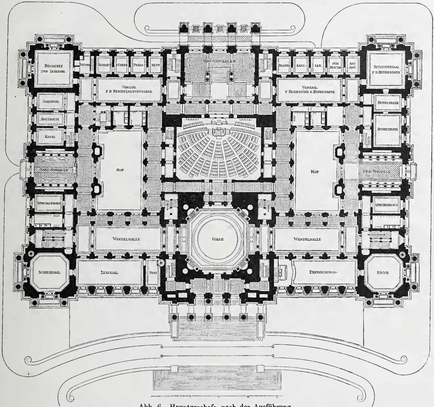
Abb. 6. Hauptgeschofs, nach der Ausführung. Reichstagshaus in Berlin.
