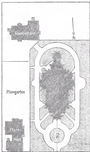
Abb. 3. Lageplan.
