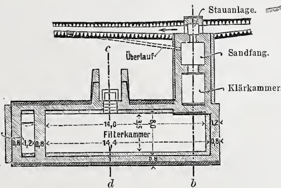
Abb. 6. Grundriß.
