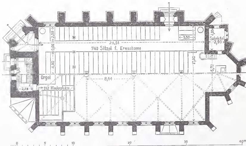
Abb. 3. Grundriß.
