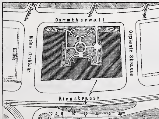
Abb. 1. Lageplan.
