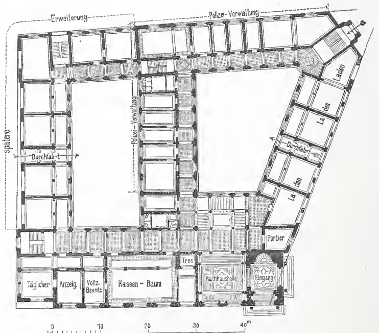
Abb. 13. Entwurf von Erdmann u. Spindler in Berlin (Ein vierter Preis). Erdgeschofs.
