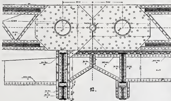
Abb. 30. Das Mittelgelenk der Tragwand.
