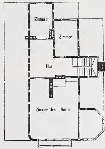
Abb. 4. Dachgeschoss.
