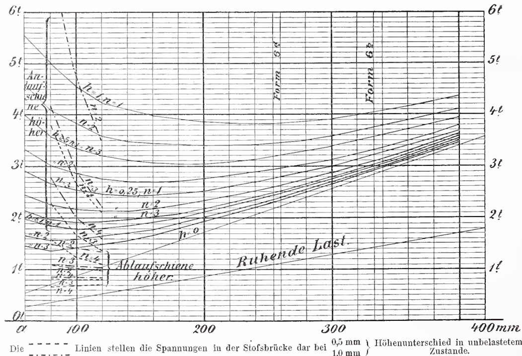
Abb. 5. Spannungen.
