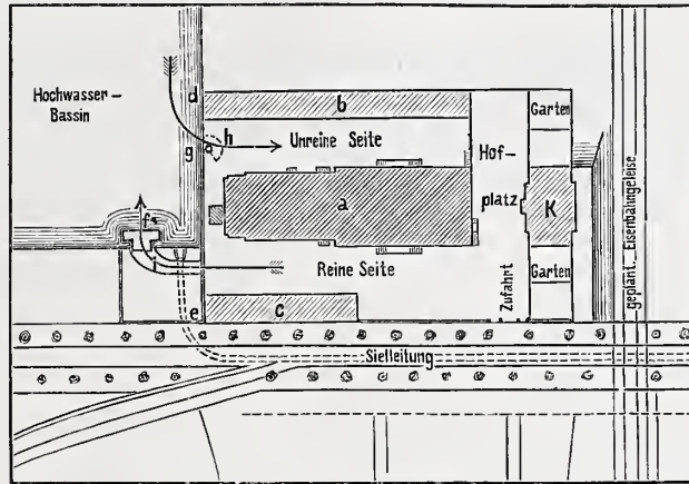
Abh. 1. Lageplan.
