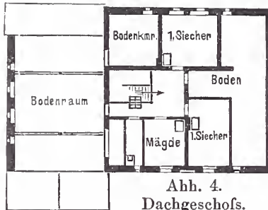
Abb. 4. Dachgeschoss.
