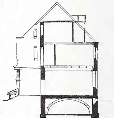
Abb. 7. Schnitt ab.
