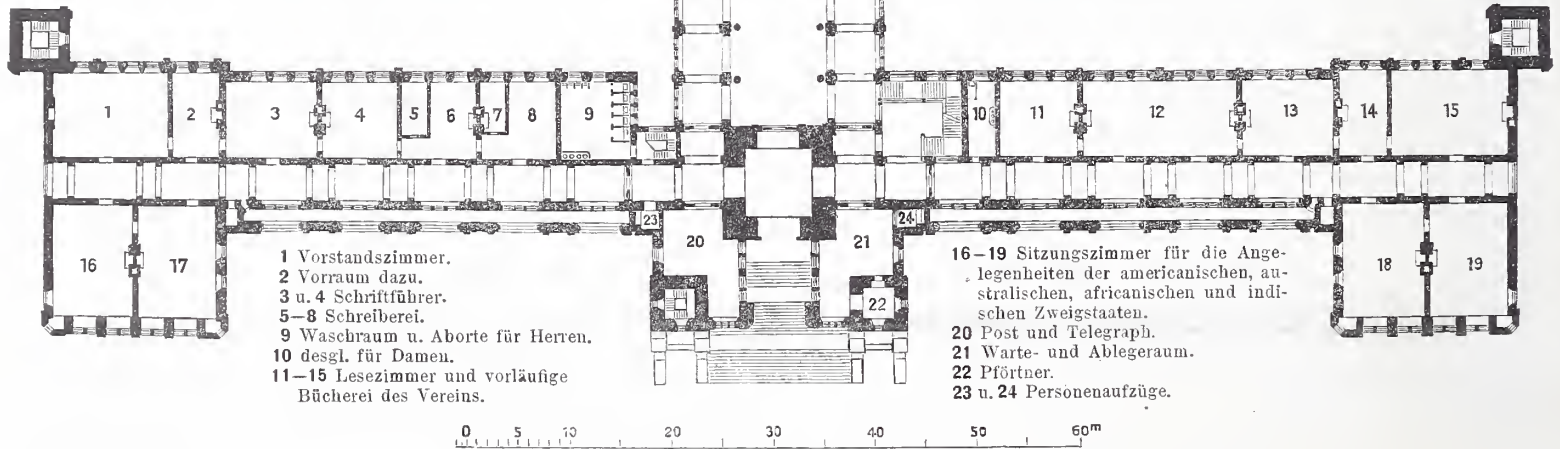
Abb. 2. Grundriss des Erdgeschosses.
