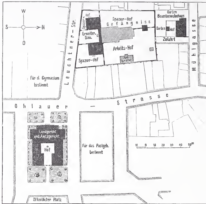
Abb. 2. Lageplan.
