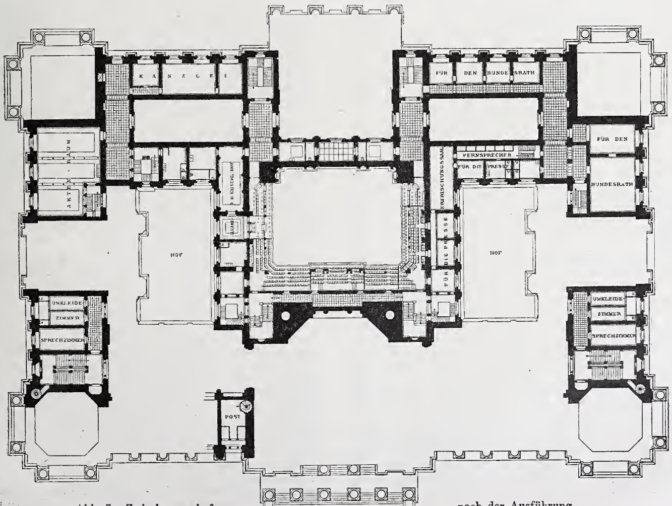
Abb. 7. Zwischengeschofs,
