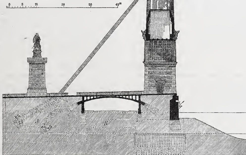
Abb. 26. Brücke am Schwurplatz in Budapest. Entwurf von A. Rieppel, Fr. Thiersch u. W. Dietz.
