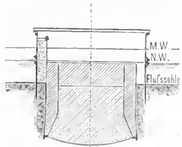
Abb. 5. Schnitt A B.
