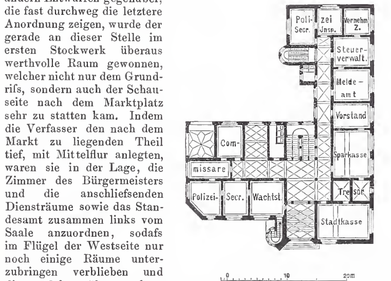
Abb. 1. Erdgeschoss. Entwurf von Reinhardt u. Süßenguth in Berlin (I. Preis).
