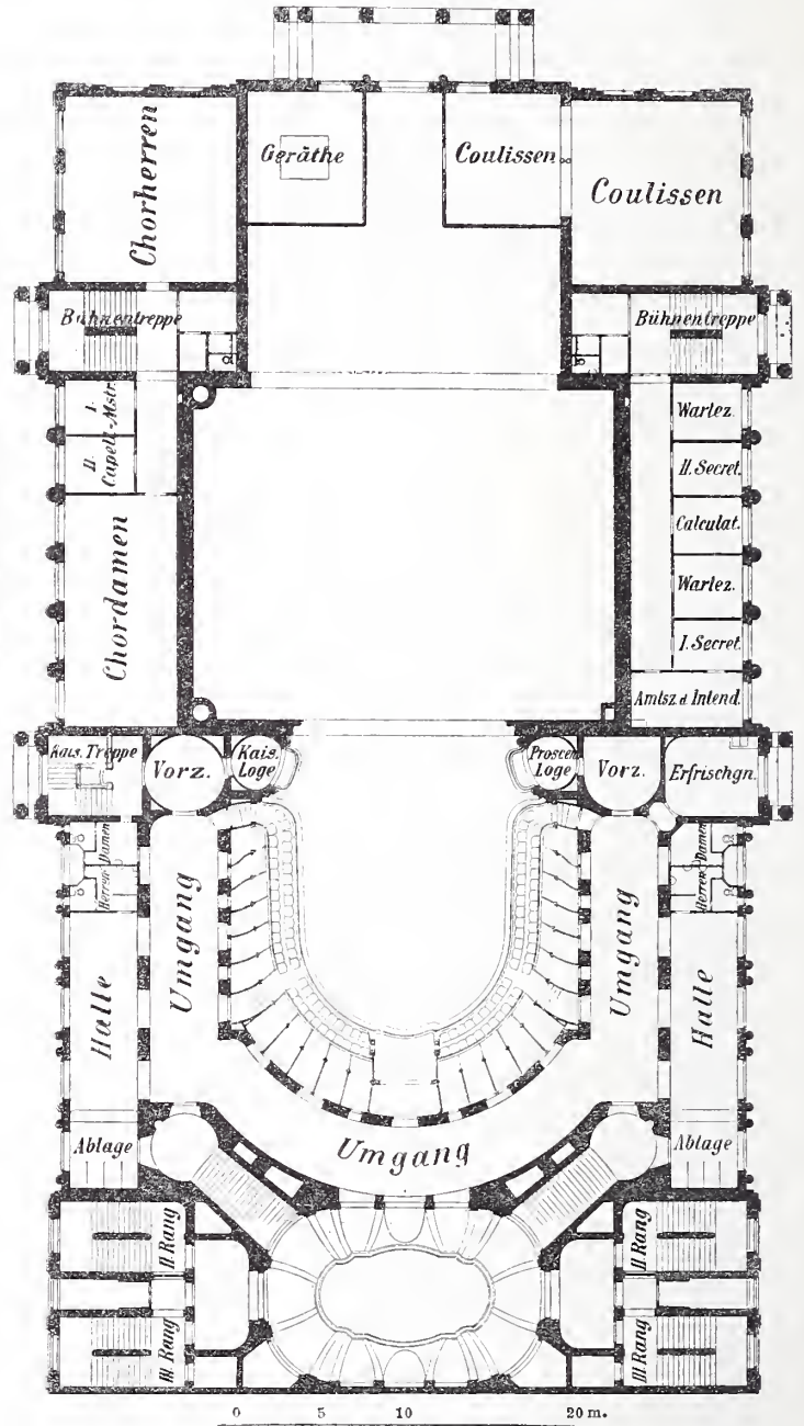
Abb. 3. Grundriß des I. Ranges.
