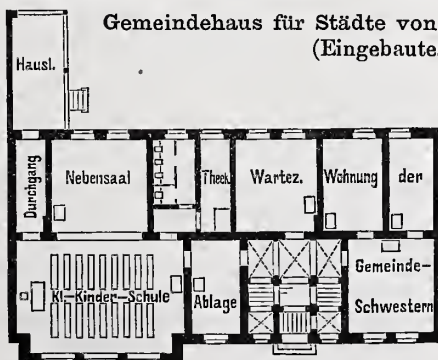
Abb. 13. Erdgeschoss.
