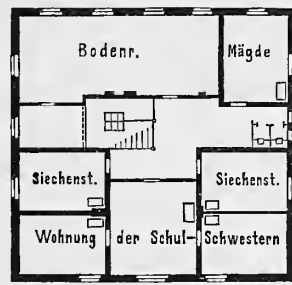
Abb. 11. I. Stockwerk.
