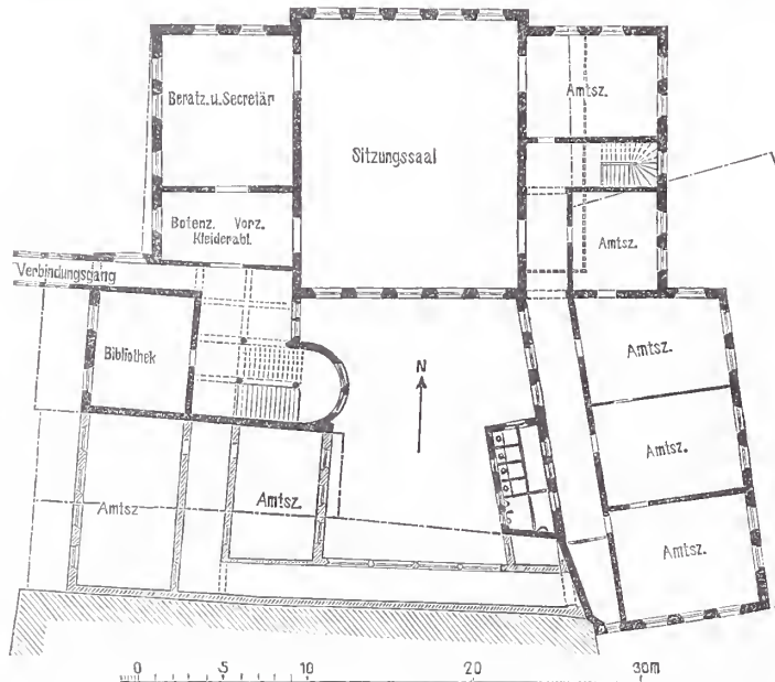
Abb. 2. II. Stockwerk. Städtisches Amtshaus am Fünferplatz in Nürnberg.
