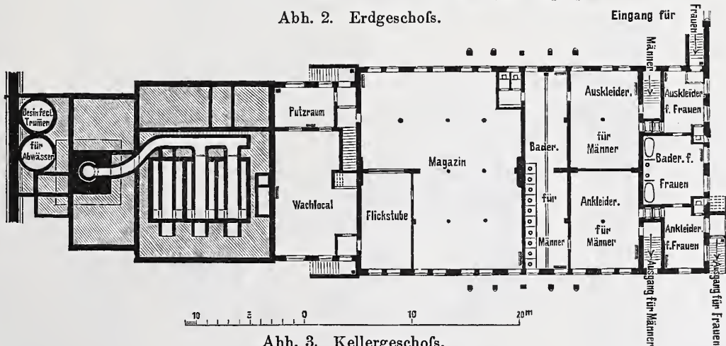
Abh. 3. Kellergeschoss. Desinfectionsanstalt am Bullerdeich.
