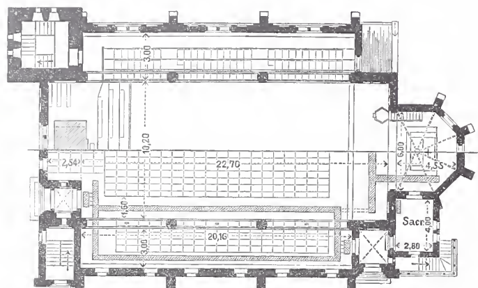
Grundrifs in Erdgeschoss- u. in Emporenhöhe.
