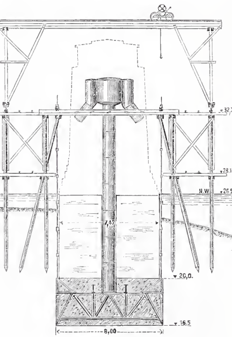
Abb. 7. Querschnitt.
