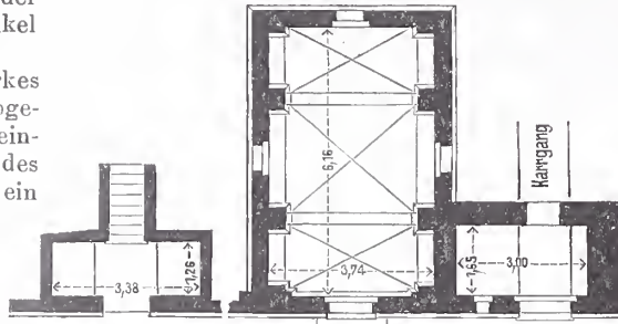
Abb. 6. Grundriss.
