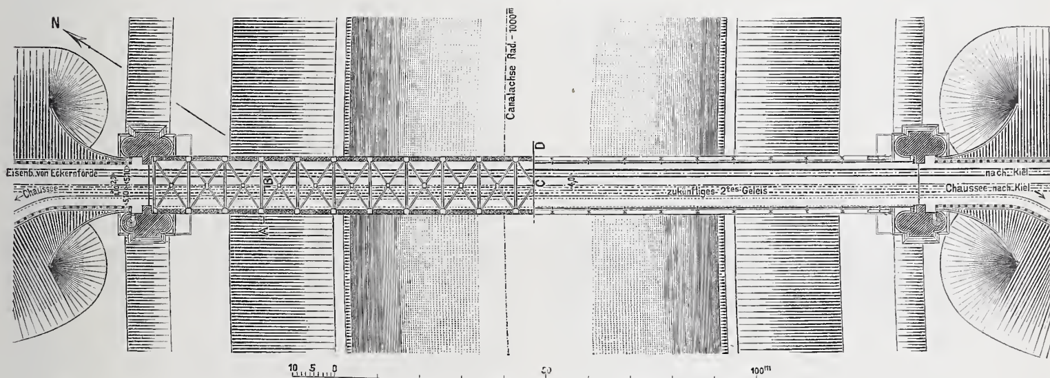
Abb. 6. Oberansicht und wagerechter Schnitt über der Fahrbahn.
