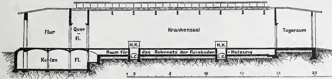
Abb. 2. Längenschnitt.
