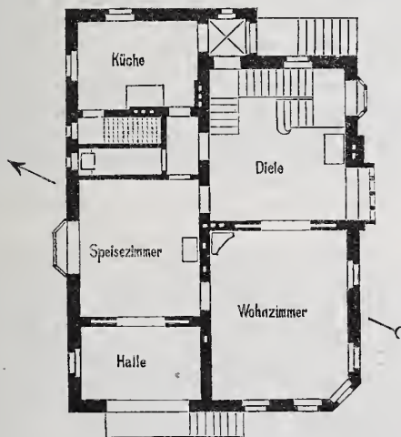
Abb. 2. Erdgeschoss.
