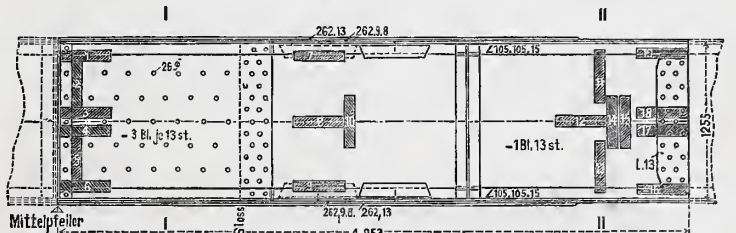
Abb. 6. Seitenansicht mit Bezeichnung der Stegblechproben.
