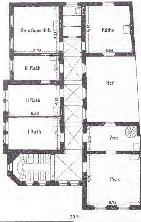
Abb. 2. Obergeschoss.
