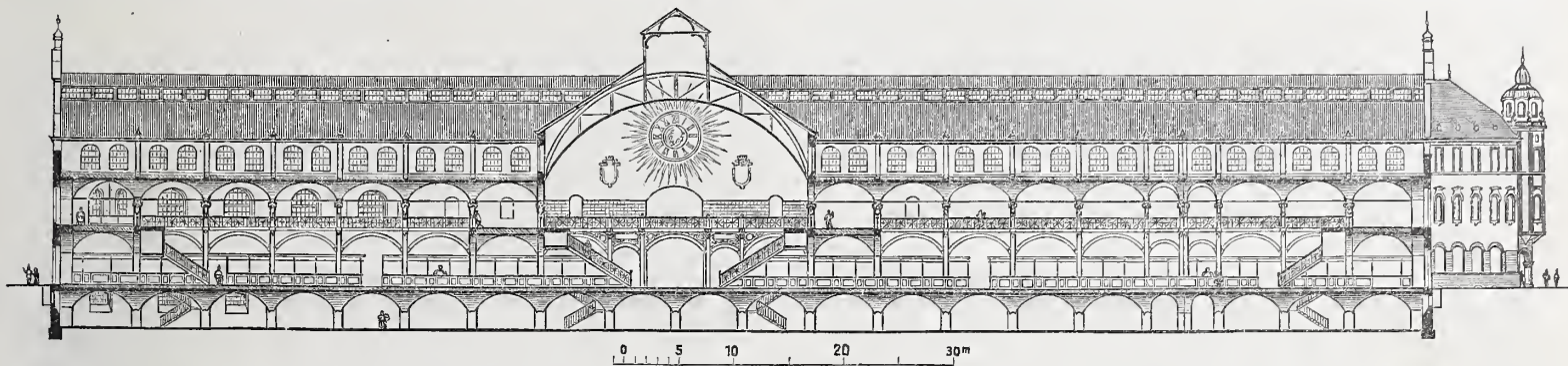
Abb. 3. Längenschnitt.
