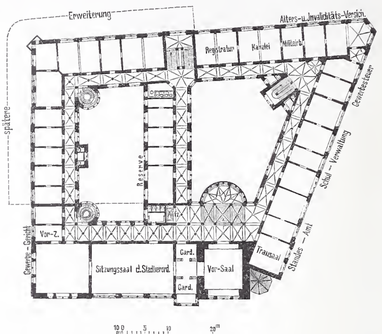
Abb. 6. Entwurf von H. Reinhardt in Berlin (Ein zweiter Preis). Zweites Obergeschoss.
