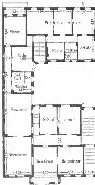
Erdgeschoss. Wohnhaus in der Lessingstraße 38 in Berlin.
