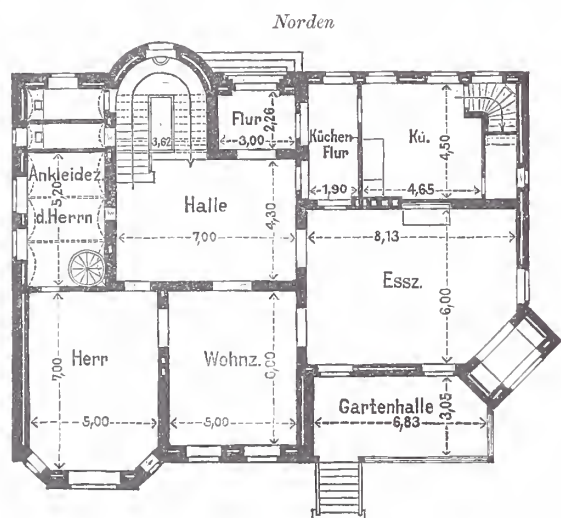
Abb. 2. Erdgeschoss.
