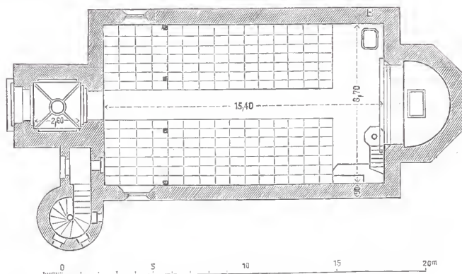
Abb. 2. Grundrifs. Evangelische Kirche in Laufersweiler.
