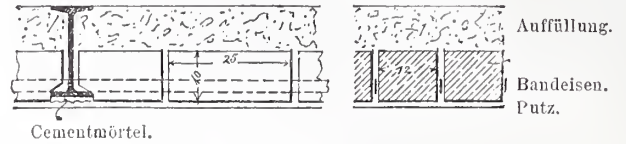
Abb. 1. Decke aus porigen Lochsteinen oder Schwemmsteinen mit eingebettetem Trägerunterflansch (Wohnraumdecke).
