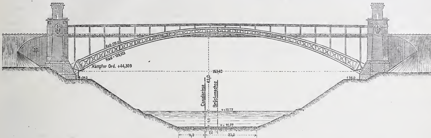
Abb. 5. Ansicht.
