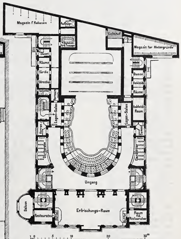
Abb. 3. Grundriß des I. Rang.
