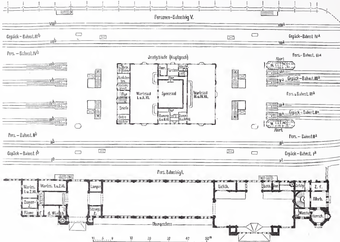
Abb. 4. Grundrifs in Höhe des Bahnsteigs.
