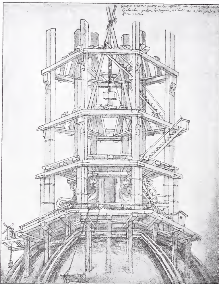
Abb. 1. Das Gerüst für den Bau der Laterne des Florentiner Domes. Original in der Sammlung alter Zeichnungen in den Ufficien. (Aus dem Werke: „v. Stegmann, Architektur der Renaissance in Toscana.“)
