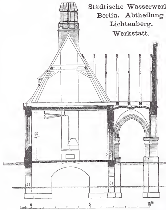
Abb. 14. Schnitt.
