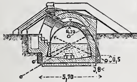
Abb. 8. Schnitt c d.
