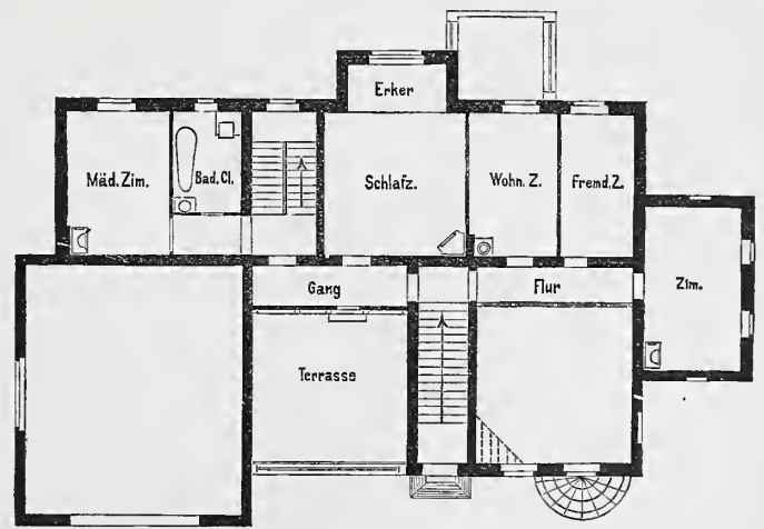
Abb. 4. Obergeschoss.
