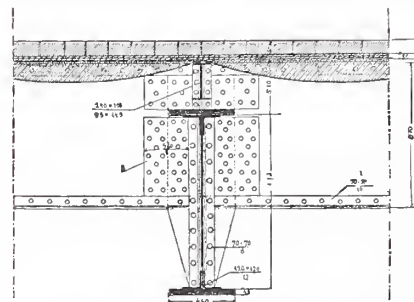
Abb. 12. Längenschnitt der Fahrbahn.
