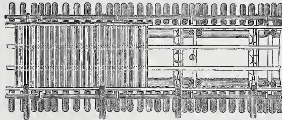
Abb. 5. Grundrifs der Westmole von 256 bis 356 m.
