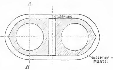
Abb. 6. Grundrifs.
