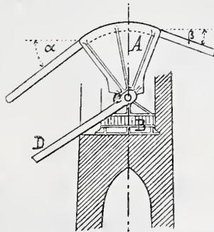
Abb. 7. Auflagerung der Kabel auf den Pylonen. (Erste Anordnung.)
