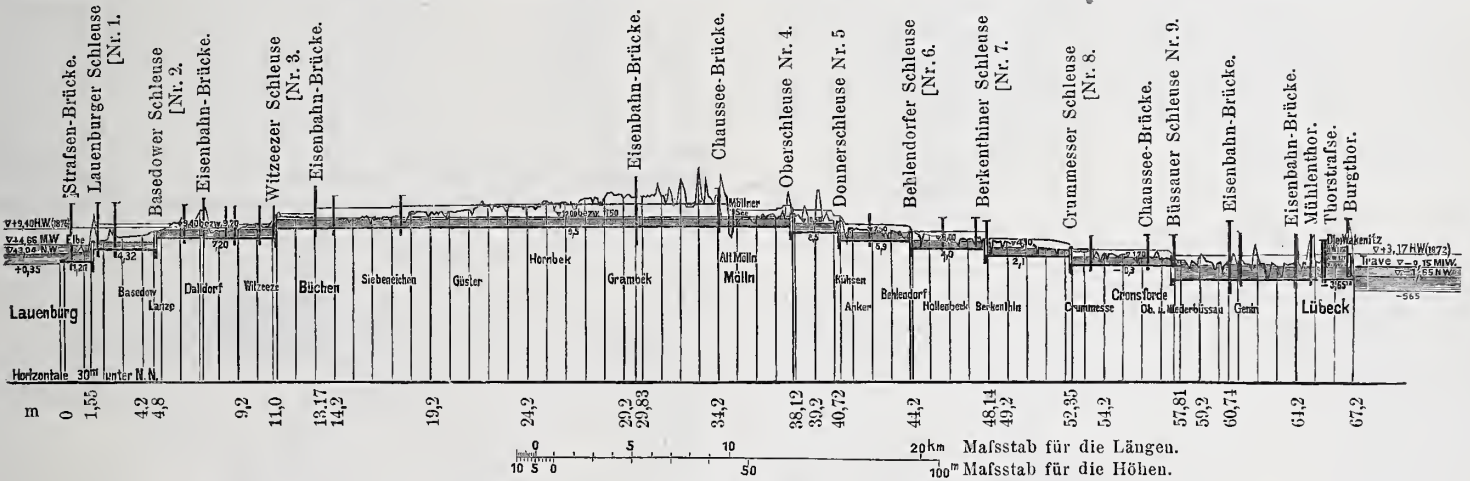
Abb. 2. Längenschnitt.
