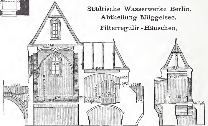
Abb. 8. Schnitte.
