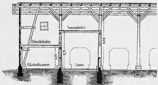
Abb. 6. Längenschnitt.
