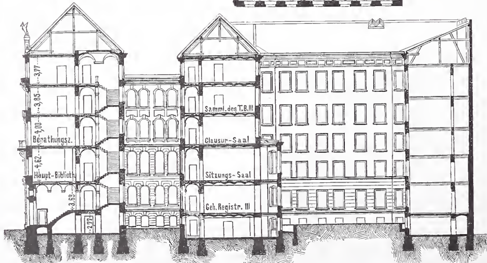
Abb. 3. Schnitt von Süden nach Norden.
