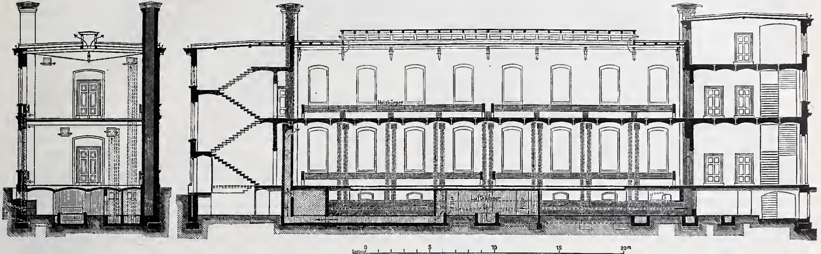
Abb. 10. Schnitt a b.
