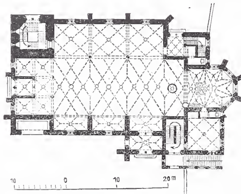
Abb. 4. Grundriss.
