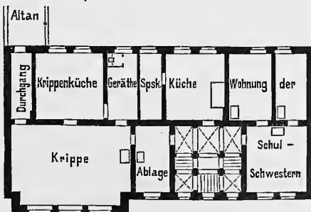
Gemeindehaus für Städte von 10 000—20 000 Einwohnern. (Eingebautes Grundstück.)
