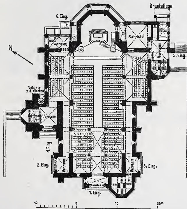
Abb. 1. Grundriss.
