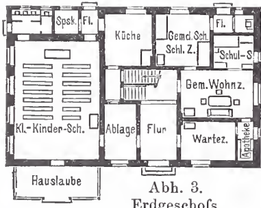
Abb. 3. Erdgeschoss.
