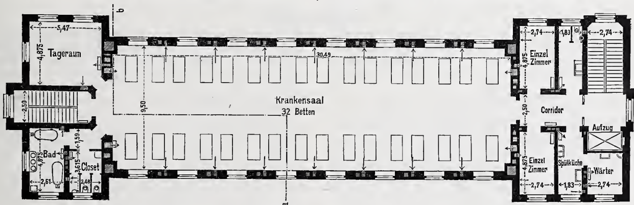
Abb. 12. Erdgeschoss.
