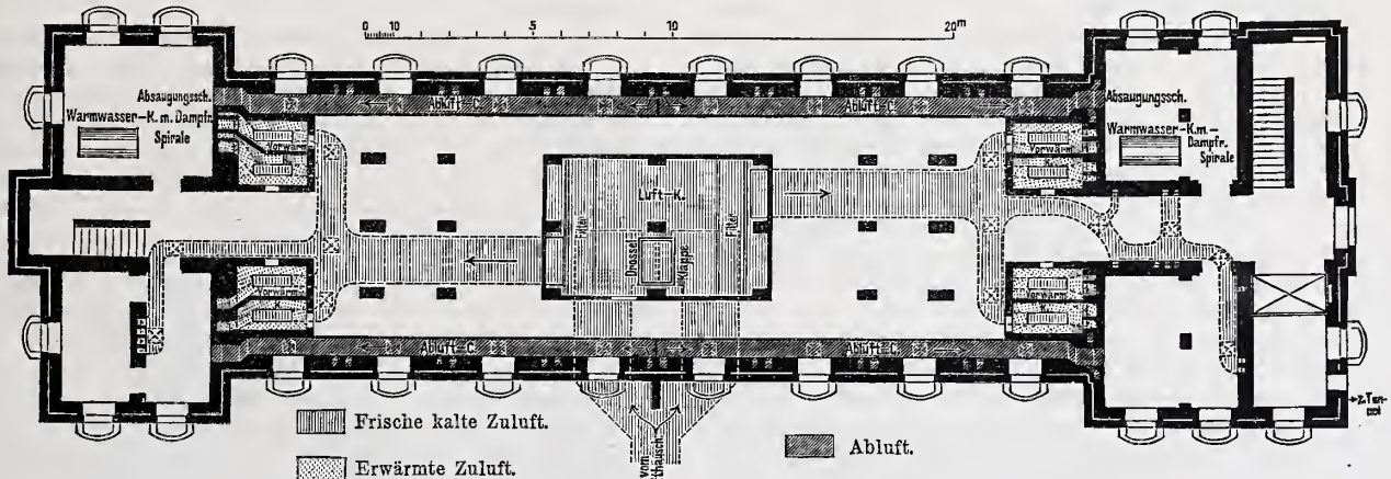
Abb. 13. Keller.
