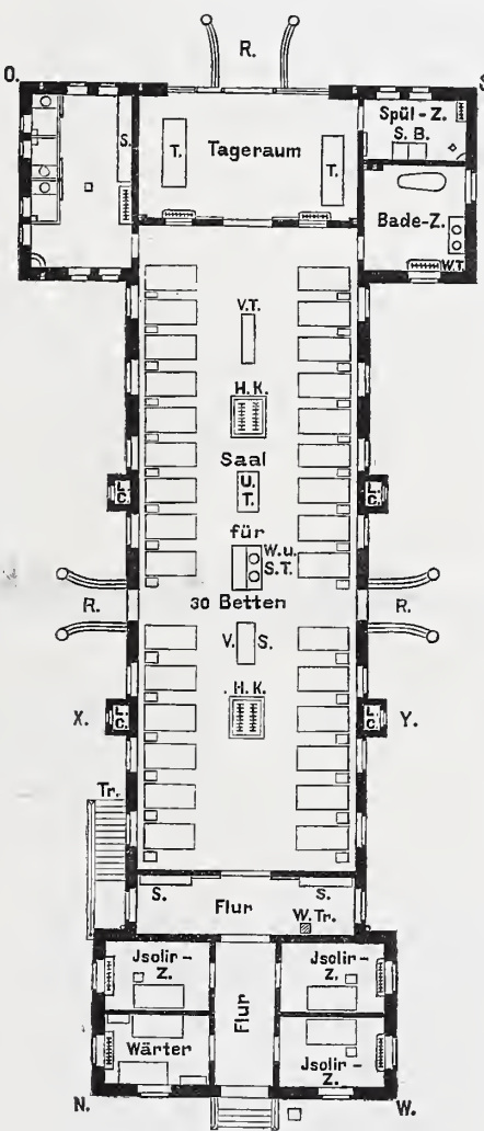
Abb. 5. Erdgeschoss.
