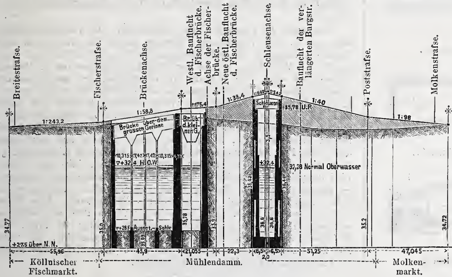
Abb. 3. Höhenplan des Mühlendamms.
