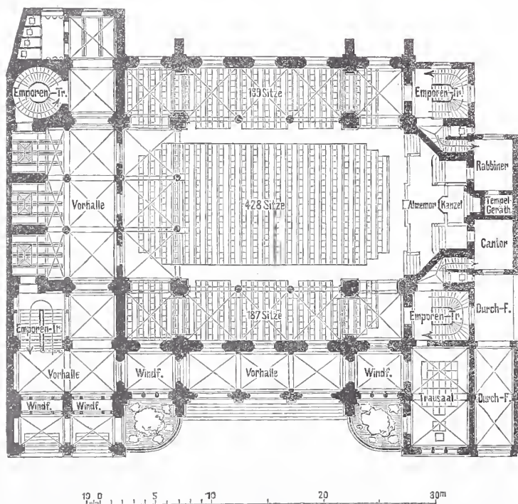
Abb. 2. Entwurf von Schreyer u. Below in Köln. (Erster Preis.) Synagoge für Köln a. Rhein.
