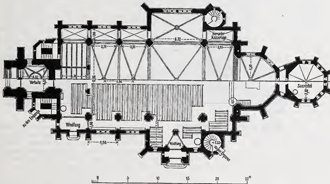
Abb. 1. Grundrißs.
