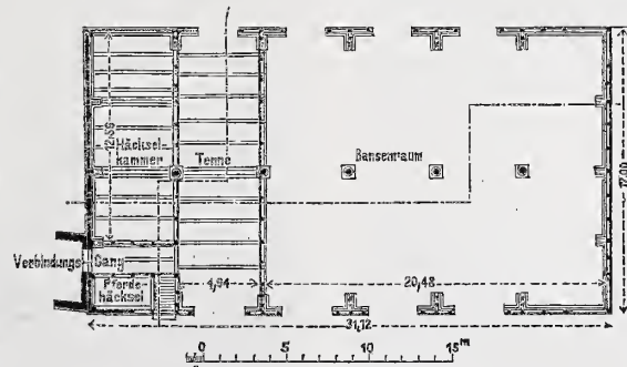
Abb. 4. Grundriss.
