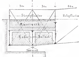
Abb. 11. Anordnung des Gegengewichtes an den Widerlagern.
