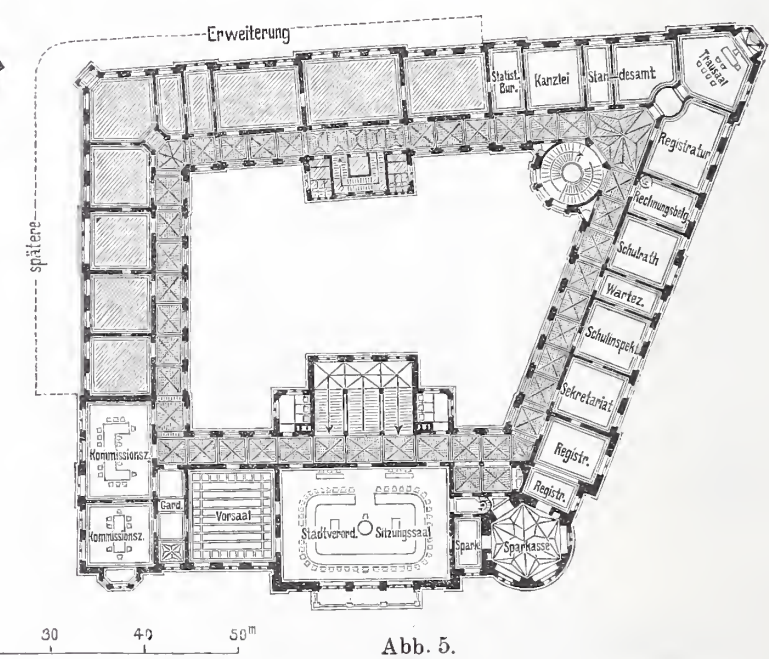
Abb. 5. Entwurf von A. Rofsbach u. Th. Köfser in Leipzig (Ein zweiter Preis). Zweites Obergeschoss.
