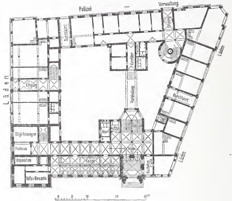
Abb. 9. Entwurf von Emil Schreiterer in Köln (Ein dritter Preis). Erdgeschofs.
