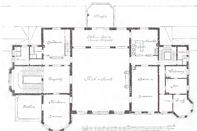
Abb. 3. Obergeschoss.
