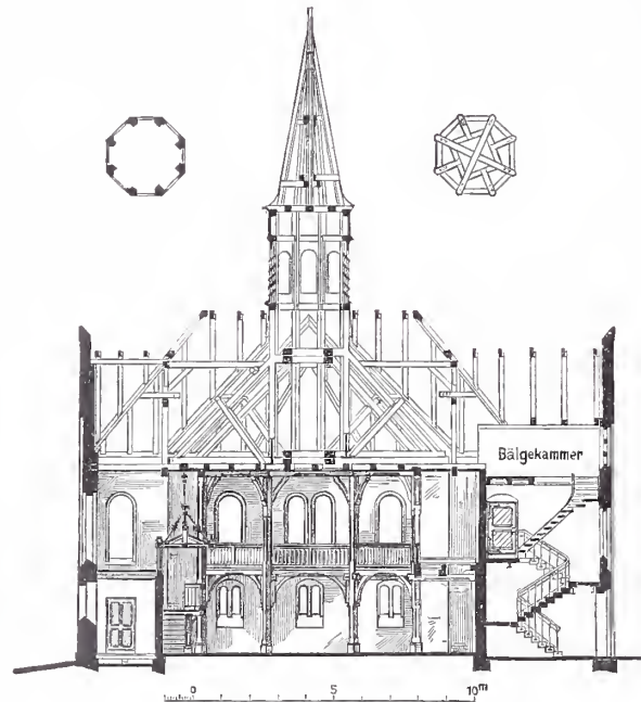
Abb. 3. Schnitt. Evangelische Kirche in Kupp.
