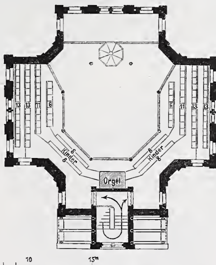
Abb. 2. Grundriss über den Emporen.
