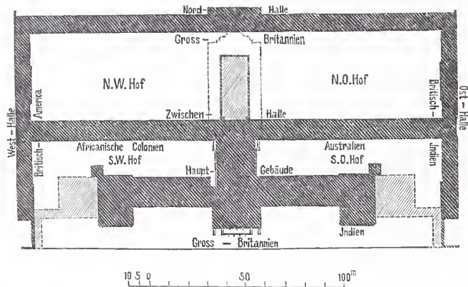
Abb. 1. Gesamtanlage.
