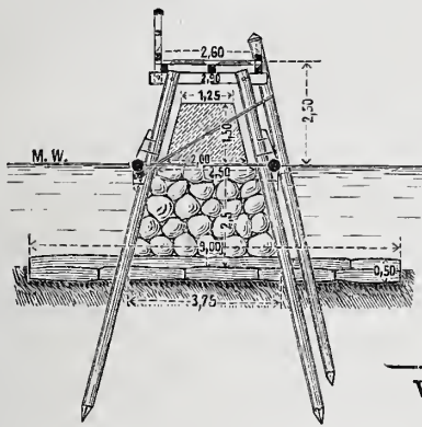
Abb. 2. Querschnitt 1.
