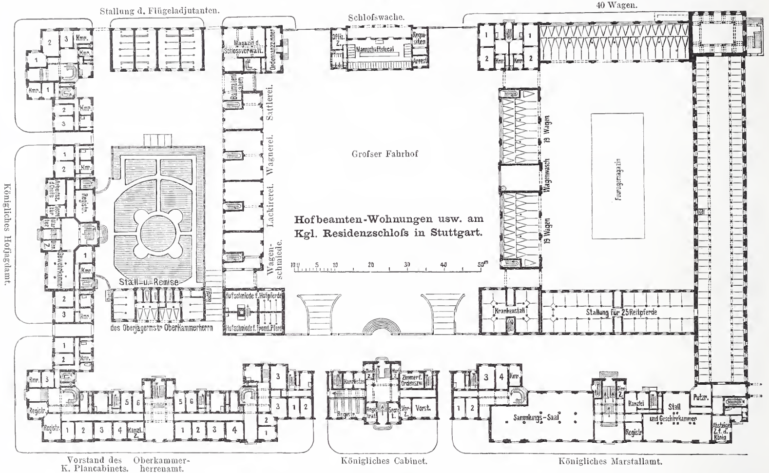
Abb. 7. Grundriß des Erdgeschosses. Entwurf von L. Neher und A. v. Kauffmann in Frankfurt a./M. (III. Preis).
