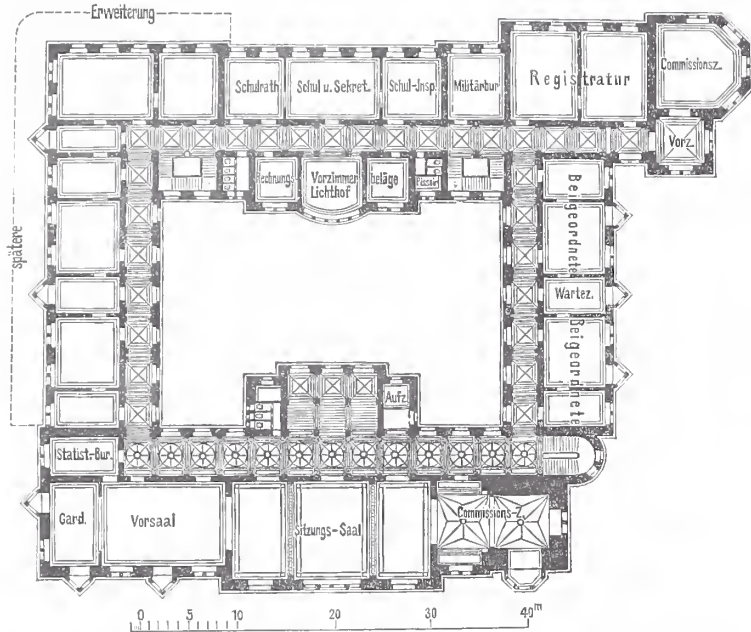
Abb. 8. Entwurf von Polster u. Höhne und Alwin Anger in Leipzig (Ein zweiter Preis). Zweites Obergeschofs.
