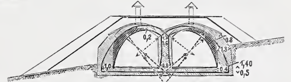
Abb. 9. Querschnitt e f.
