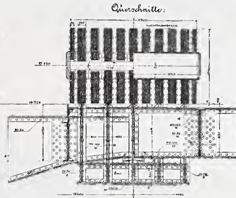
Abb. 30. Das Mittelgelenk der Tragwand.
