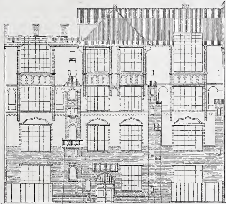
Abh. 5. Ansicht des Ateliergebäudes des Hauses Kurfürstenstr. 126. Berliner Miethshäuser.
