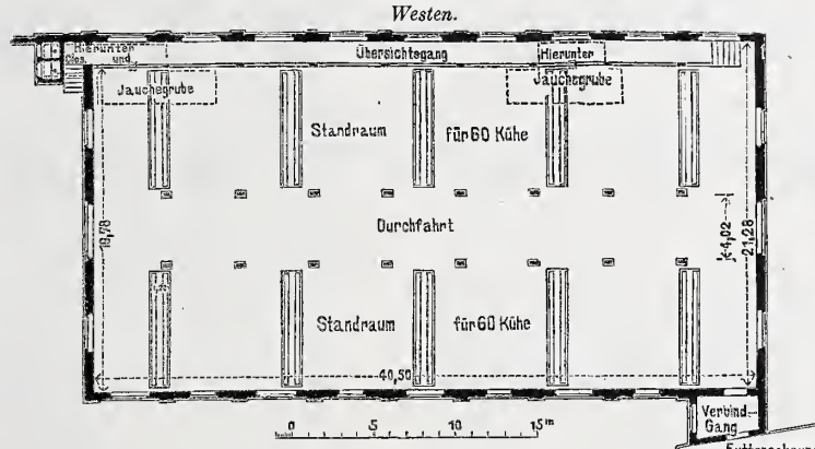
Abb. 1. Grundriss.
