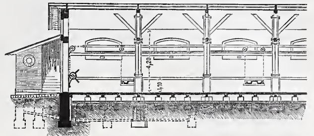
Abb. 3. Längenschnitt.
