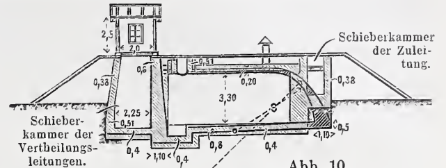
Abb. 10. Längenschnitt g h i k l m.
