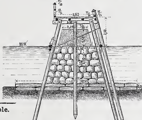
Abb. 3. Querschnitt 2.
