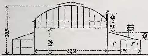
e Schnornstein. f Wohnung des Stationsvorstehers. Abb. 2. Schnitt durch die Halle und die Anbauten.
