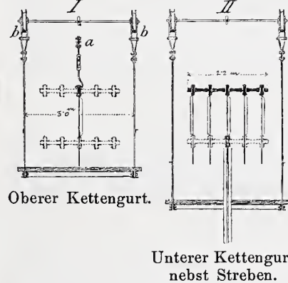
Abb. 34. Aufstellung des Kettengurtes.
