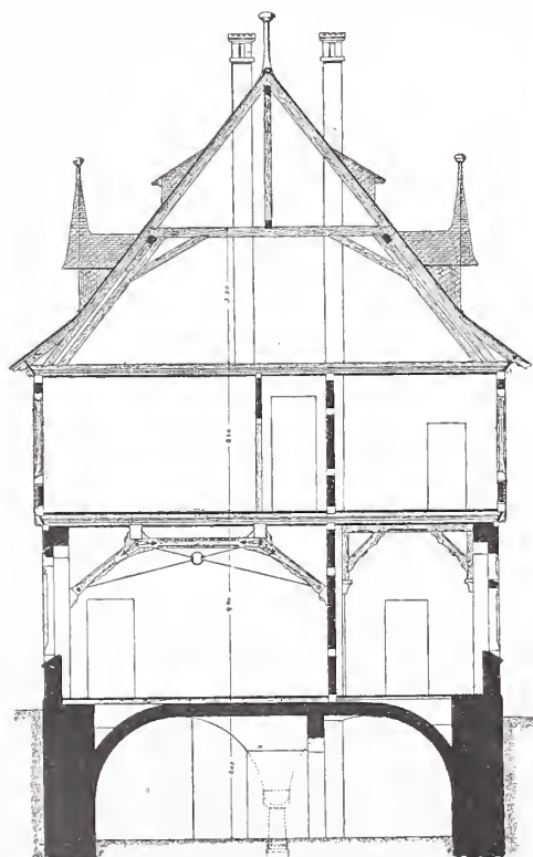
Abb. 2. Querschnitt.
