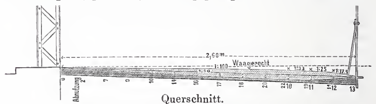
Asphalt-Fufssteig der Strombrücke in Magdeburg.
