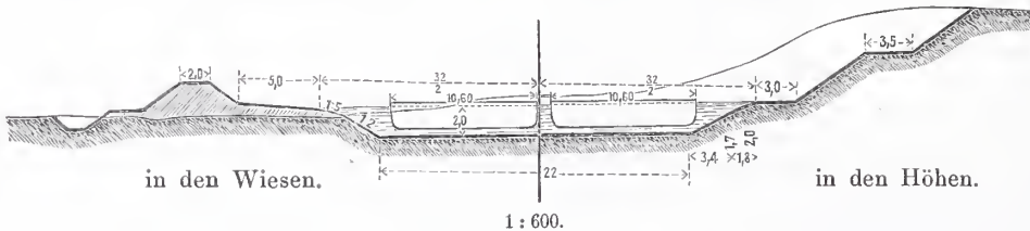
Abb. 4. Querschnitte.
