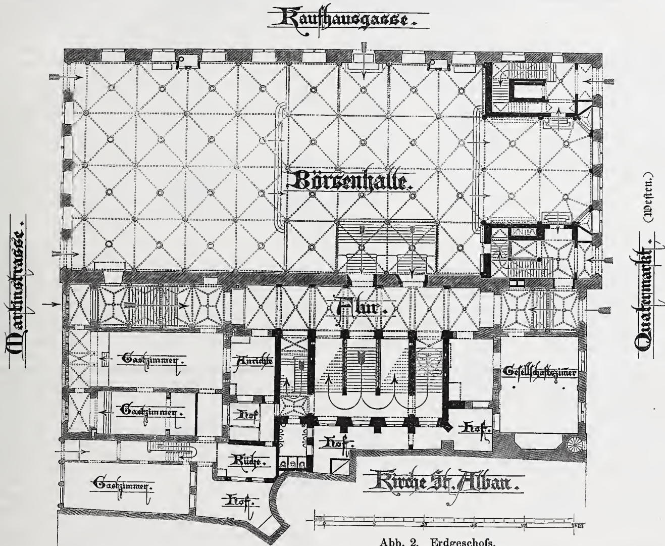
Abb. 2. Erdgeschoss.
