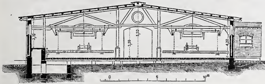
Abb. 2. Querschnitt.
