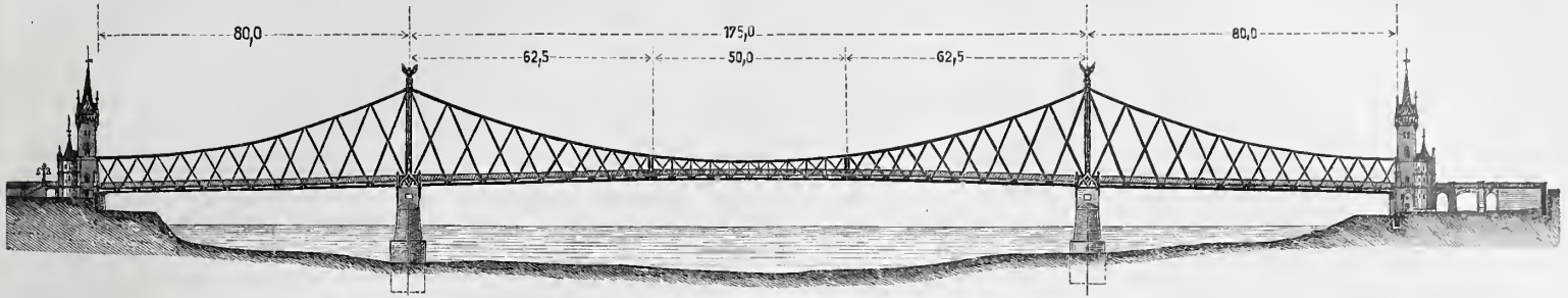
Abb. 14. Ansicht.
