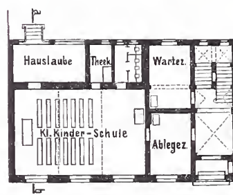
Abb. 8. I. Stockwerk.
