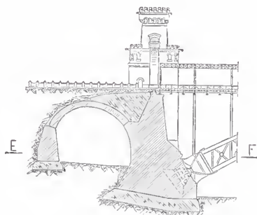
Abb. 2. Schnitt durch das nördliche Widerlager in der Brückenachse.
