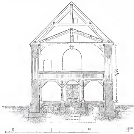
Abb. 1. Querschnitt. Evangelische Kirche in Laufersweiler.
