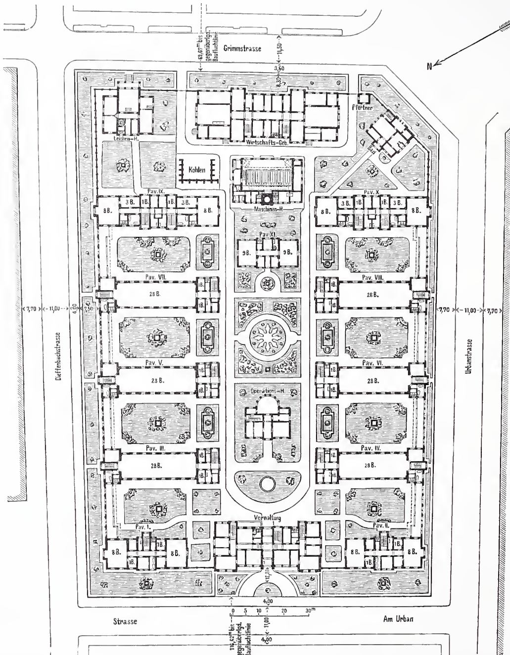
Abb. 9. Lageplan.
