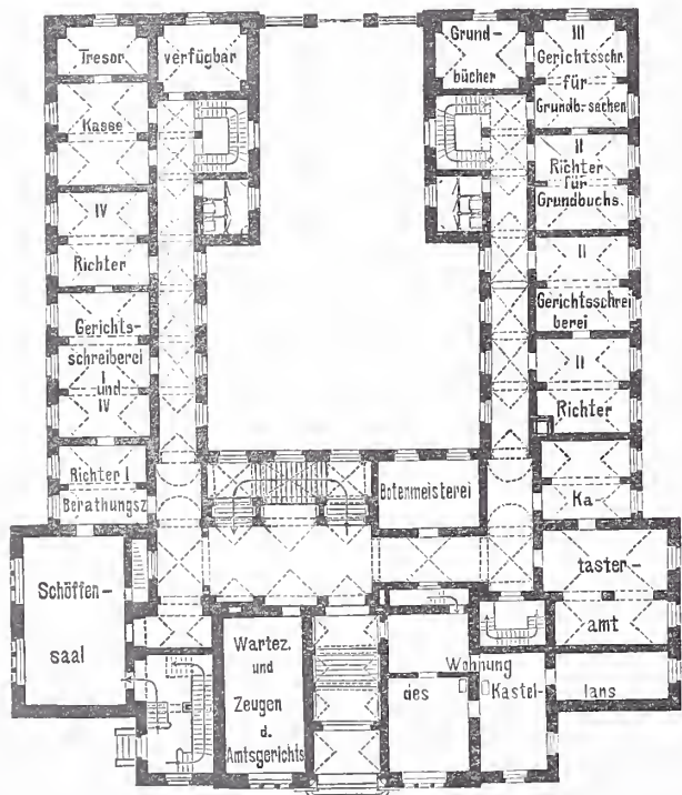
Abb. 3. Erdgeschoss.
