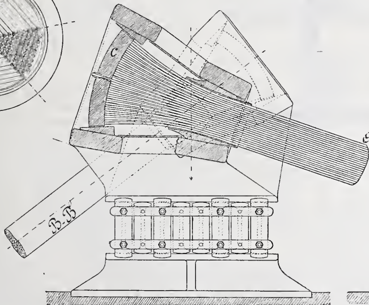
Längenschnitt durch das mittlere Gehäuse.
