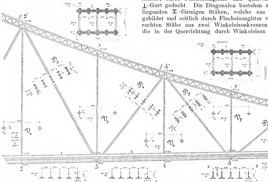
Abb. 29. Construction der Tragwand.
