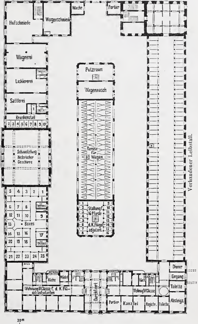
Abb. 6. Erdgeschofs. Gruppe nach dem Marstall hin.
