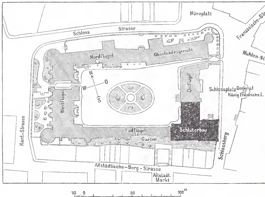
Abb. 1. Lageplan.
