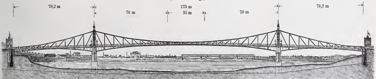
Abb. 9. Hauptzollamtbrücke.
