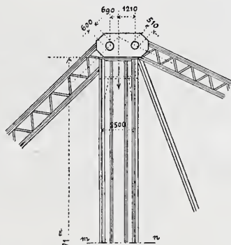
Schnitt mn
