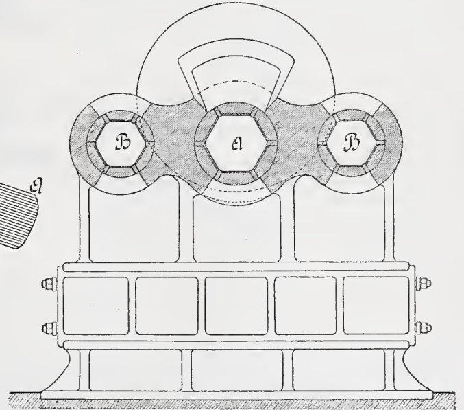
Querschnitt durch die Gehäuse.
