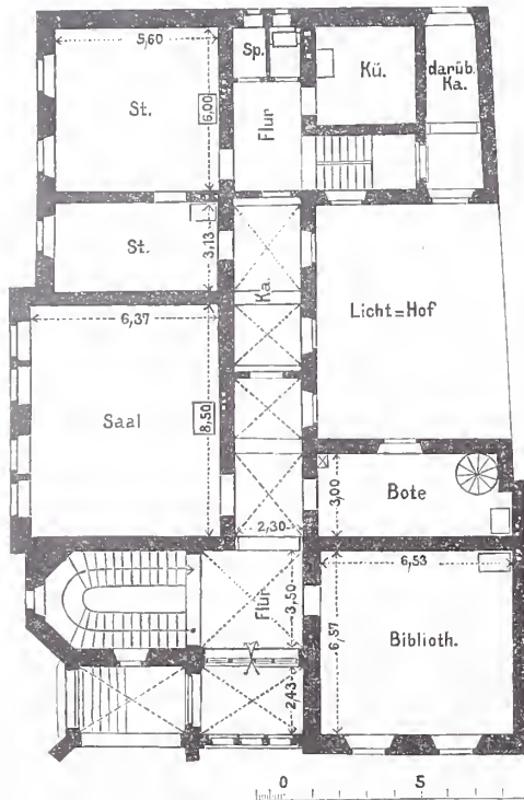
Abb. 1. Erdgeschoss.
