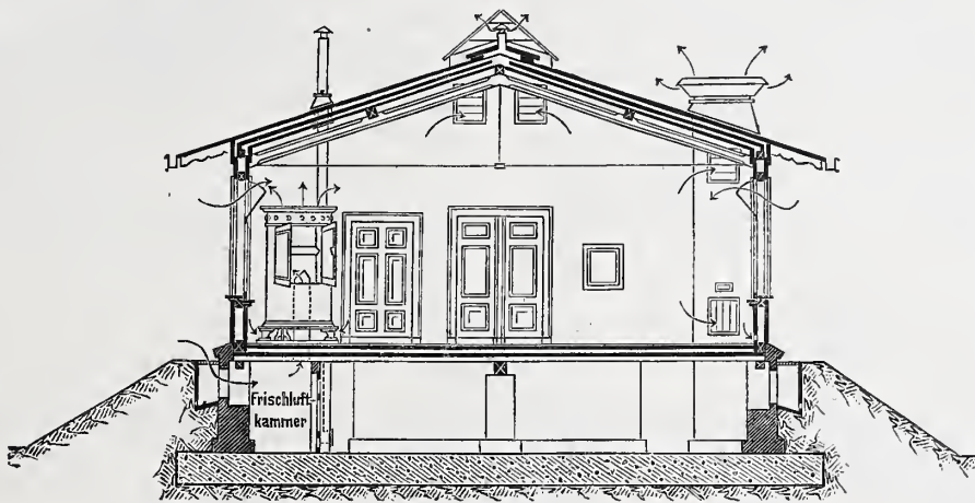
Abb. 7. Schnitt AB in Abb. 8.
