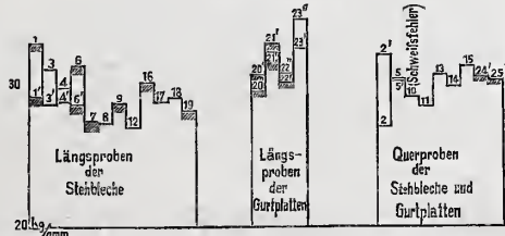
Abb. 2. Elasticitätsgrenze in kg/qmm.
