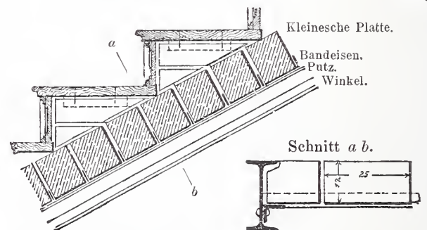
Abb. 9. Massive Treppe nach Kleinescher Bauart.
