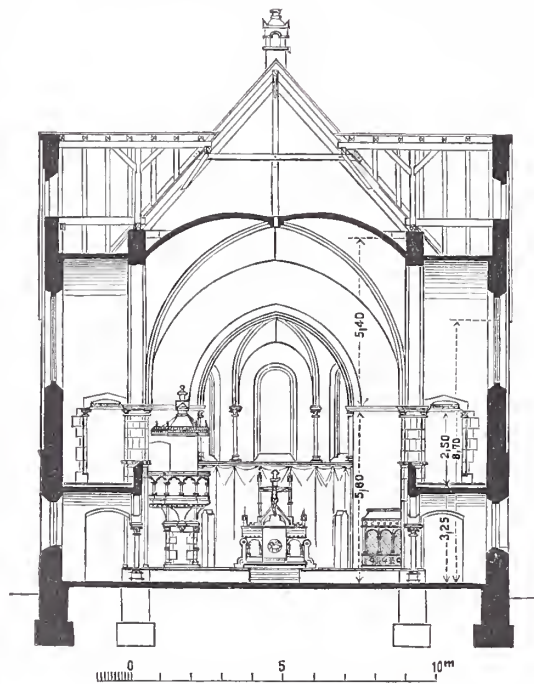
Ahh. 3. Querschnitt.
