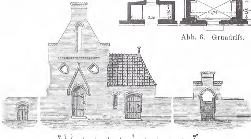
Abb. 7. Ansicht.
