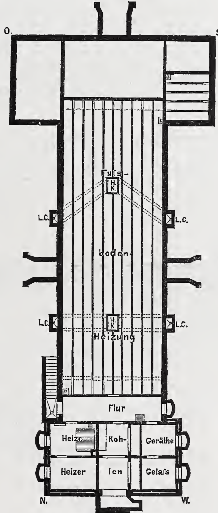
Abb. 4. Kellergeschofs.
