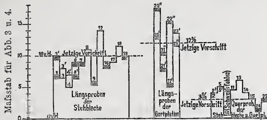
Abb. 3. Bruchdehnung.
