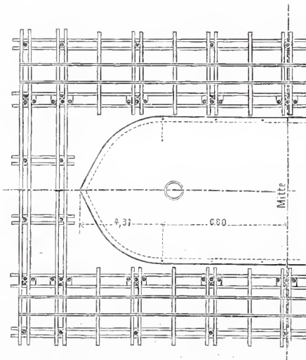
Abb. 9. Grundrifs.
