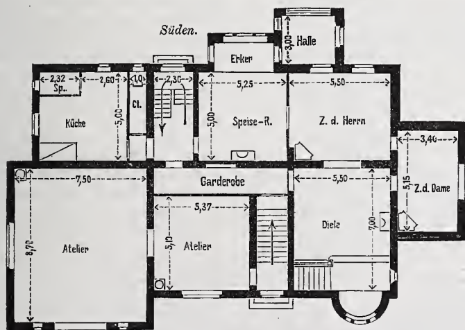
Abb. 3. Erdgeschoss.
