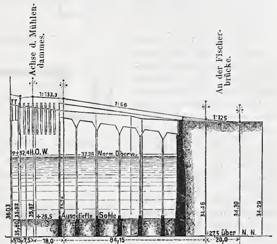
Abb. 4. Höhenplan der Fischerbrücke.
