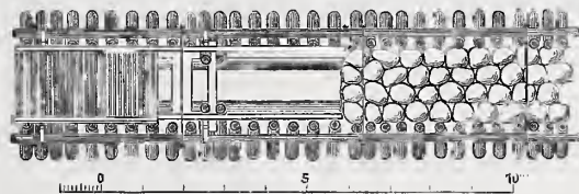
Abb. 6. Grundrifs der Ostmole.
