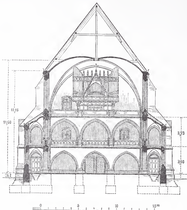
Abb. 2. Querschnitt.
