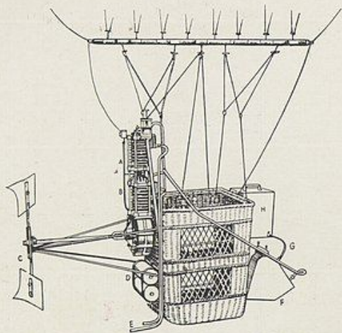
A B. Moteurs superposés. — C. Hélice. — D. Bobines. — E. Tubes d'échappement F. Carburateur. — G. Tube d'admission. — H. Réservoir à essence. La nacelle et le moteur.
