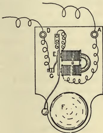
FIG. 354—ELECTRIC BELL
