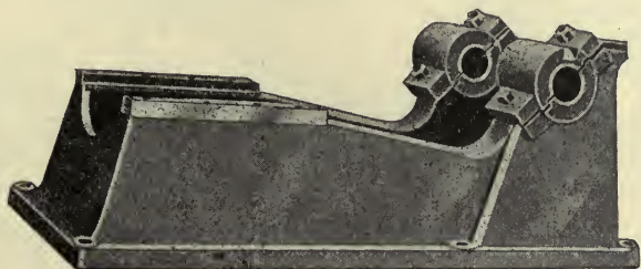
FIG. 291—BASE
