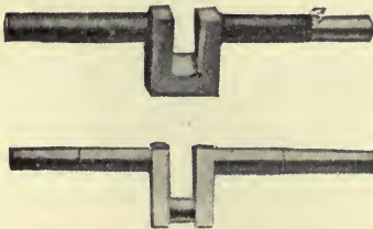
FIG. 294—CRANK SHAFT
