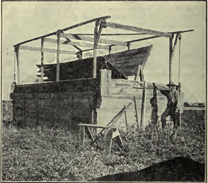
FIG. 202—HOME-MADE JUMBO
