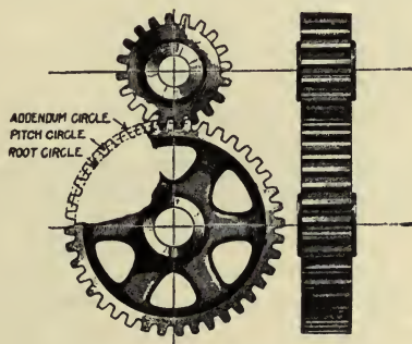
FIG. 24—SPUR GEARING
