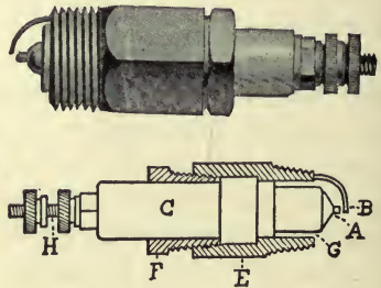
FIG. 307—JUMP-SPARK IGNITOR
