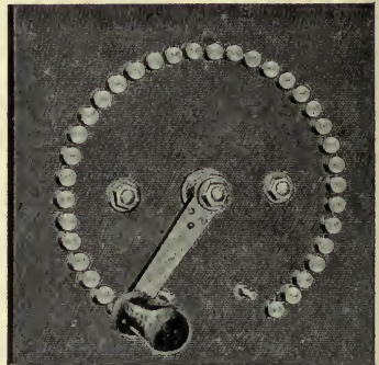
FIG. 348—PRINCIPLE OF RHEOSTAT FIG. 349—COMMERCIAL RHEOSTAT
