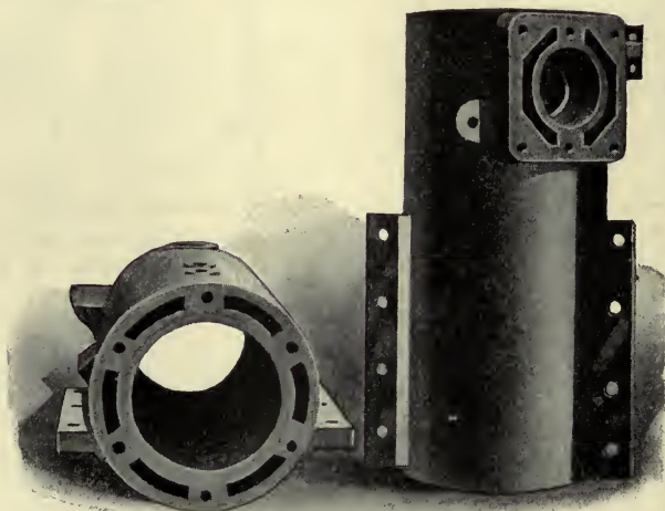
FIG. 290—CYLINDER
