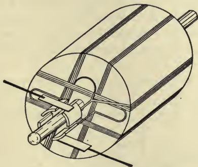
FIG. 362—DRUM ARMATURE
