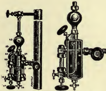
FIG. 279—CYLINDER LUBRICATOR
