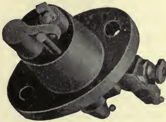
FIG. 306—CONTACT-SPARK IGNITOR
