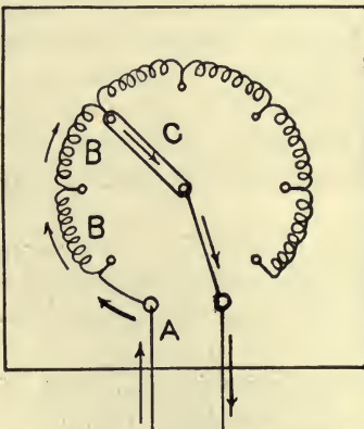
FIG. 348—PRINCIPLE OF RHEOSTAT FIG. 349—COMMERCIAL RHEOSTAT
