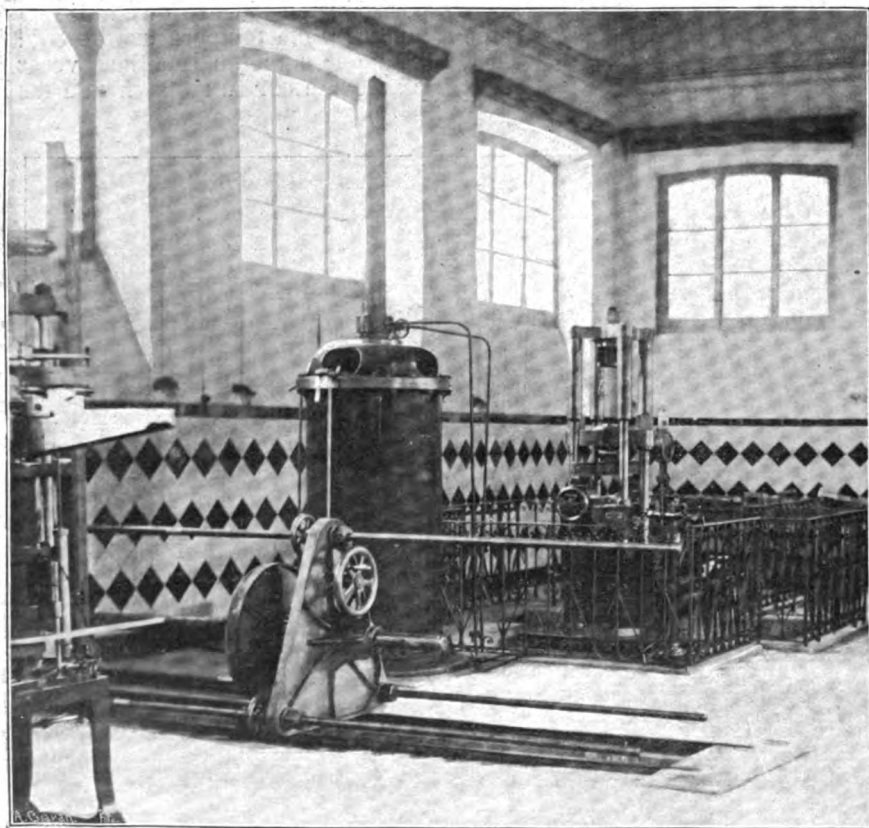
SS. MM. visitando el Laboratorio (de fotografía de Cao). — Máquina Falcot, universal, de 100 toneladas. — Máquina Falcot de 15 toneladas. Prensa de 100 toneladas Heindr. Ehrhardt y prensa hidráulica para tubos. — Máquina Amsler Laffon, universal, de 200 toneladas.
