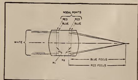
FIG. 22. Lateral chromatism. I.
