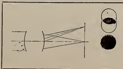
FIG. 24. Vignetting.
