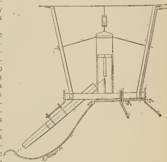
Fig. 3. - Esquema del aparato para luz eléctrica
