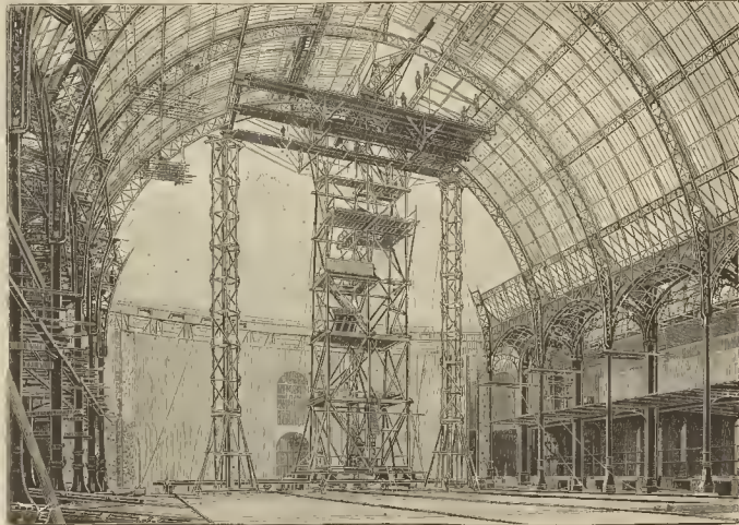
Fig. 1. - Montaje de los cuchillos de armadura
