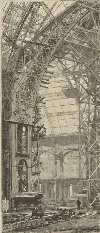
Fig. 2. - Arranque de uno de los cuchillos de armadura y de una armadura de enlace
