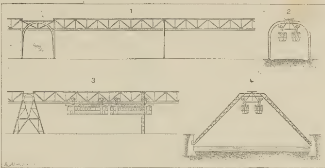
Fig. 4. — Modos de suspensión y disposición en la calle y sobre el río. — 1. Vista de lado en la calle. — 2. Sección transversal. — 3. Construcción sobre el río: vista de lado. — 4. Sección transversal
