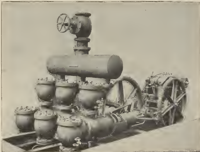
Fig. 1. - Bomba eléctrica para extracción del agua
