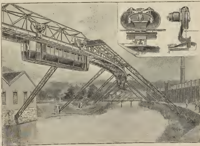
Fig. 3. - Vista en conjunto de una parte de la vía construída cerca de Elberfeld sobre el río Wupper. En el cartucho, sistema de suspensión y disposición de los bastidores
