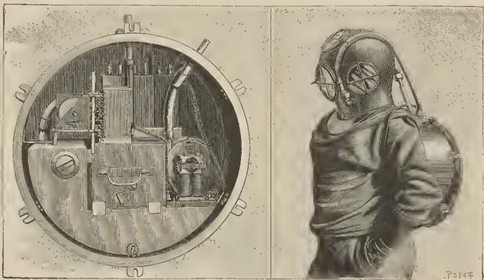
APARATO DESGREZ Y BALTHAZARD. - Vista interior: caja distributriz; motor eléctrico, ventilador, depósito de agua. Vista en conjunto: individuo vestido con el escafiandro y el aparato regenerador del aire viciado
