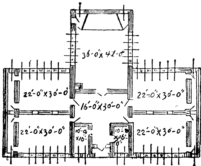
四 教 室 校 舍 平 面 圖
