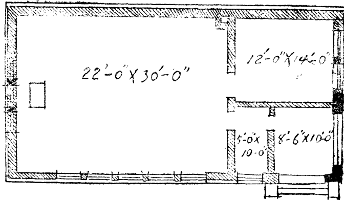
單 教 室 校 舍 平 面 圖
