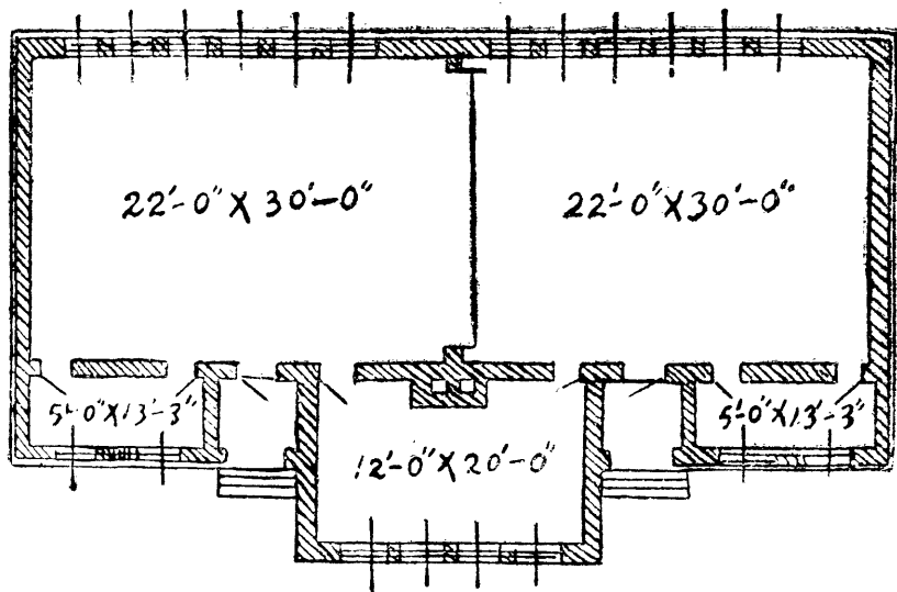
兩 教 室 校 舍 平 面 圖
