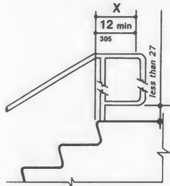
(d) Extension at Top of Run
