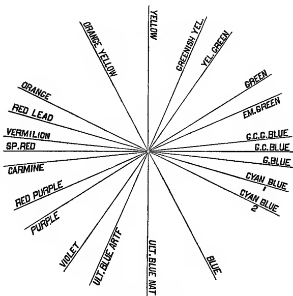
FIG. 181.—Contrast Diagram.
