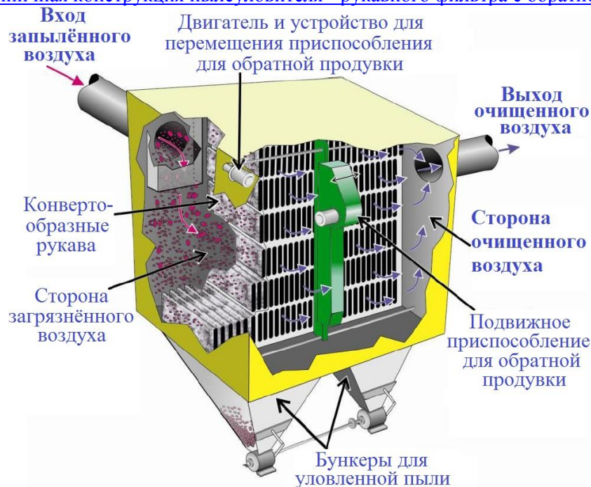
Рис. 1.18 Типичная конструкция пылеуловителя - рукавного фильтра с обратной продувкой
