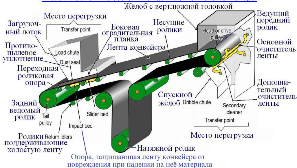
Рис. 5.1. Основные составные части ленточного конвейера.
