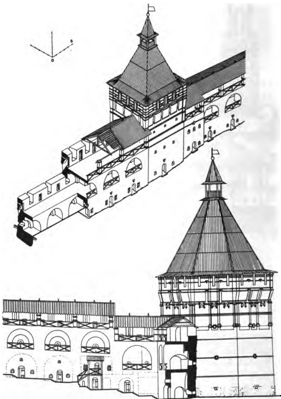
Крепостная стена с башней. Схема стронтельных этапов XVI—XVII вв.
