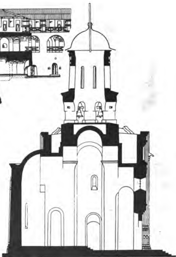
Духовская церковь. 1476. Разрез. Реконструкция В. Балдина
