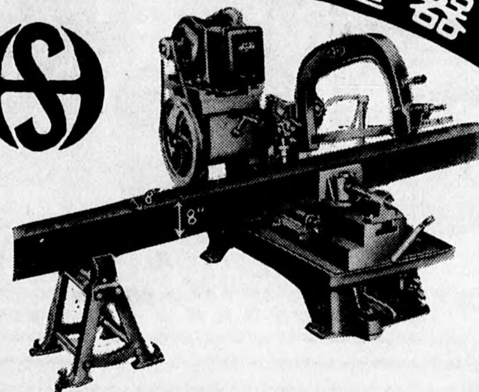
H.S式高速金切鋸機 (A型8"×8"自動電磁閉器付二段變速)
