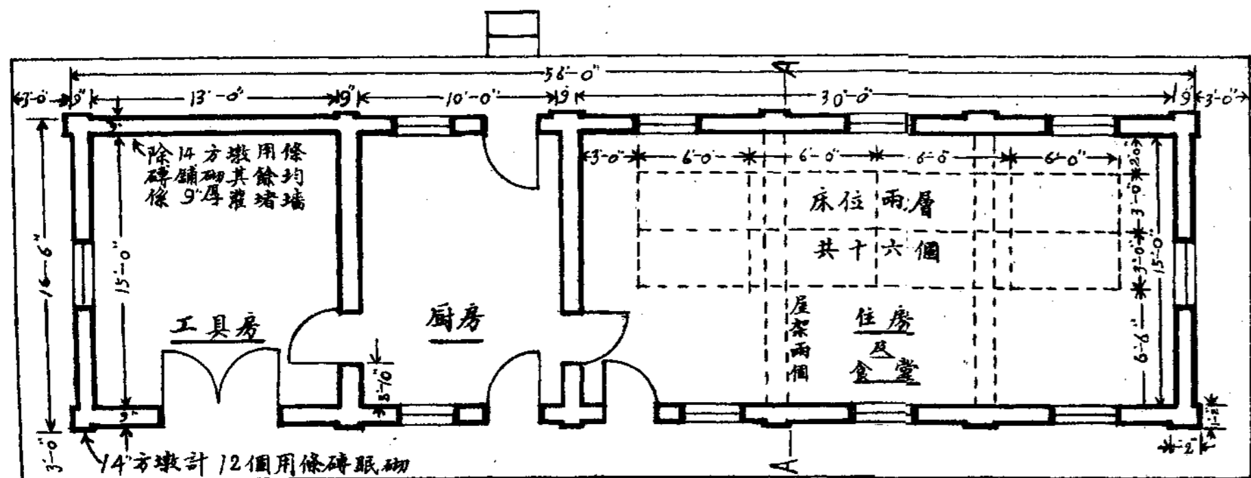
平面圖
