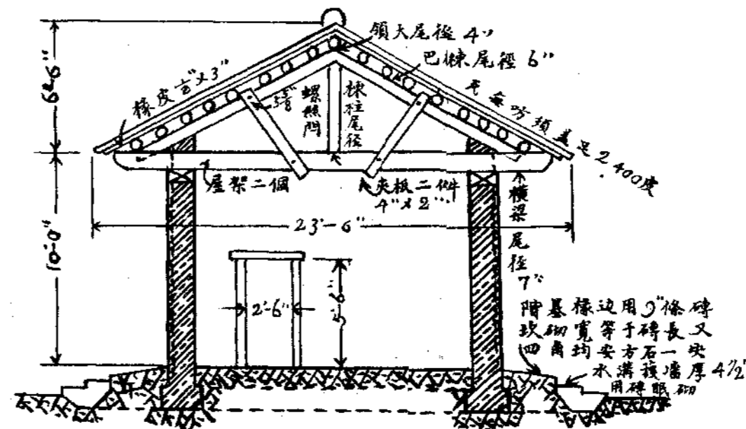
斷面 AA
