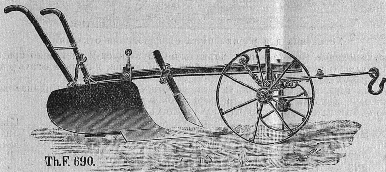
Видъ плуга съ переставнымъ передкомъ.
