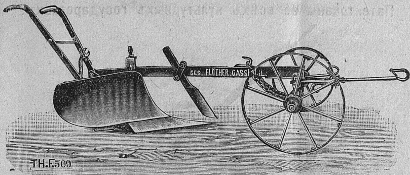
Видъ плуга съ обыкновеннымъ передкомъ.
