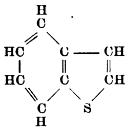
Thionaphthene.
