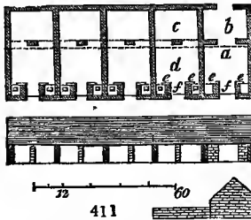
2831. Cattle-hammels (fig. 411.)
