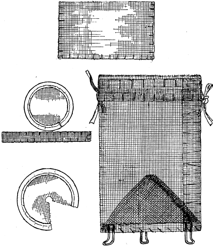
FIG. 22.—Fly trap.
