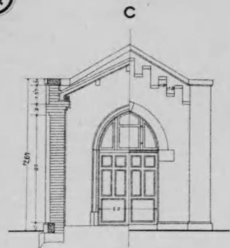
入口詳細圖
