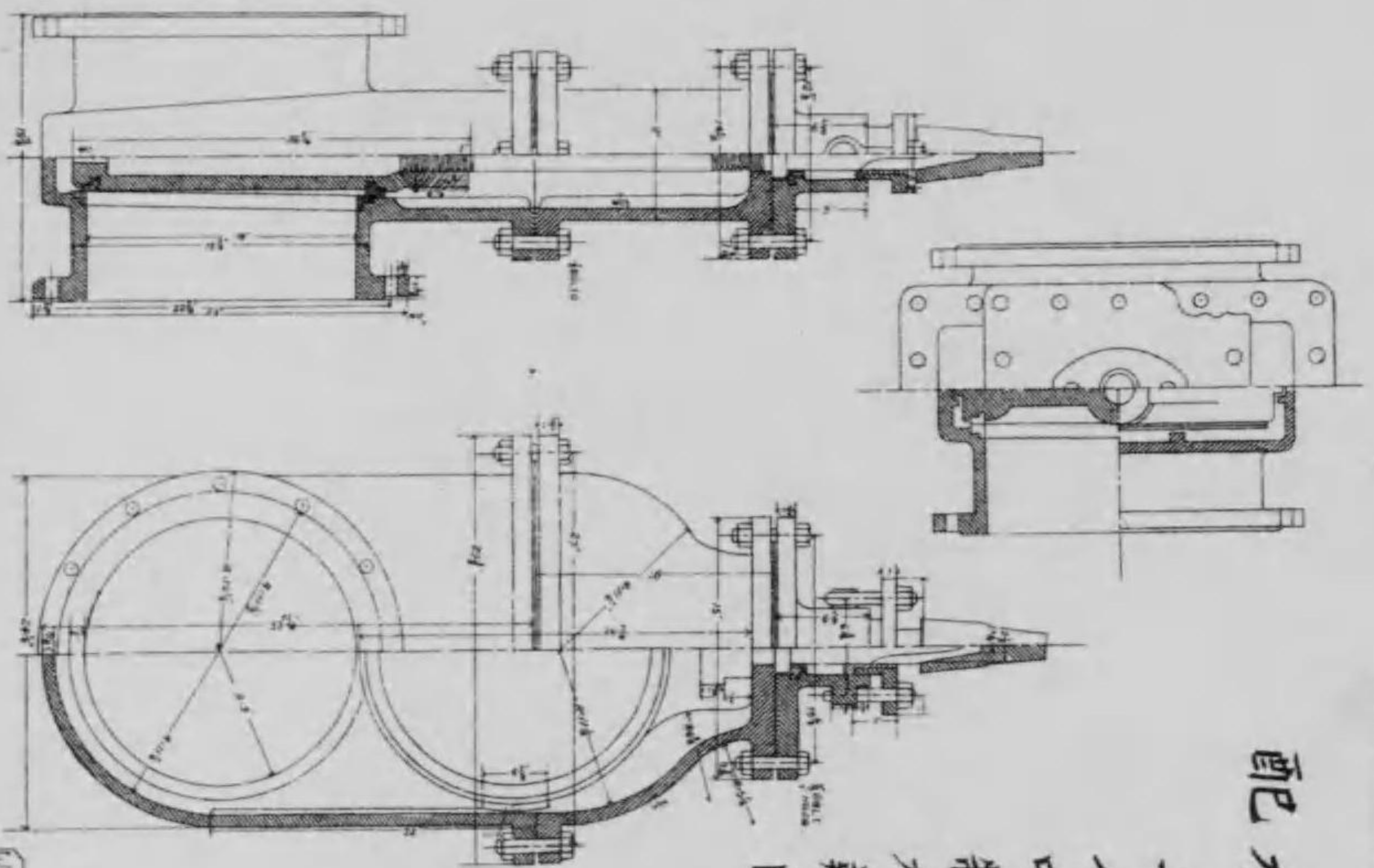
十八吋制水瓣圖
