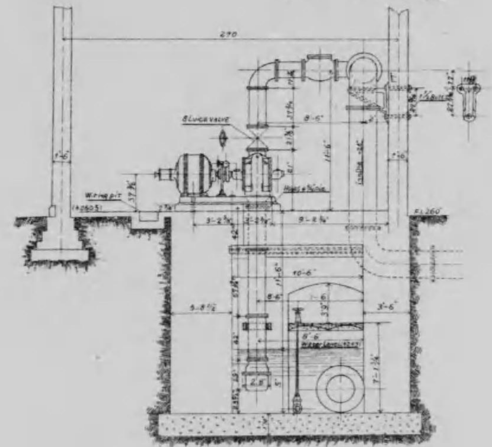
圖斷橫
