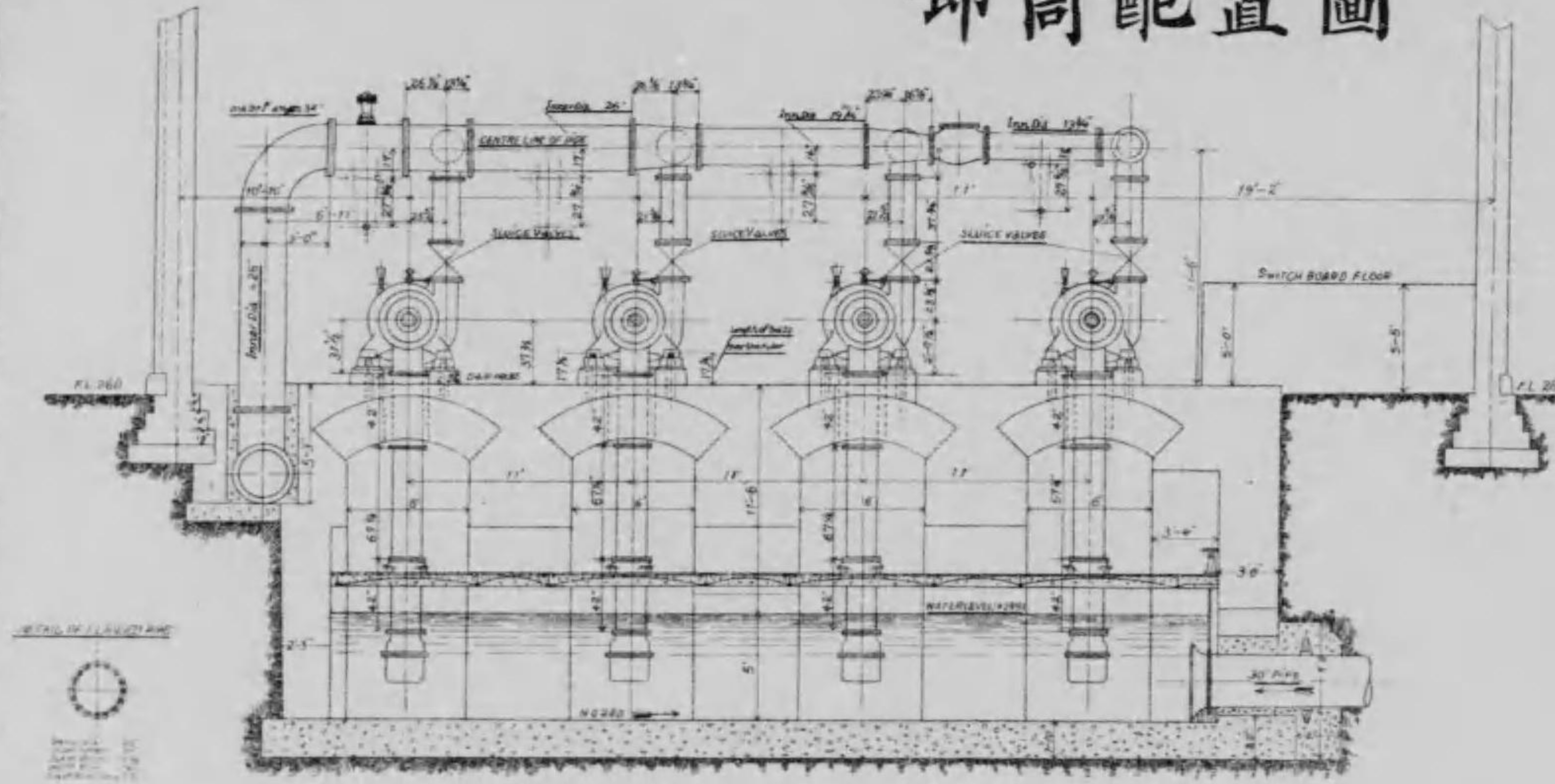
縱斷圖
