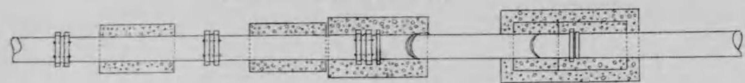
縱断面詳細圖
