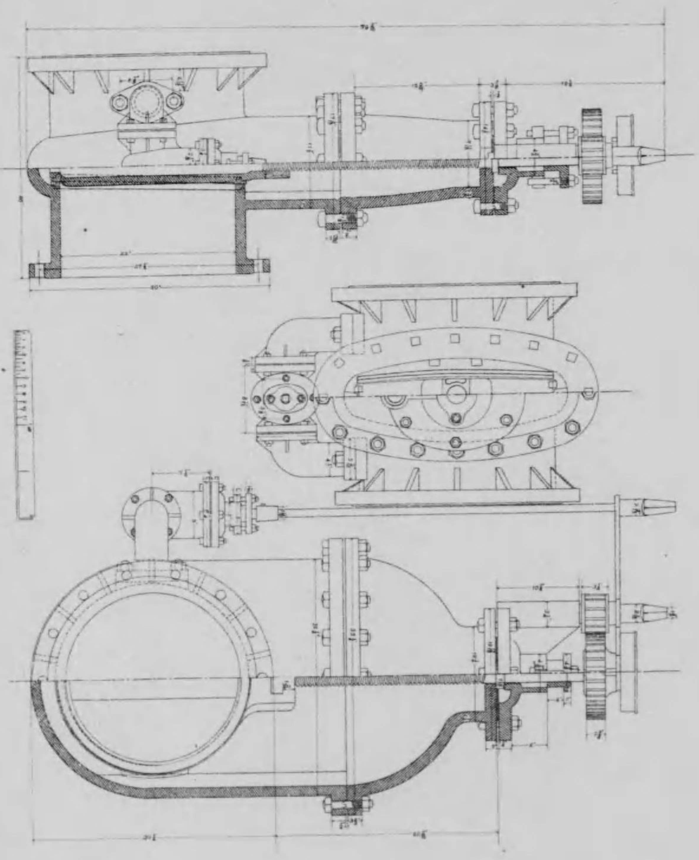
二十二吋制水瓣圖
