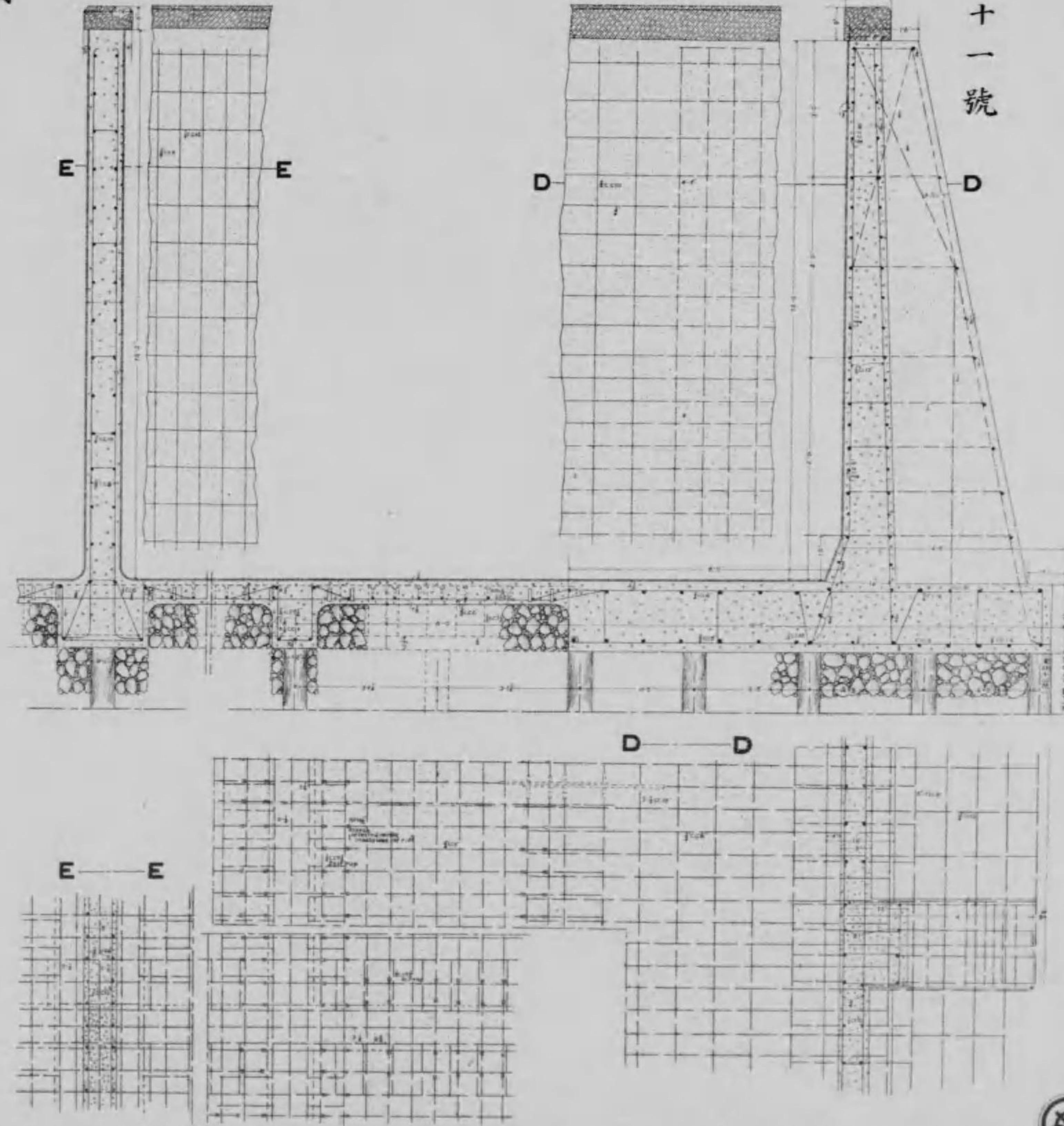
側壁圖
