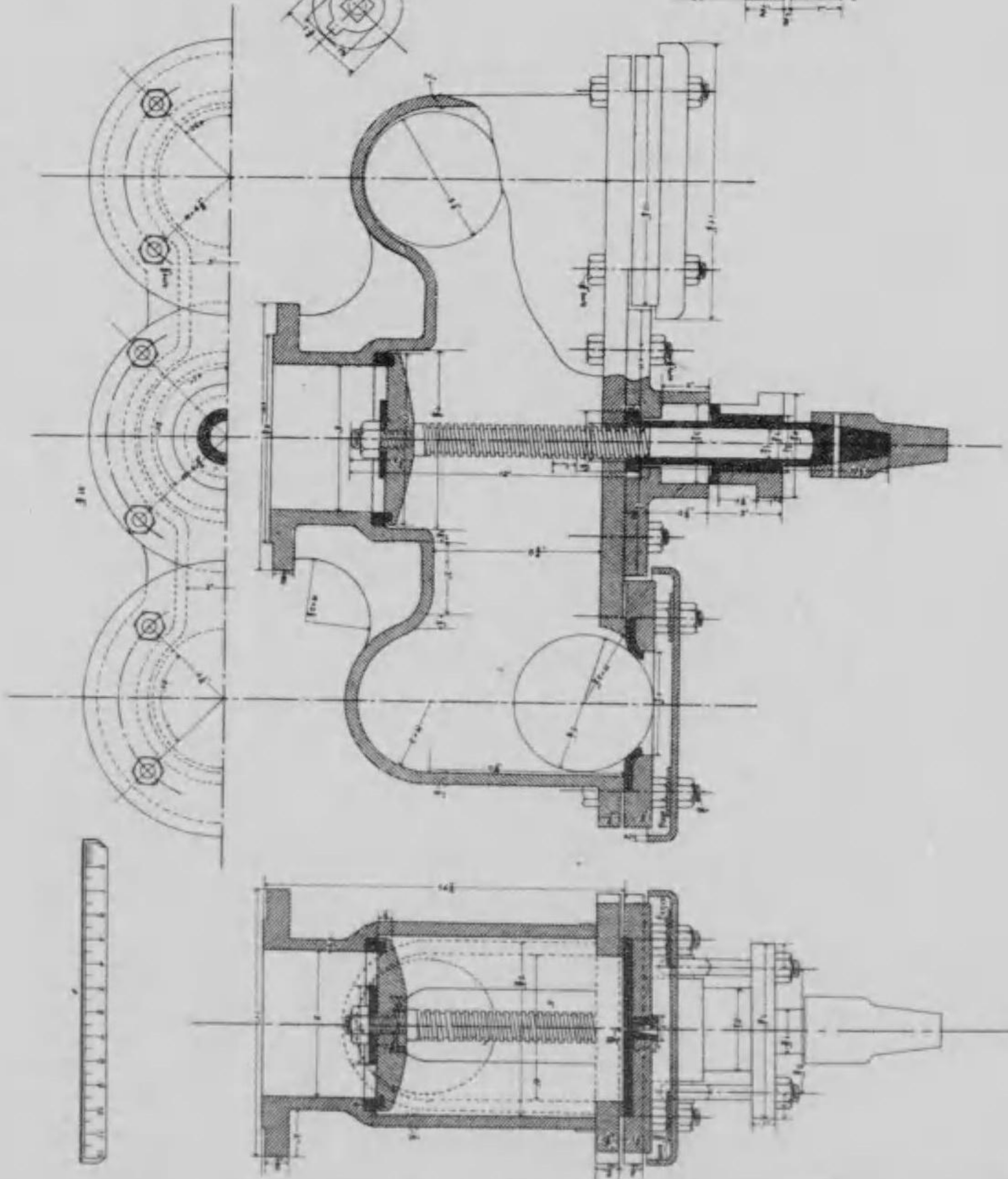
六吋排氣瓣圖
