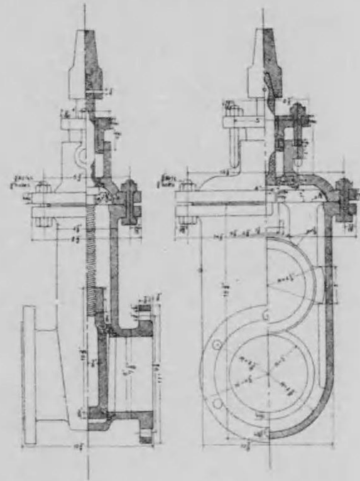
六吋制水瓣圖
