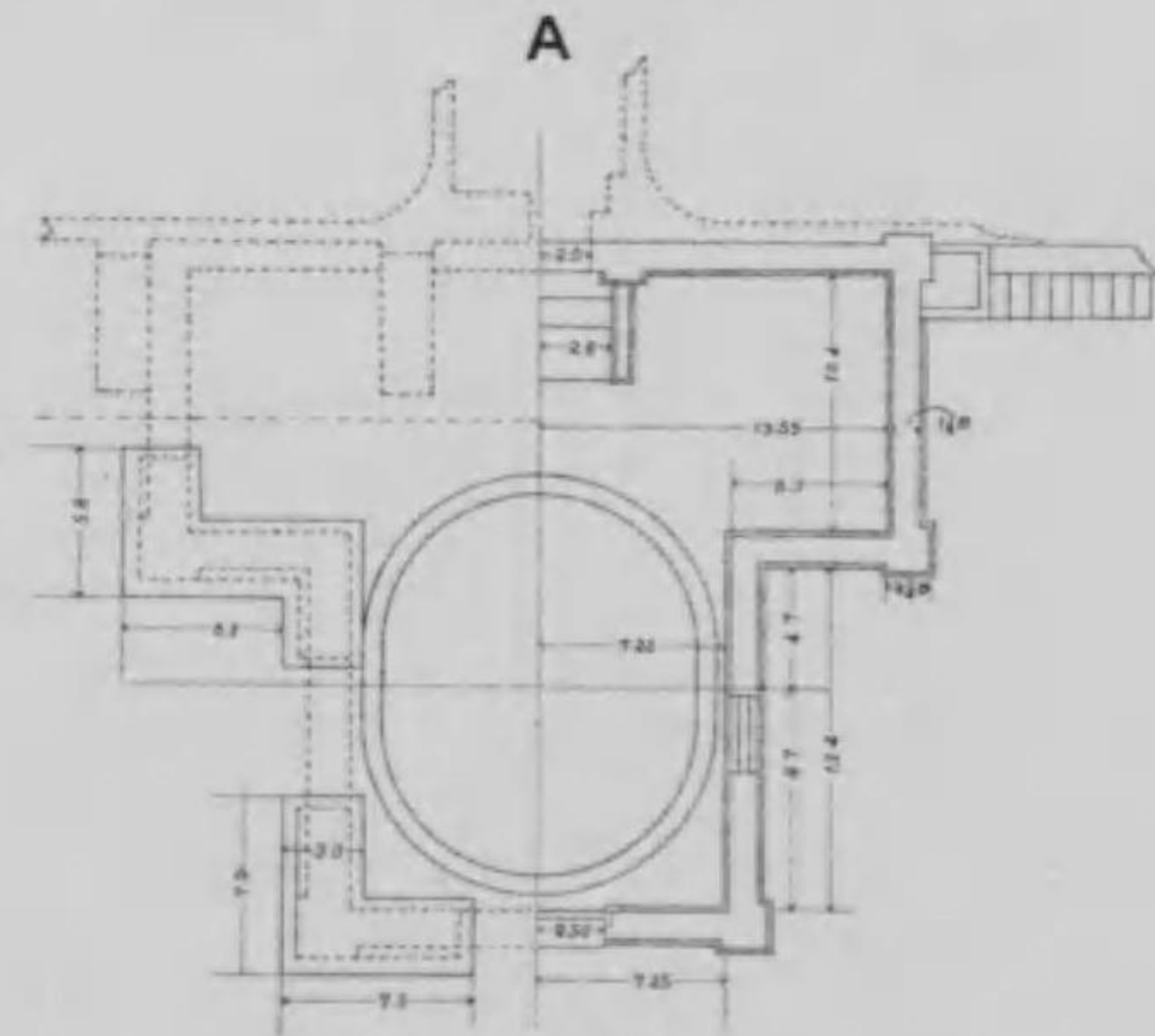
出口平面圖
