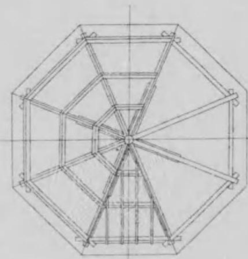
家根平面圖
