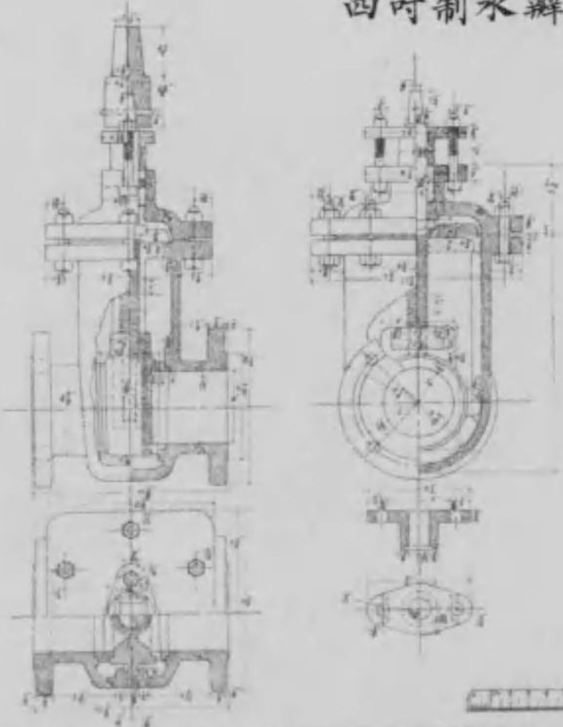
四吋制水瓣圖
