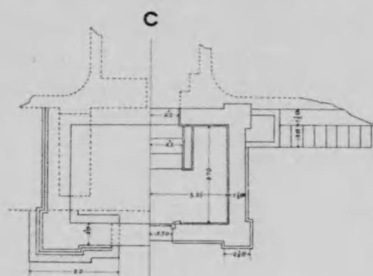
入口平面圖
