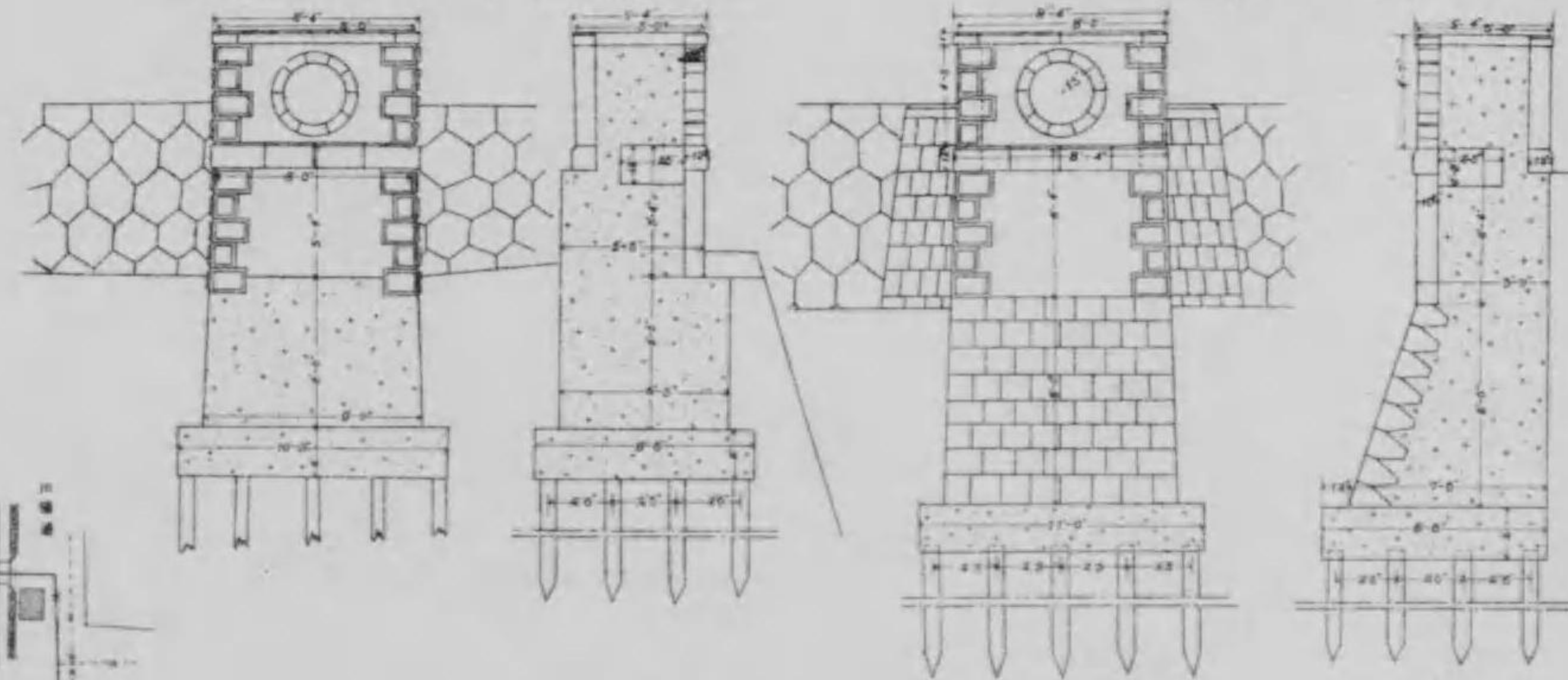
運河西側橋台
