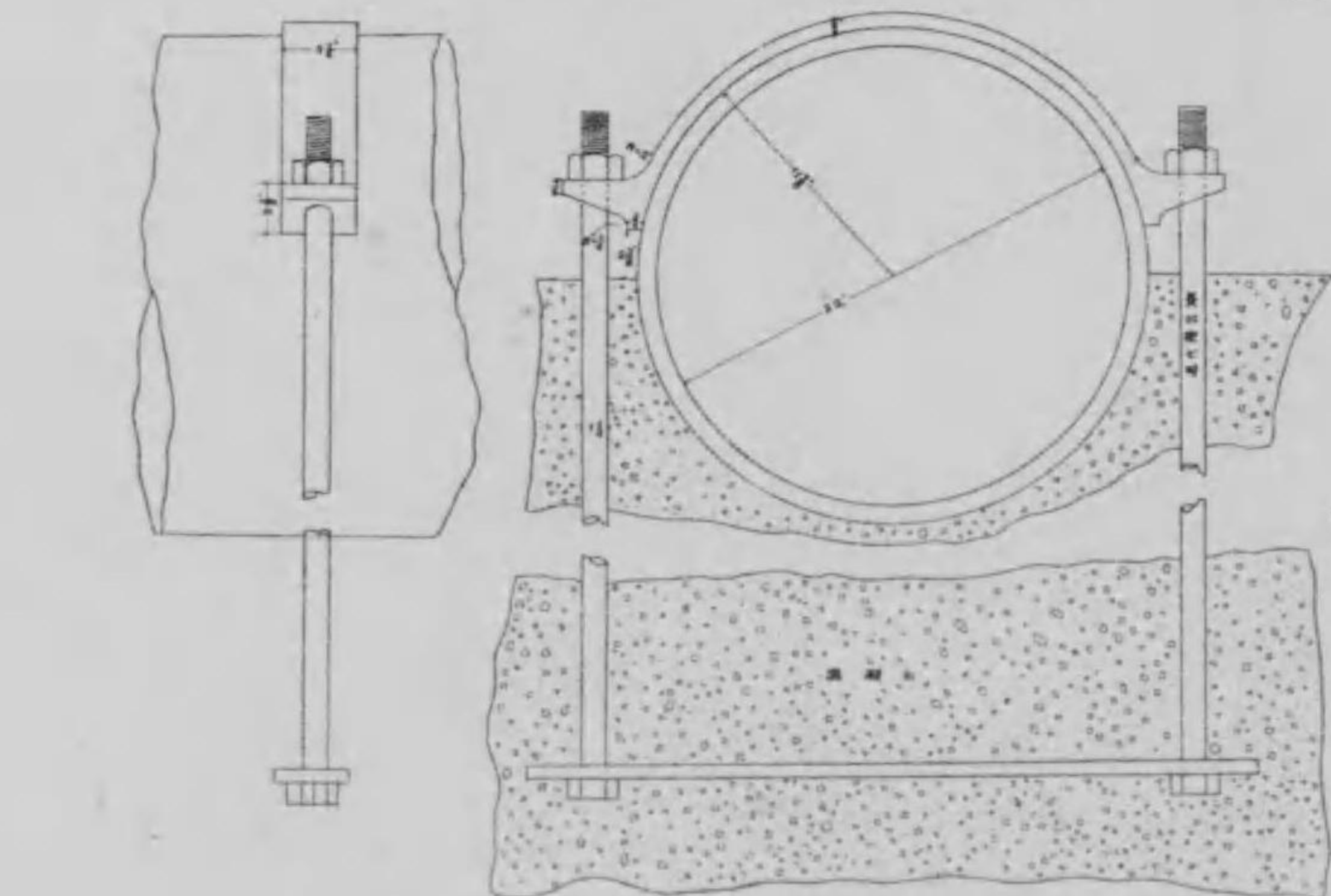
鉛止器之圖
