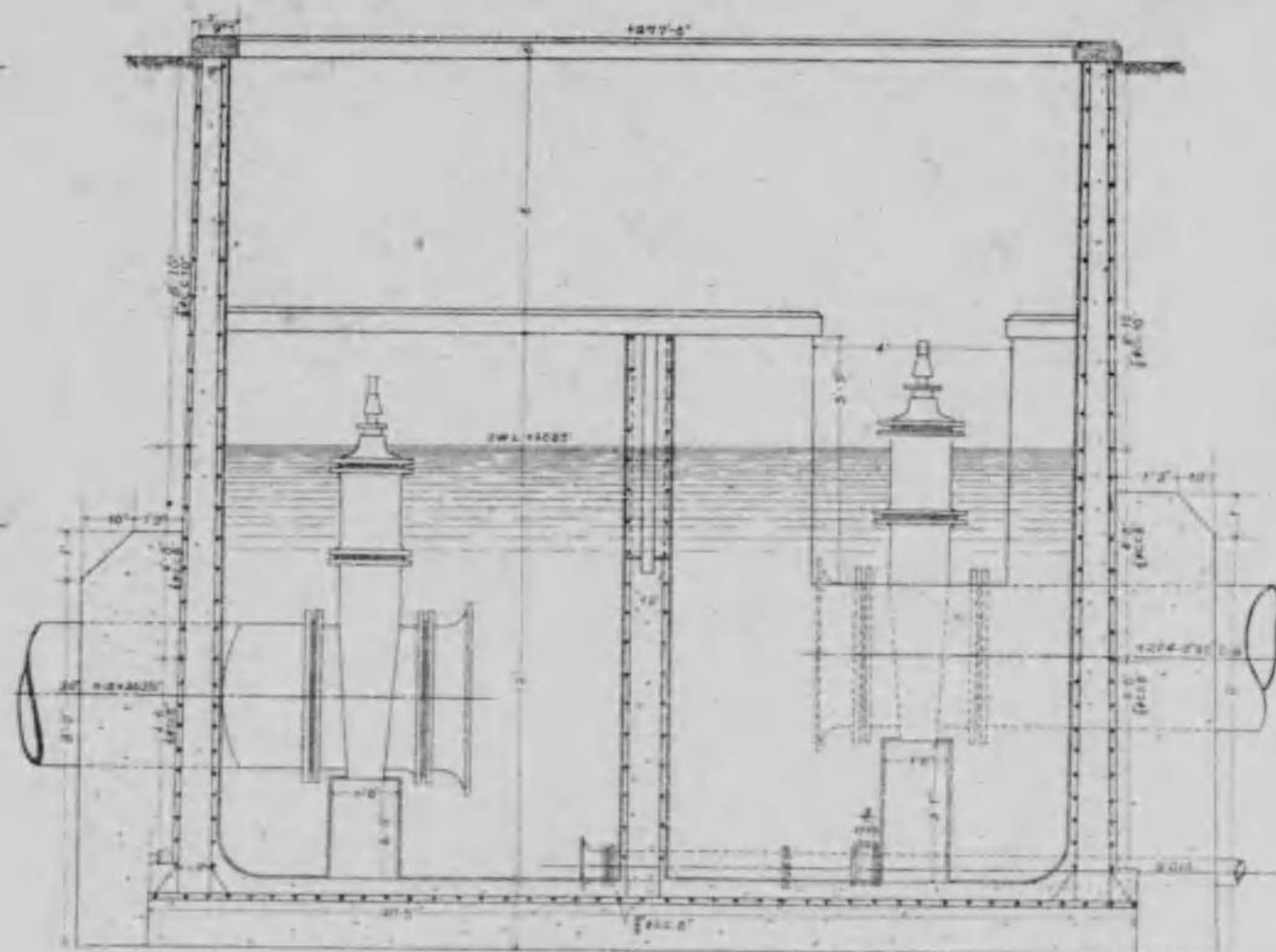
除砂井構造圖
