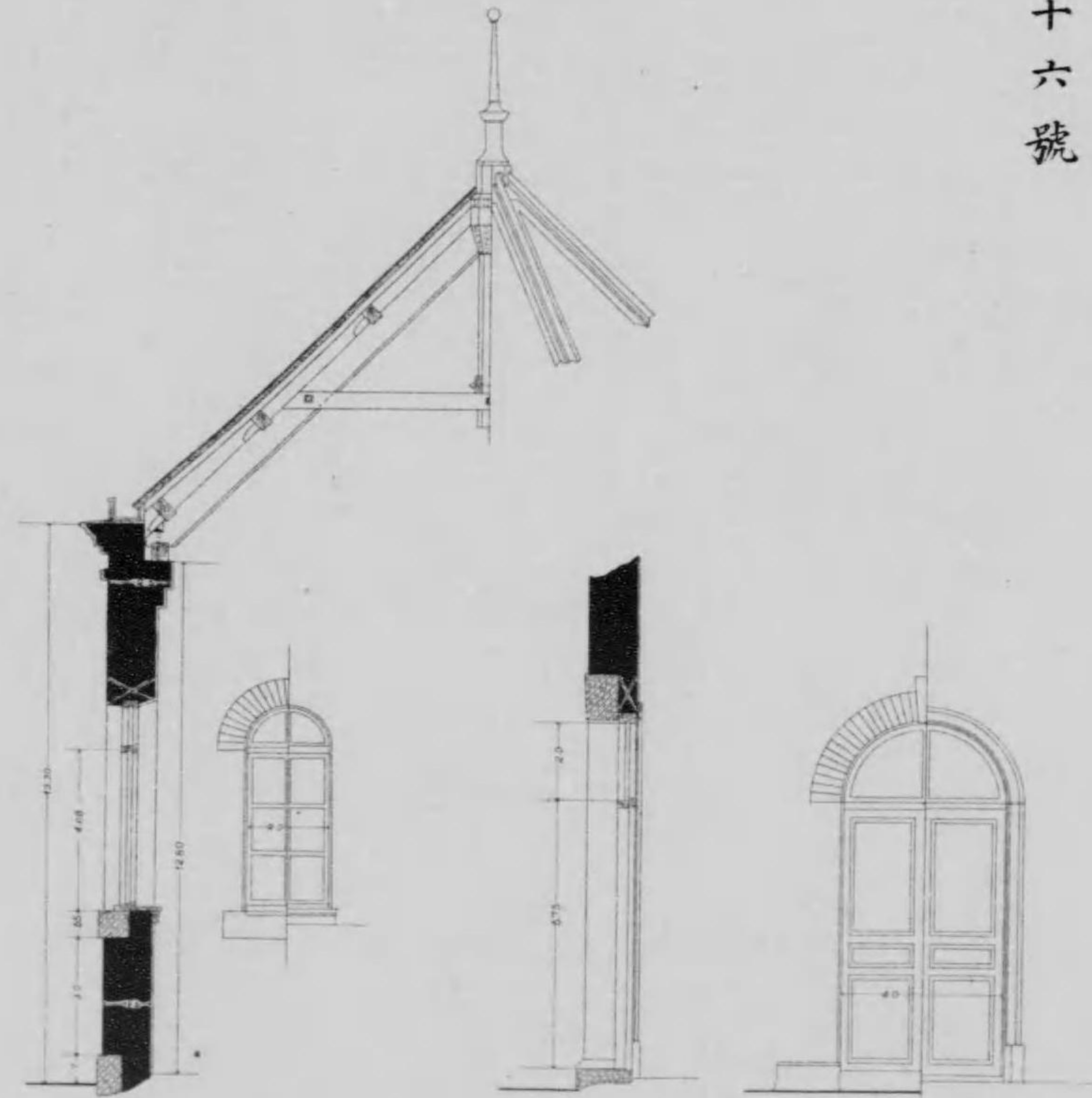
断面圖
