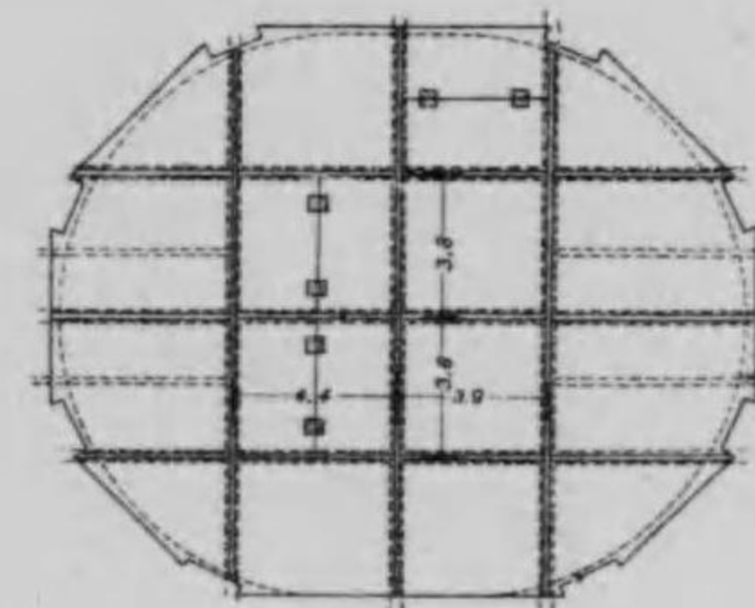
床鉄板平面圖
