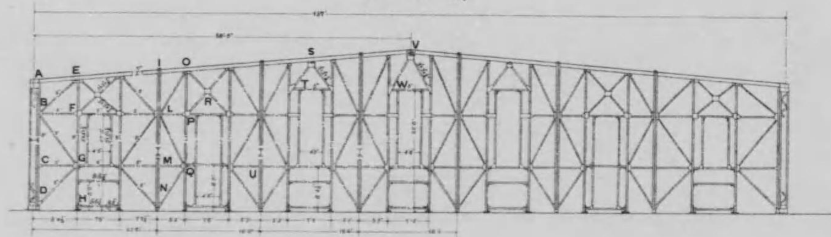
正面圖
