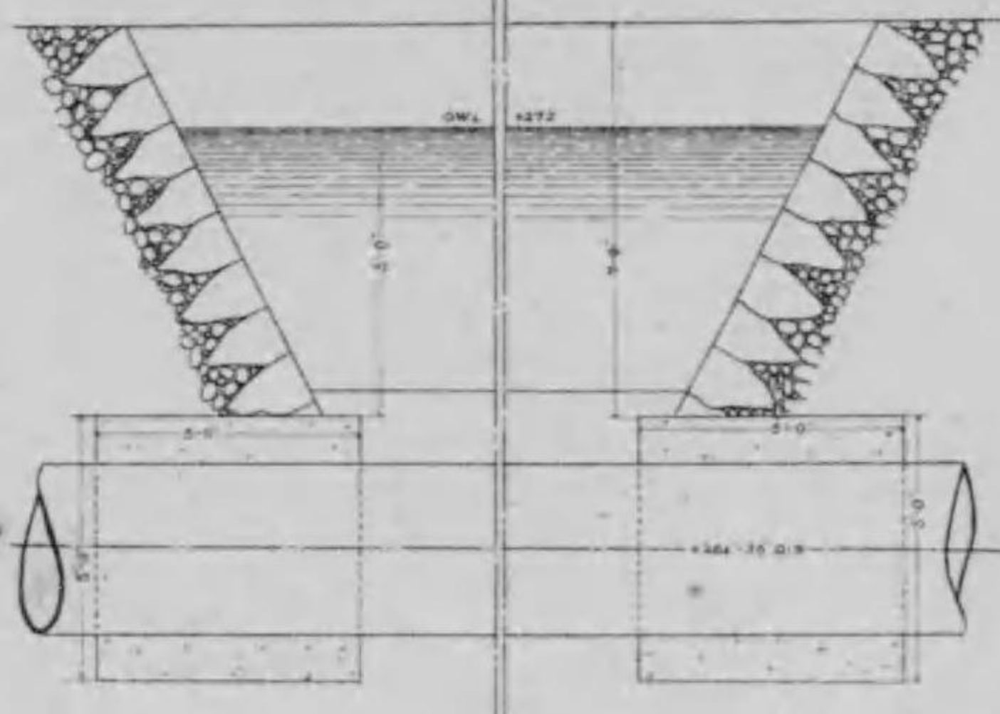
第一疏水運河橫斷圖
