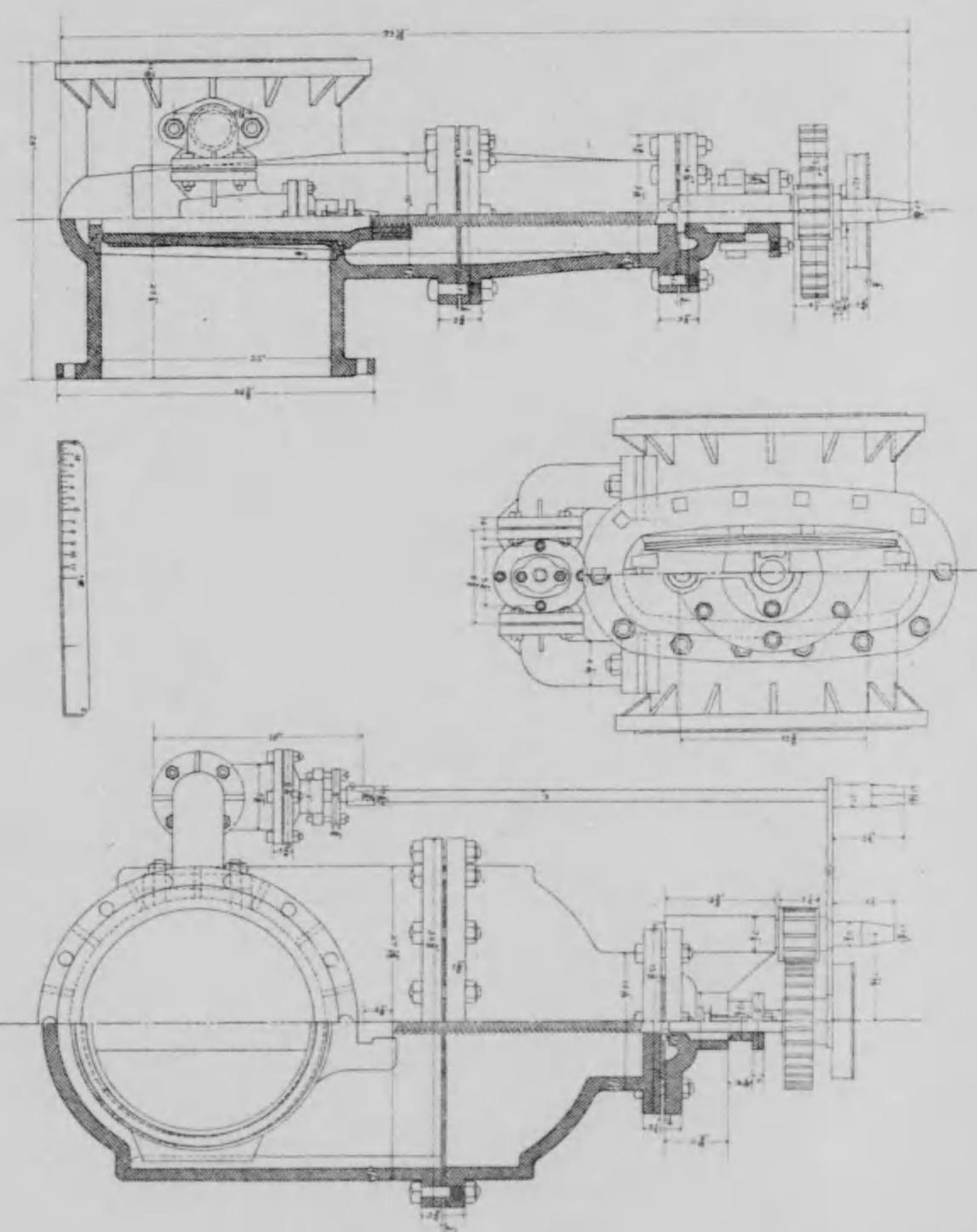
二十吋制水瓣圖
