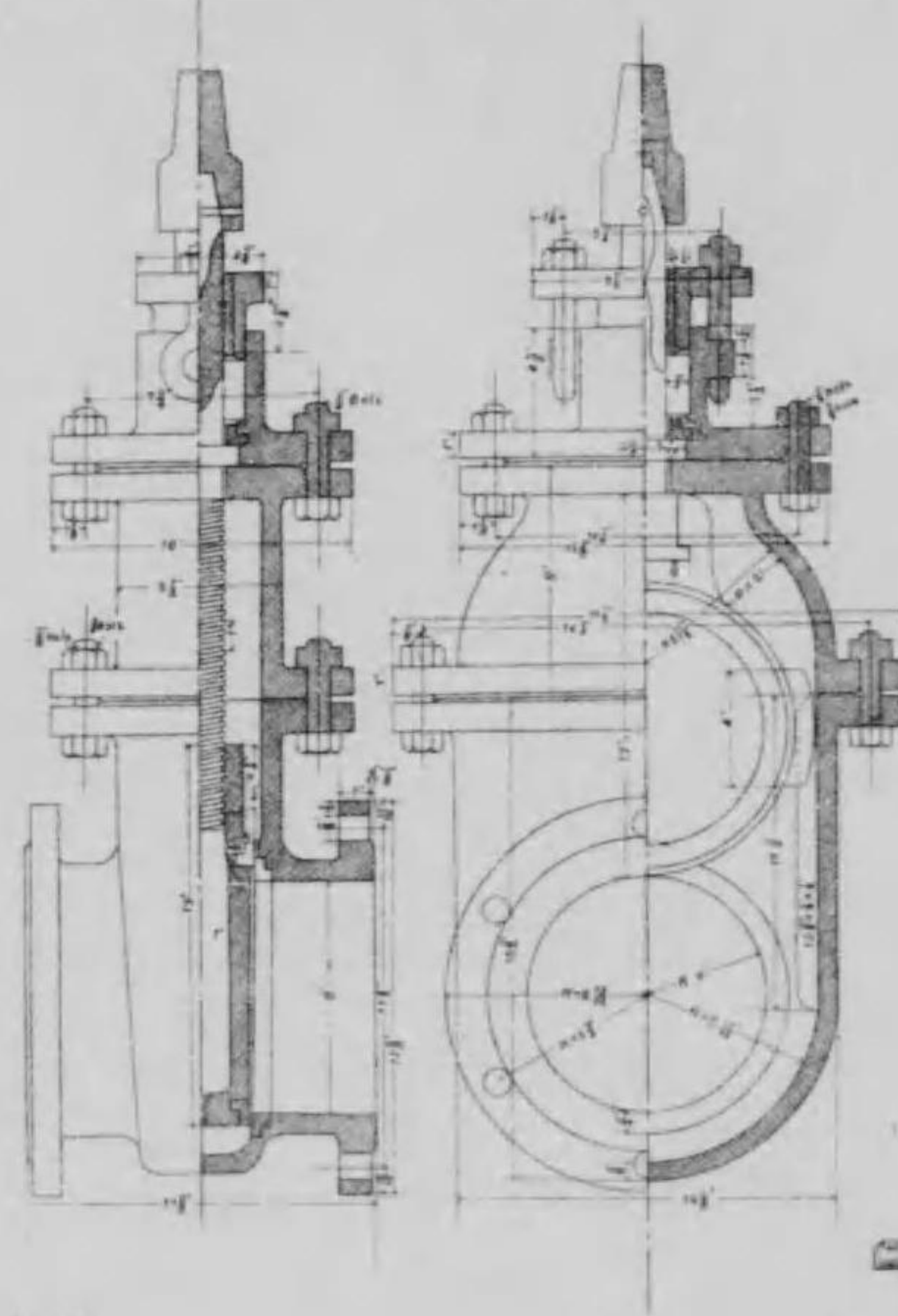
八吋制水瓣圖
