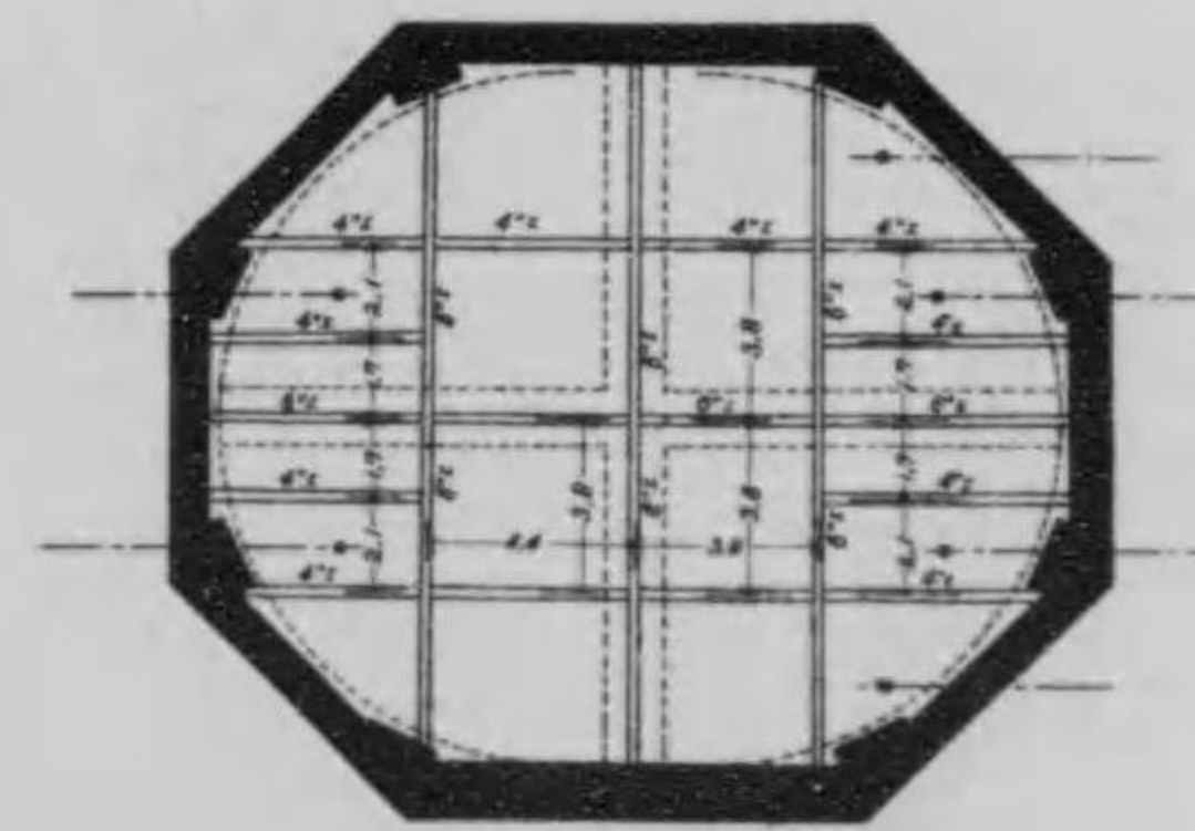
床梁配置圖
