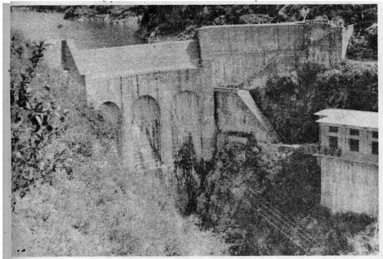
峡门口水库及发电站一角
